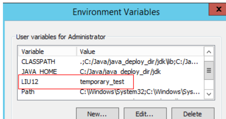
图 3-8 执行结果
