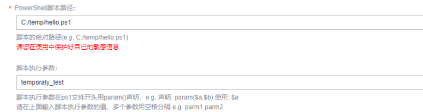
图 3-7 属性设置
