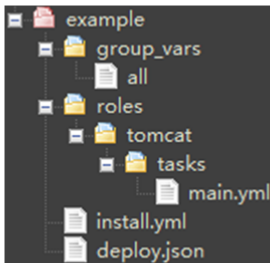
图 3-9 文件架构
