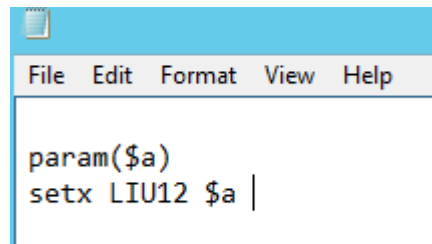
图 3-6 脚本内容
