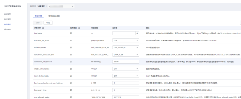
图 9-2 编辑参数模板
