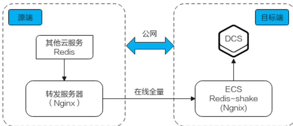
图 11-14 本方案数据流向示意图
