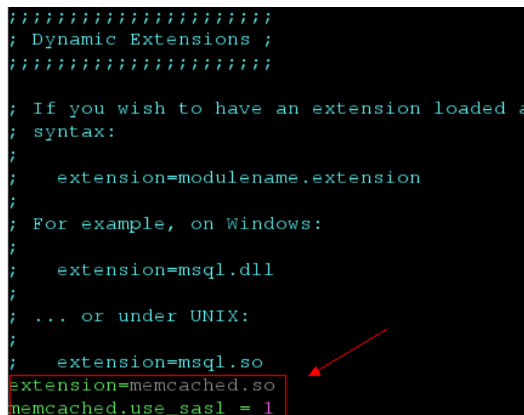
图 5-1 增加 php.ini 配置
