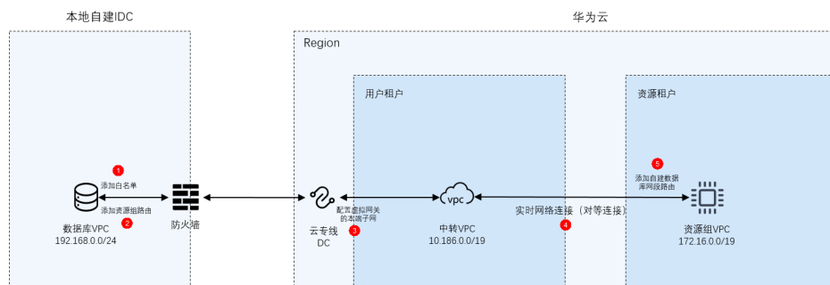
图 7-6 网络示意图
