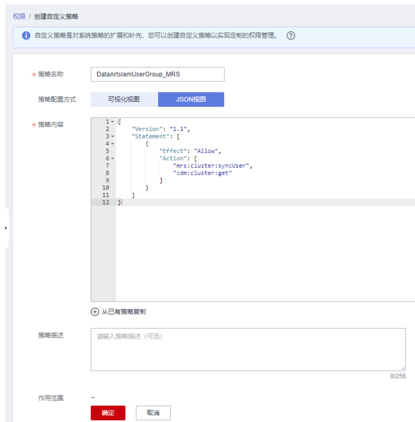
图 9-15 创建 MRS 和 CDM 相关自定义策略
