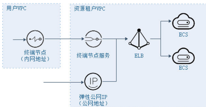
图 14-3 专享版集群网络架构说明
