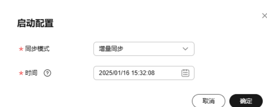
图 7-228 启动配置
