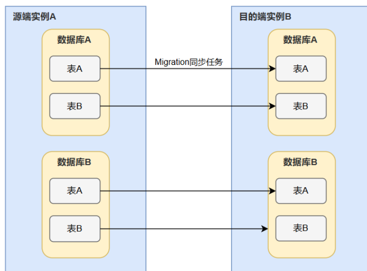
图 7-4 整库同步
