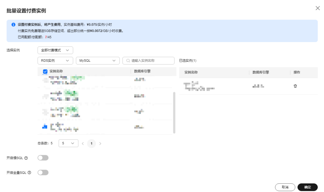
图 4-107 批量设置付费实例窗口
