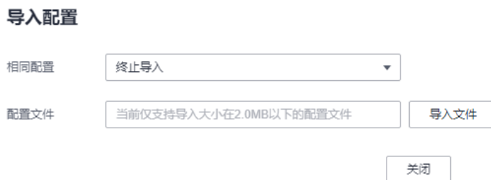
图 4-1 导入配置
