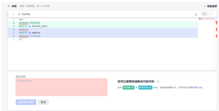
图 18-5 在线手动解决冲突内容页面
