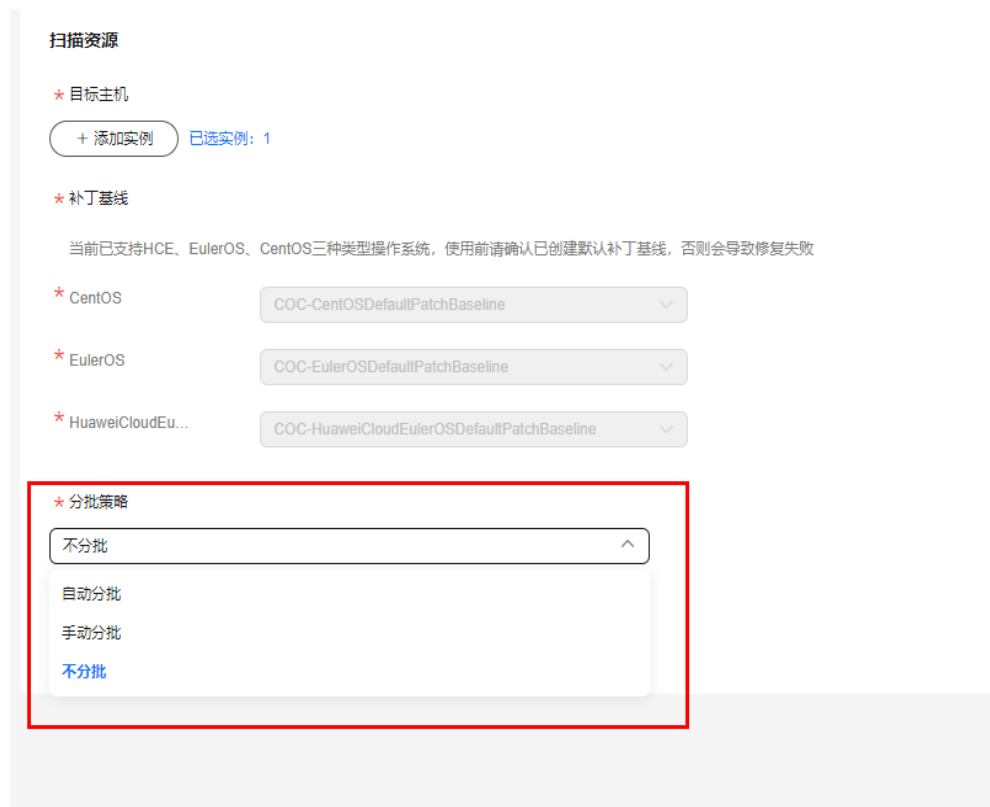
图 4-10 选择分批策略
