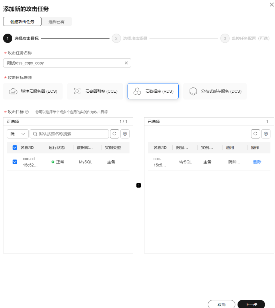
图 8-15 选择攻击目标为云数据库(RDS)
