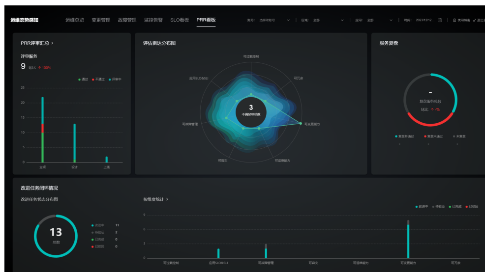
图 2-29 PRR 看板
