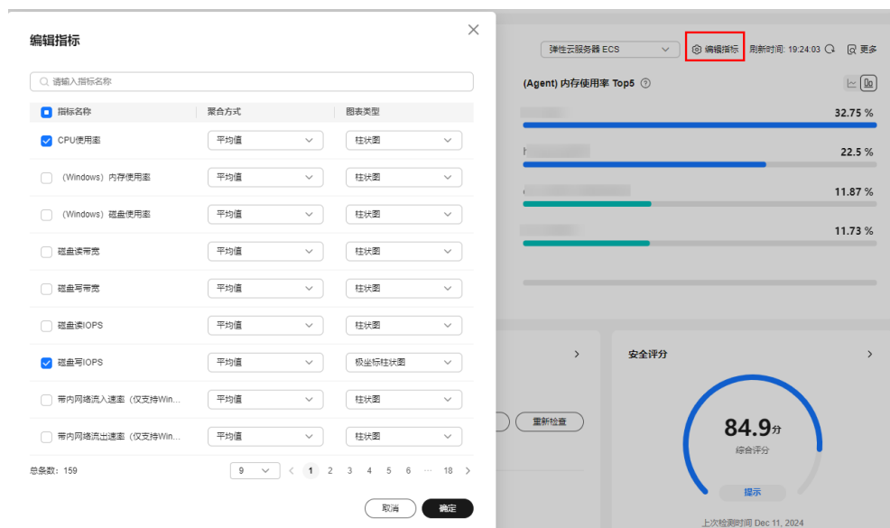
图 2-16 编辑指标
