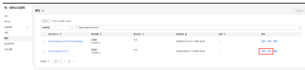
图 1-2 委托列表
