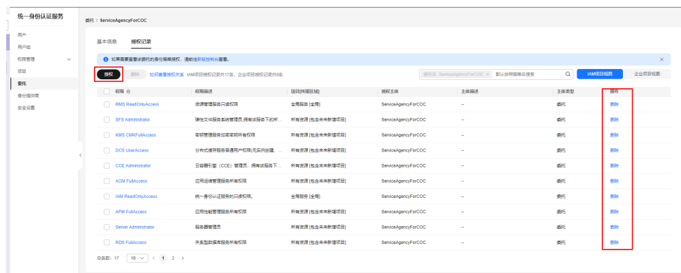
图 1-3 授权记录
