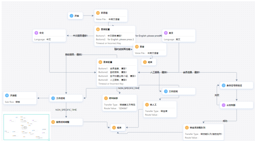
图 2-244 配置实例流程图
