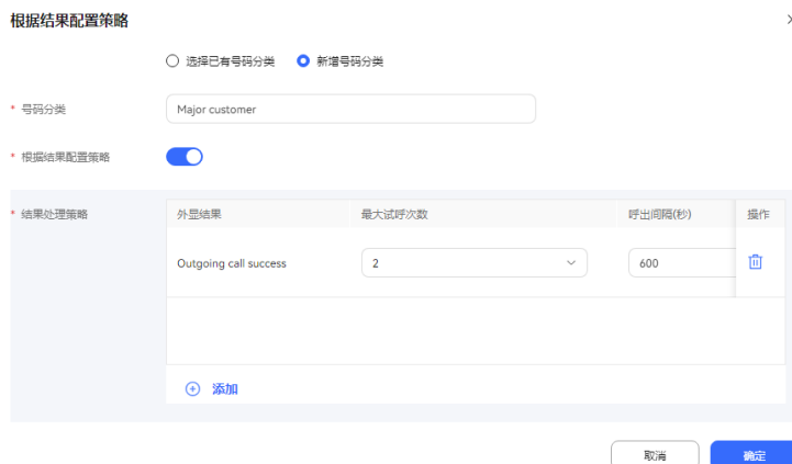
图 2-537 开启根据结果配置策略
