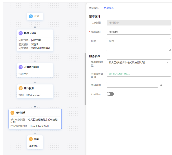
图 2-185 流程编排示例（呼叫转移图元）
