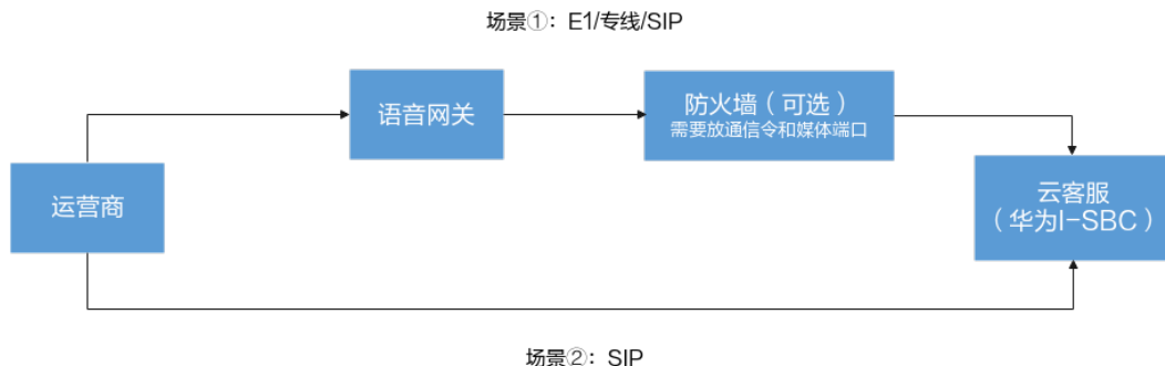
图 1-4 自有 SIP 号码对接
