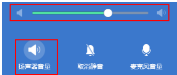
图 3-107 扬声器调节
