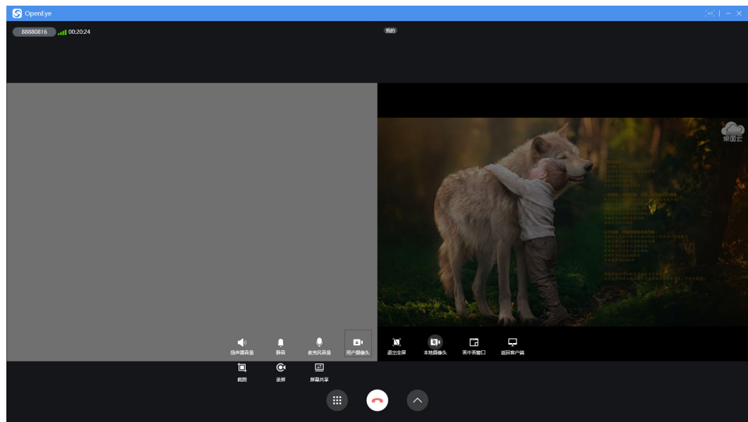
图 3-119 全屏
