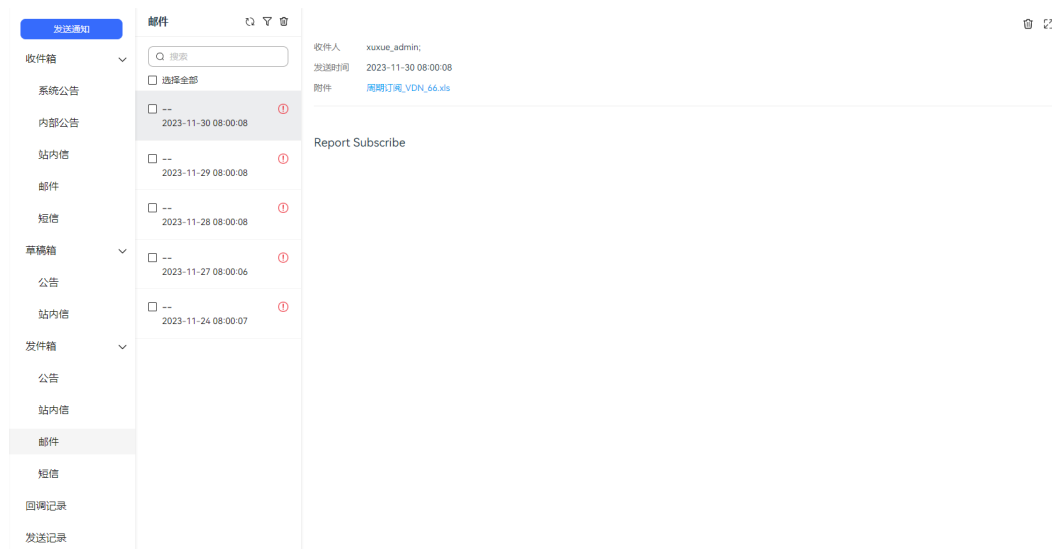
图 2-481 查看通知
