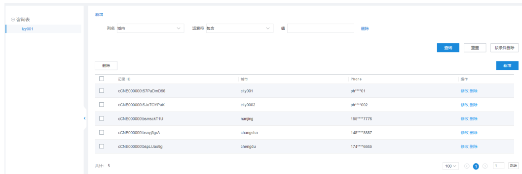
图 2-671 咨询表管理
