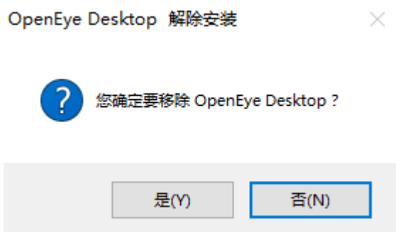
图 3-74 信息确认
