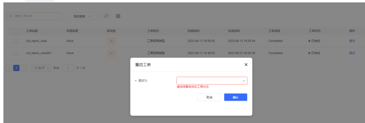
图 2-402 重启工单
