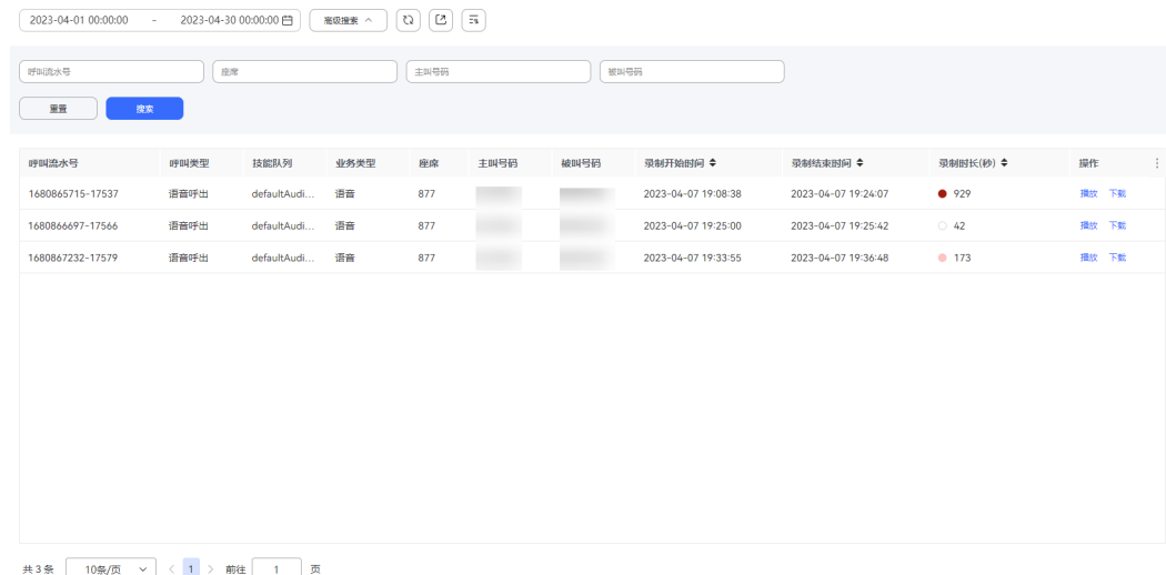
图 4-42 录音回放
