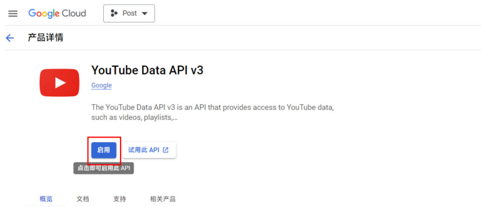
图 2-692 启用 API
