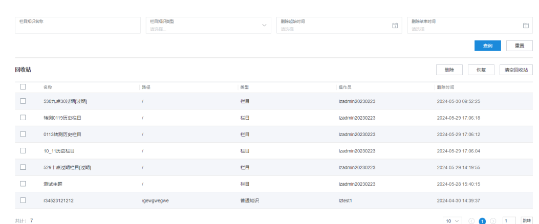
图 2-653 回收站
