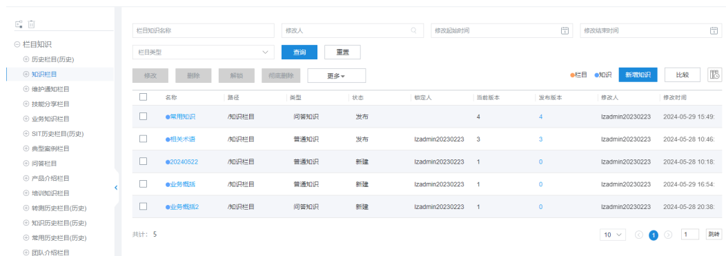
图 2-639 知识列表
