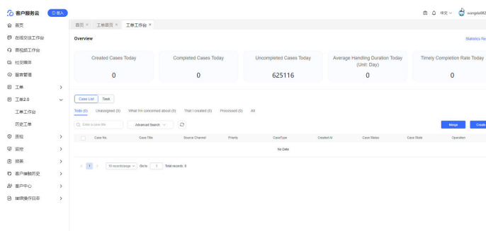
图 2-403 工单工作台
