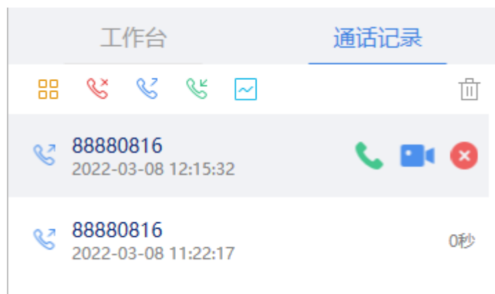
图 3-133 发起呼叫
