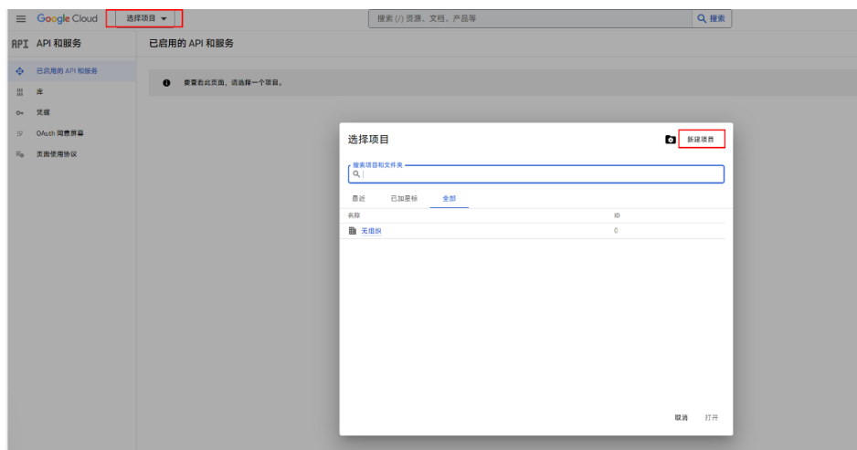
图 2-687 选择项目
