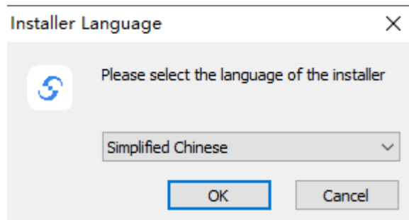
图 3-60 安装语言
