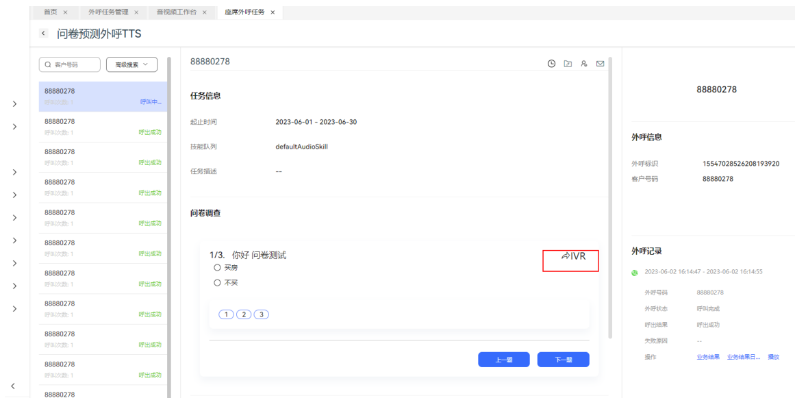
图 3-53 外呼执行
