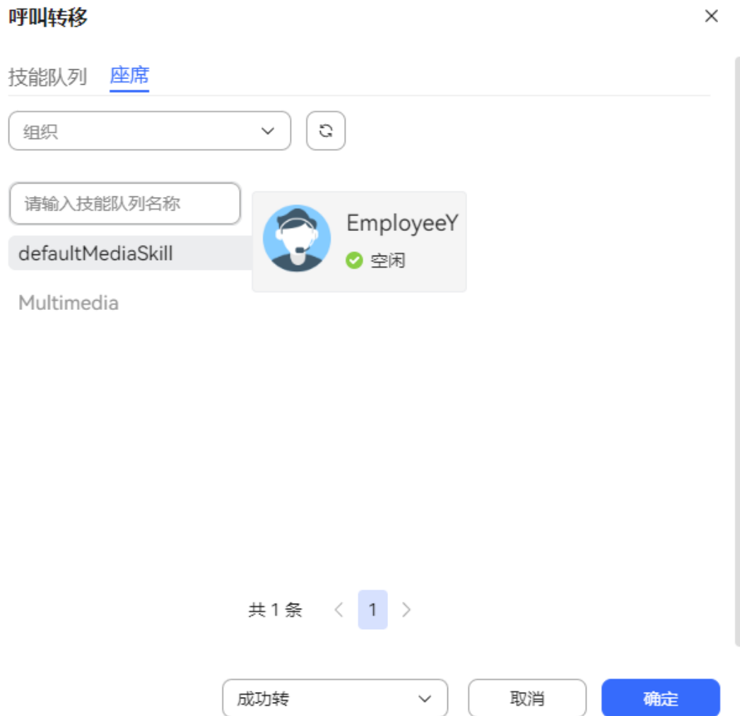
图 3-13 转座席界面
