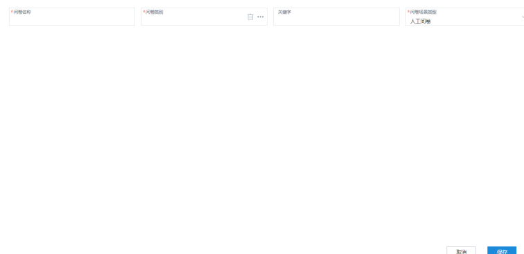
图 2-619 新增问卷
