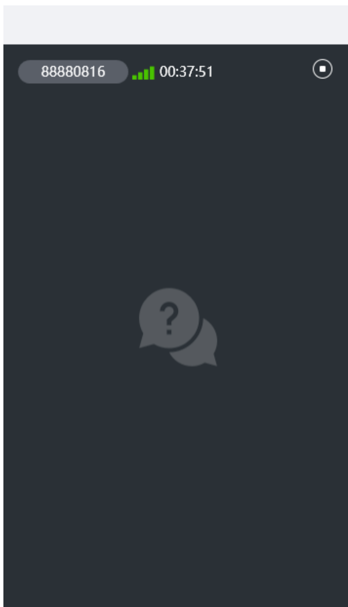
图 3-121 录屏
