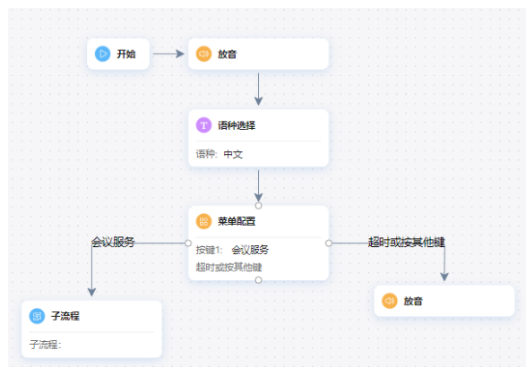
图 2-239 编辑流程
