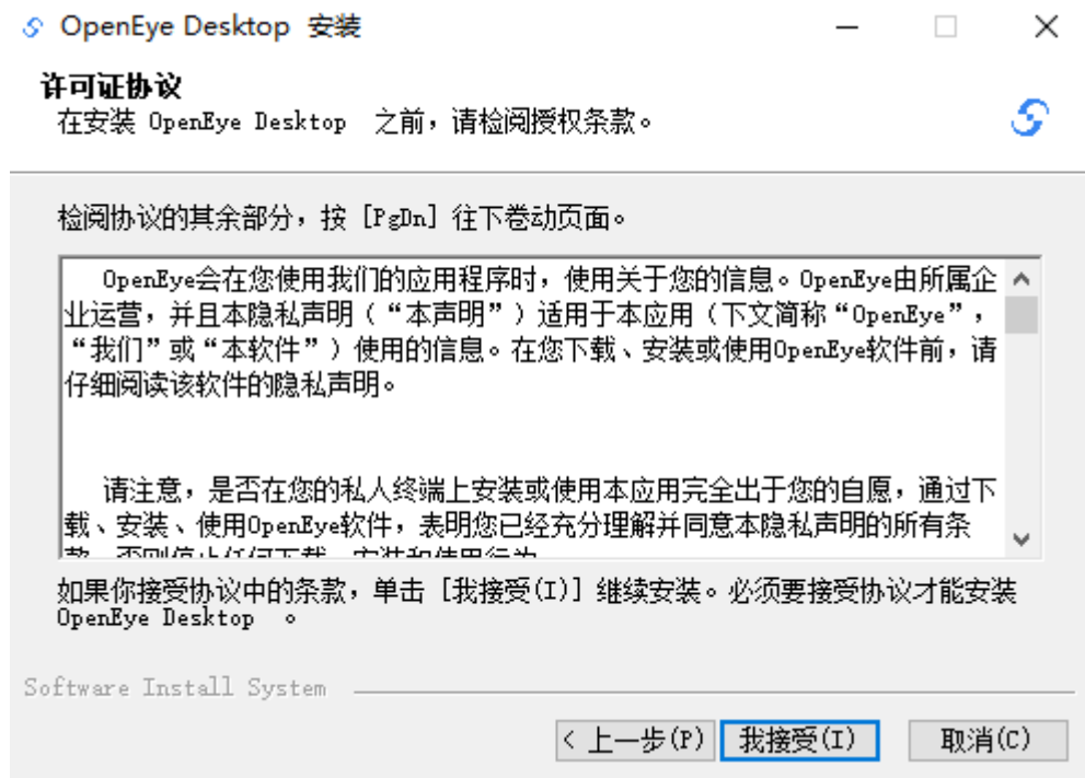
图 3-62 许可协议
