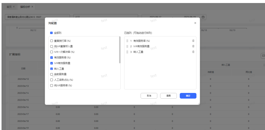
图 2-337 列配置
