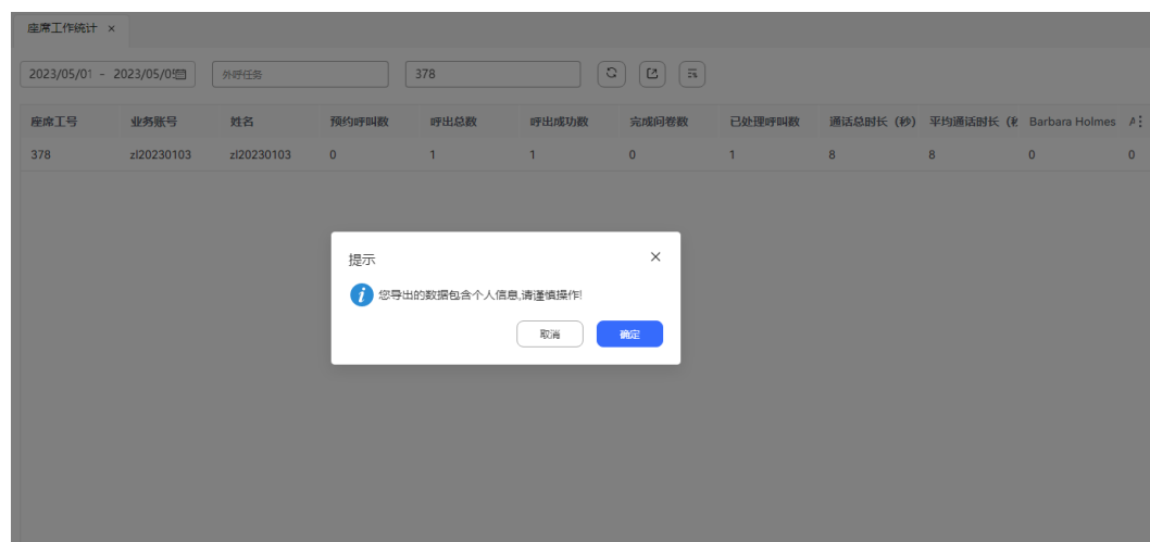
图 2-609 导出数据包
