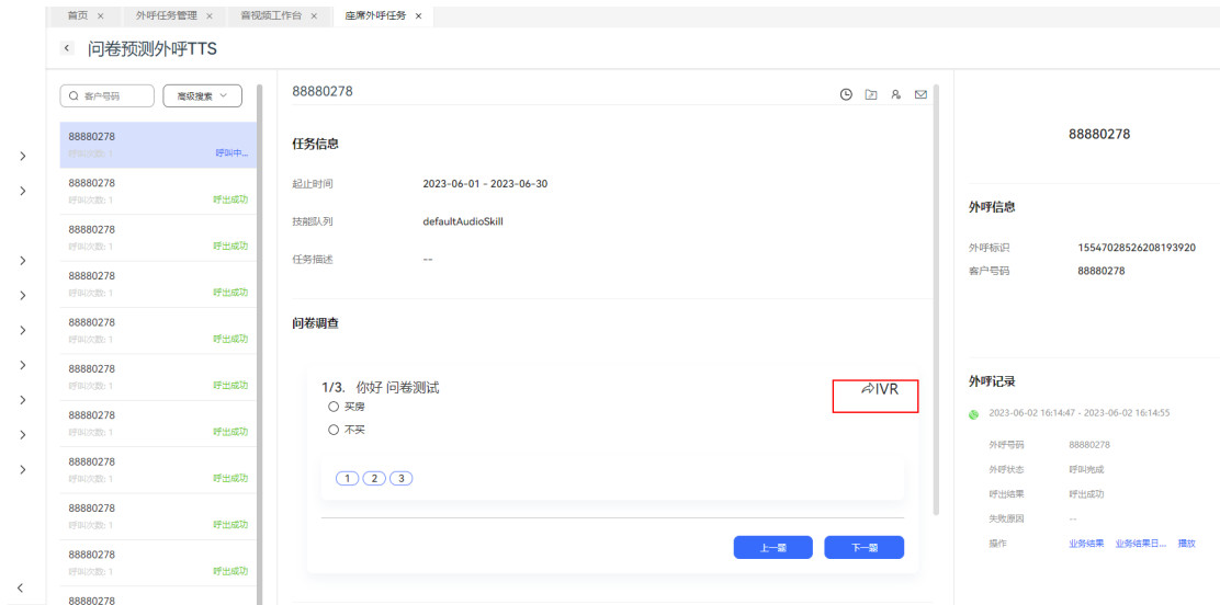
图 3-55 外呼执行
