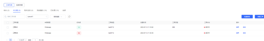
图 2-383 接受工单
