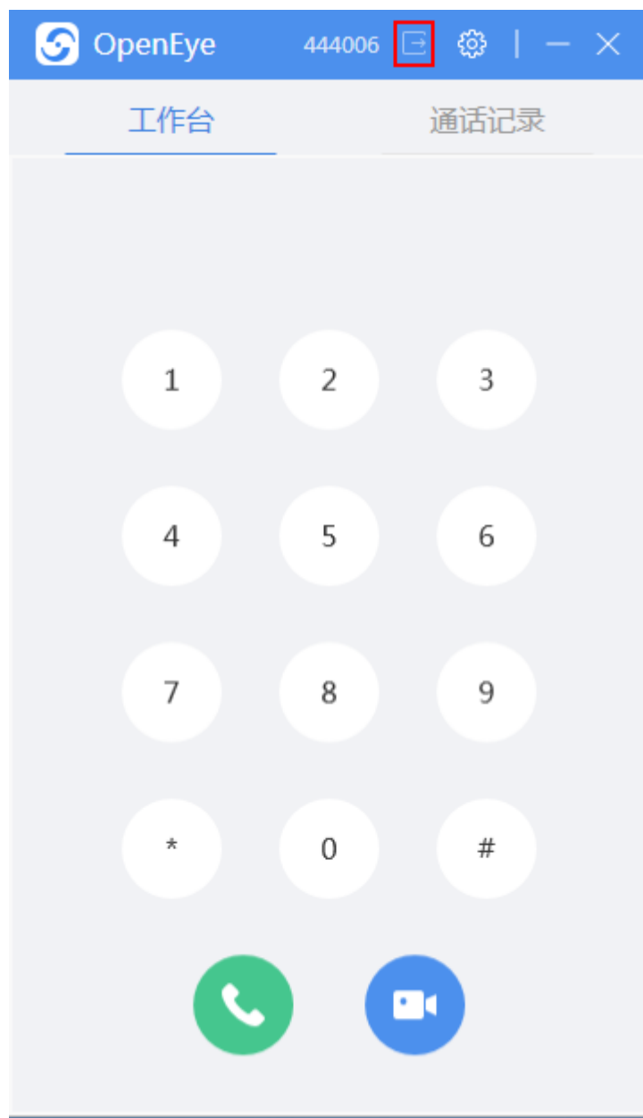
图 3-86 登出界面
