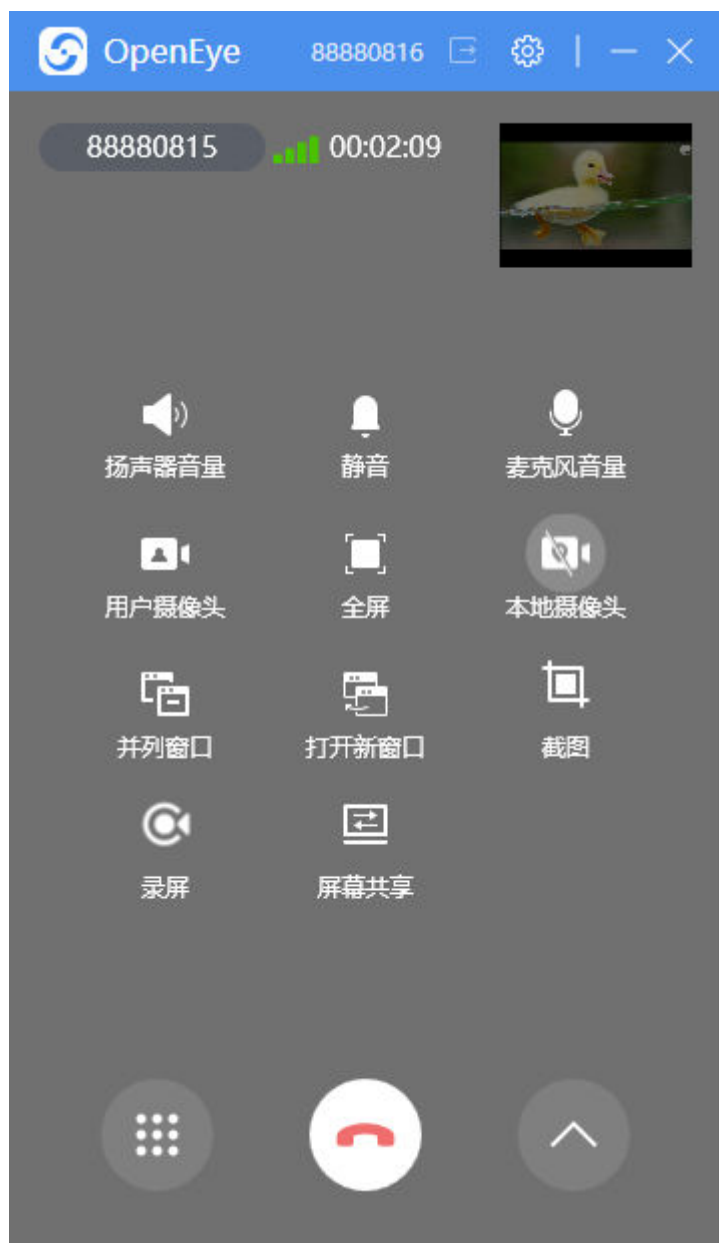
图 3-115 功能区
