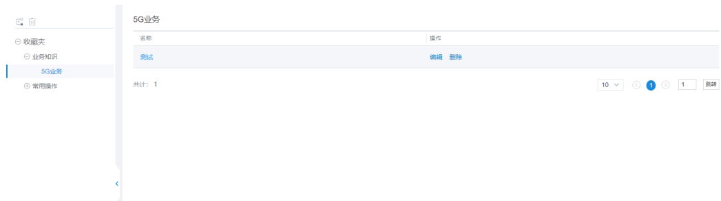
图 2-664 收藏夹
