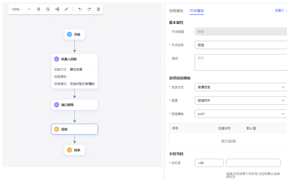
图 2-208 流程编排示例（短信发送图元）
