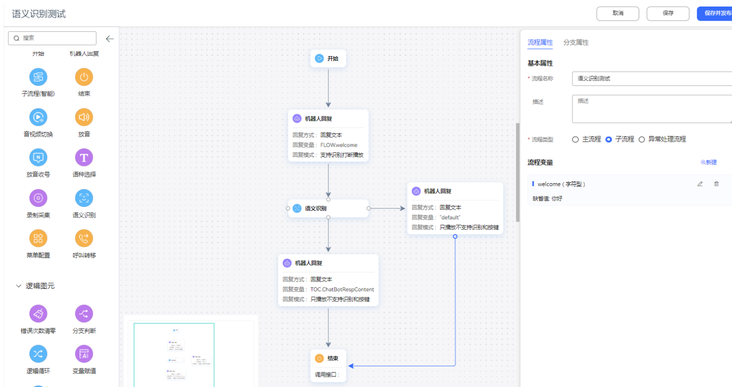
图 2-140 流程编排示例
