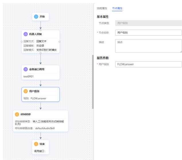
图 2-184 流程编排示例（用户级别图元）
