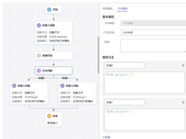
图 2-199 流程编排示例（分支判断图元）
