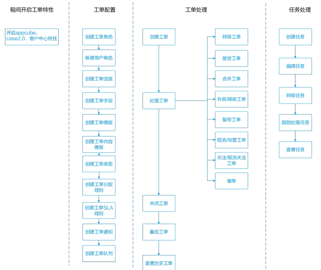
图 2-345 工单功能概览
