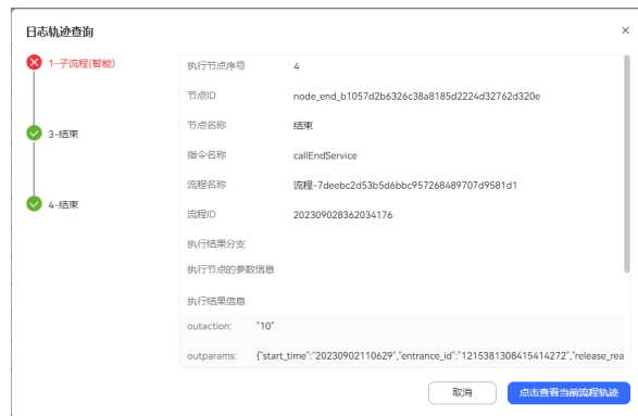
图 2-248 流程轨迹日志界面
