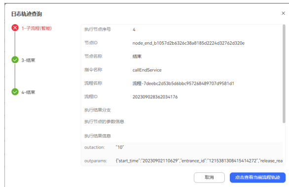
图 2-134 流程轨迹日志界面
