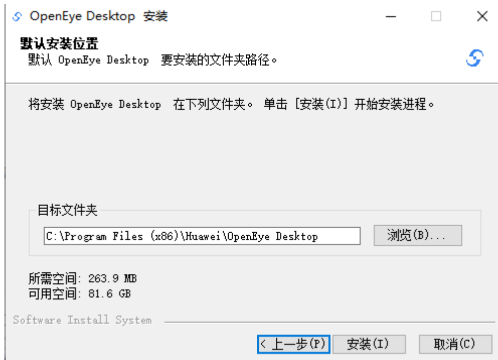
图 3-63 安装位置
