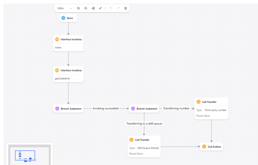
图 2-74 绘制流程
