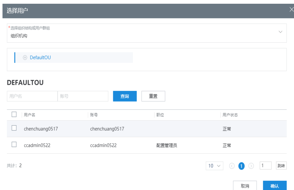
图 2-418 选择用户
