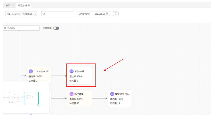
图 2-323 复合图元
