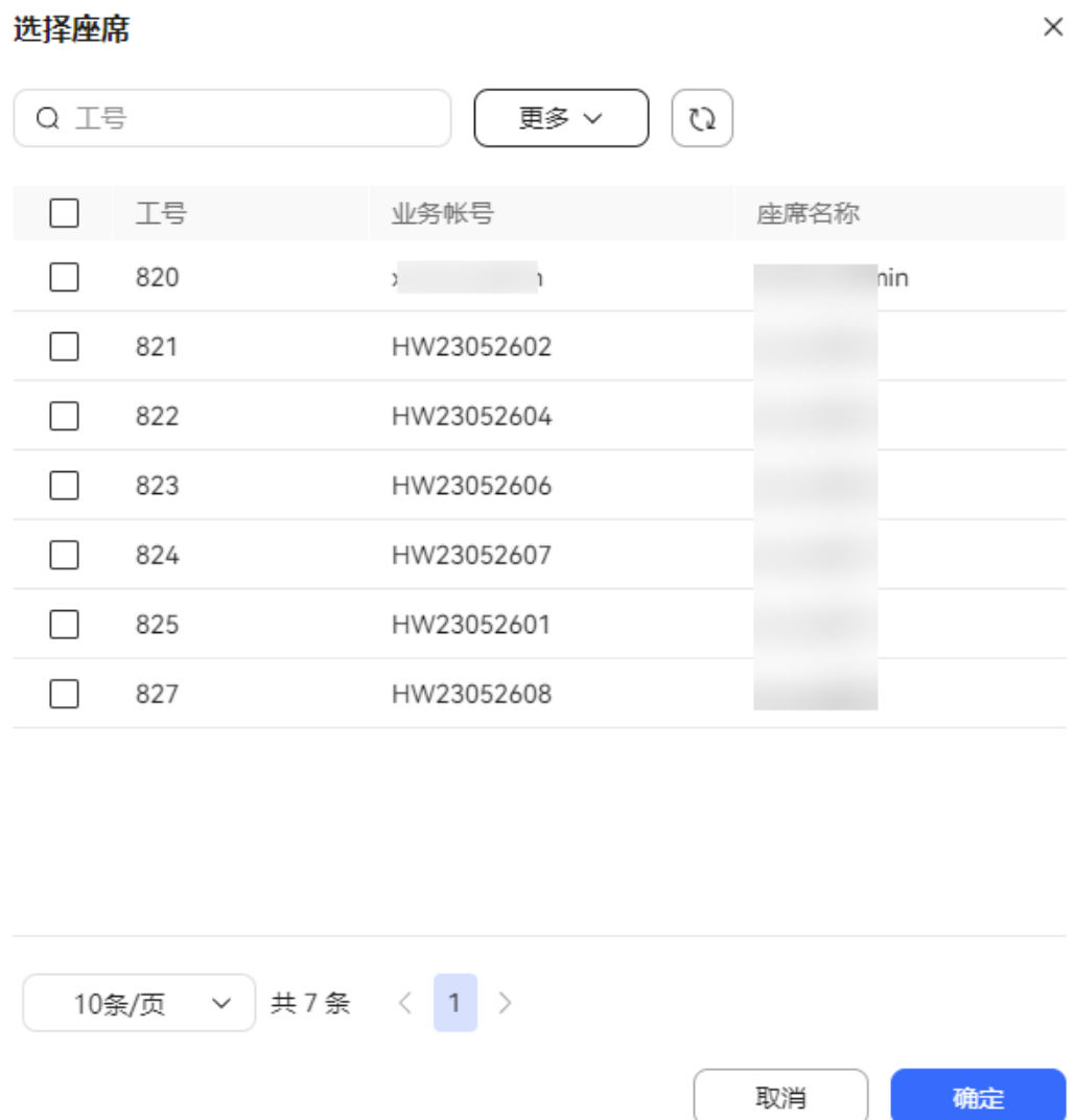
图 4-33 选择座席
