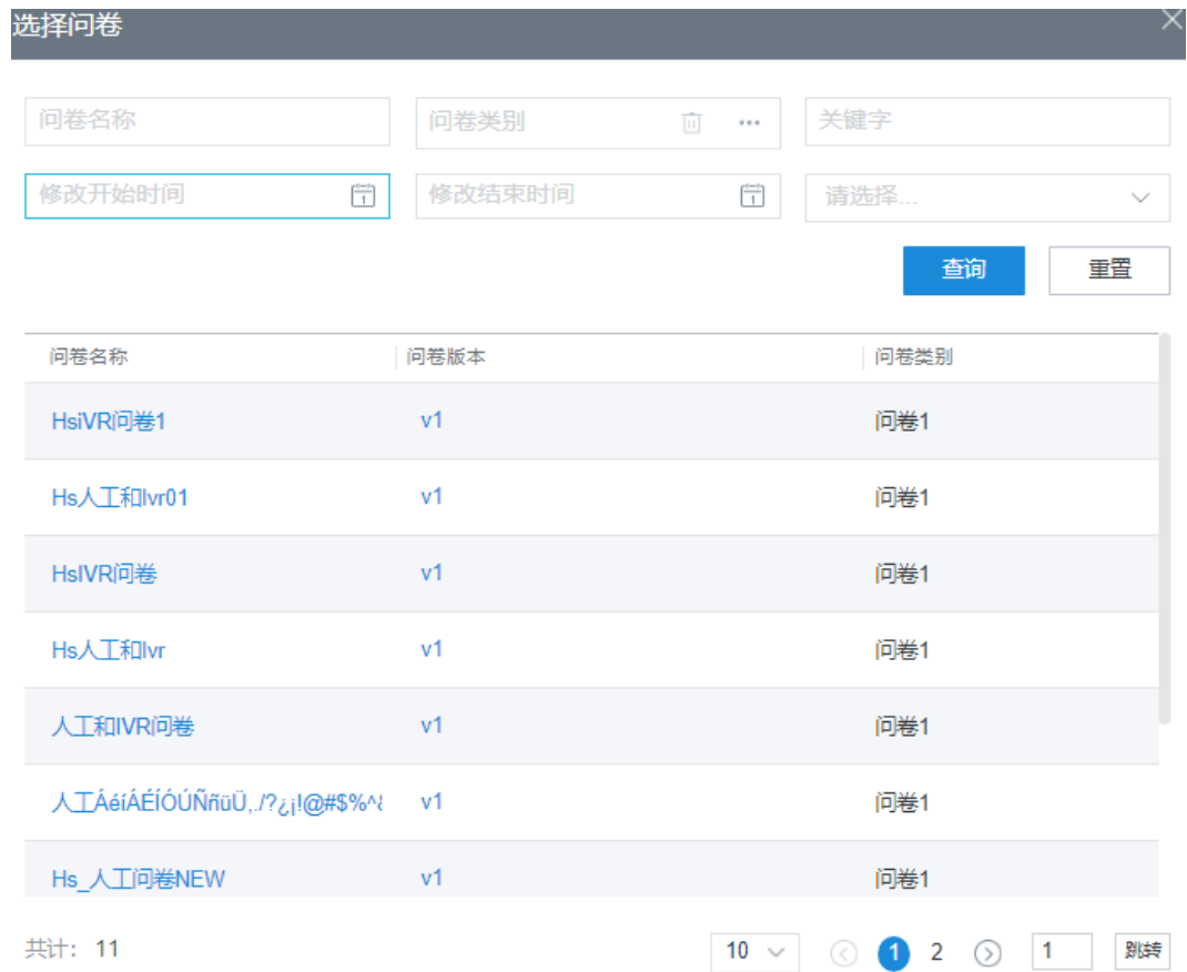
图 2-627 选择问卷
