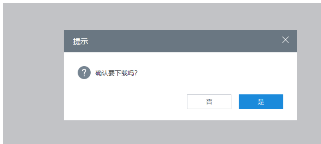
图 2-434 导出确认
