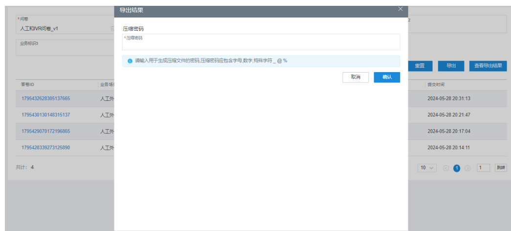
图 2-628 导出问卷
