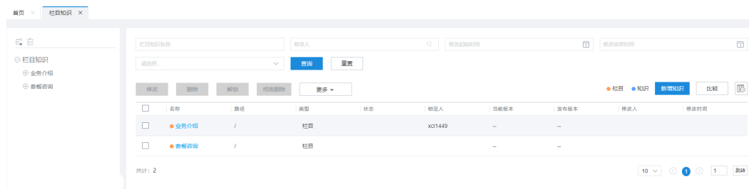
图 2-637 栏目知识
