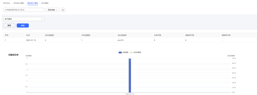
图 2-120 按天查询
