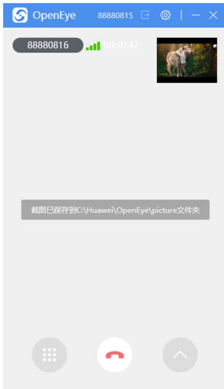
图 3-120 截图
