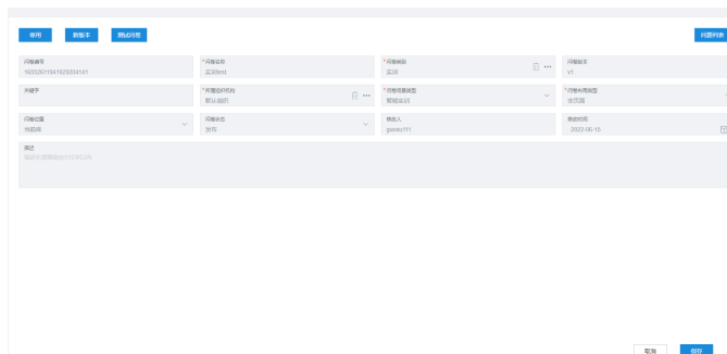
图 2-635 关联问卷
