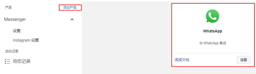
图 2-79 添加产品
