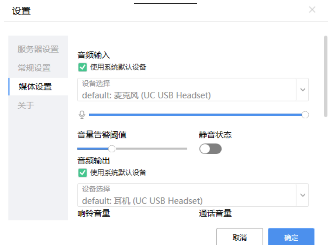
图 3-96 媒体设置 1
