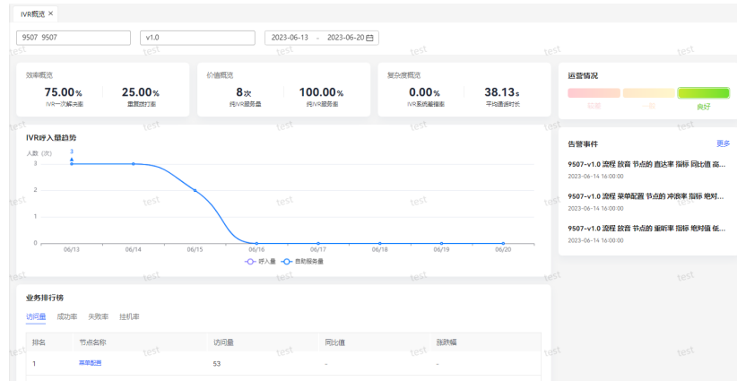
图 2-317 IVR 概览
