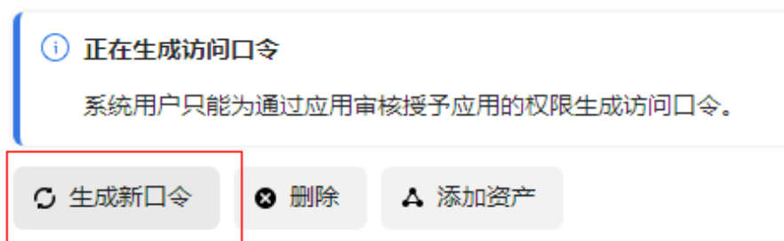
图 2-83 生成新口令
