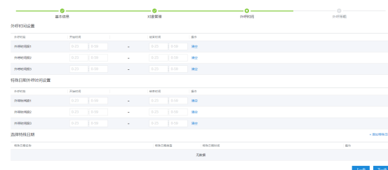
图 2-632 外呼时间
