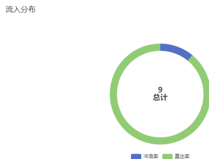
图 2-325 流入分布
