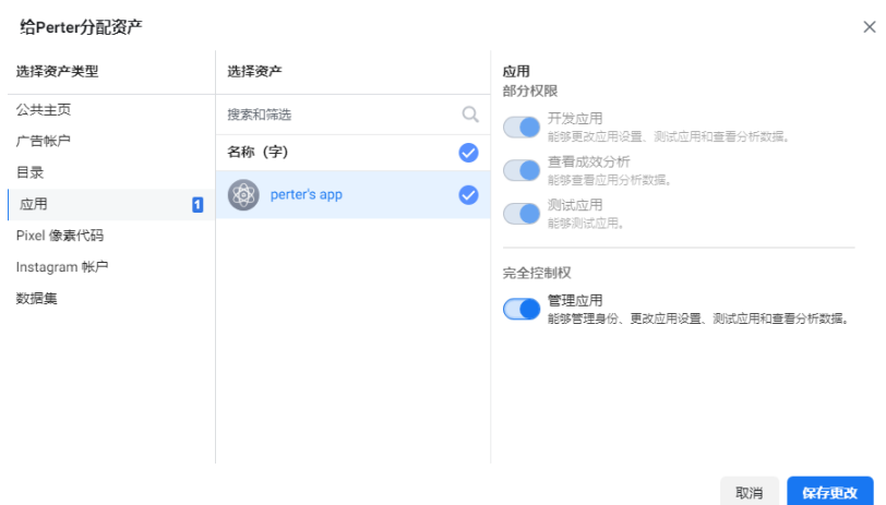
图 2-82 添加资产
