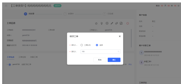
图 2-365 转派工单
