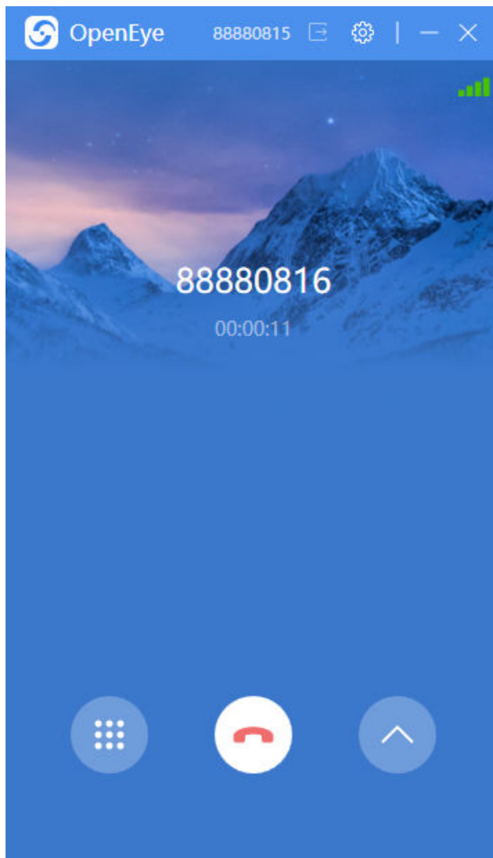
图 3-103 通话界面
