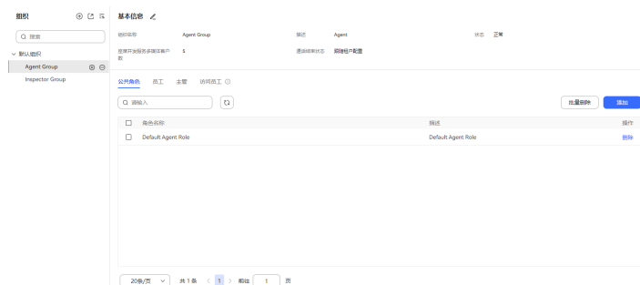
图 2-6 组织机构
