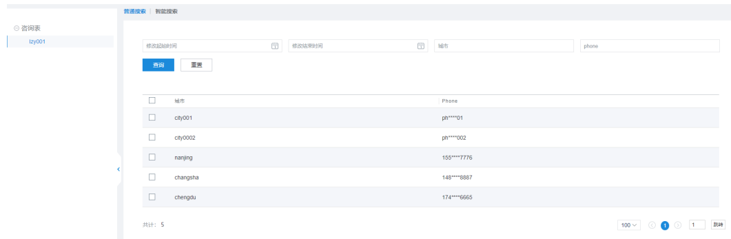
图 2-673 搜索咨询表
