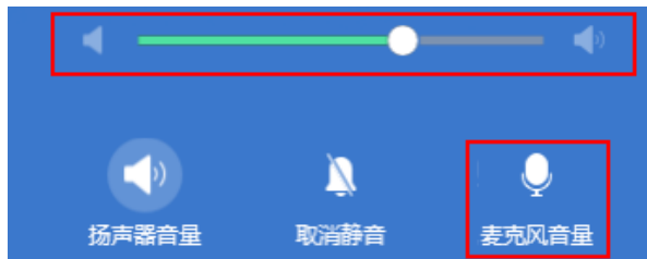
图 3-106 麦克风调节
