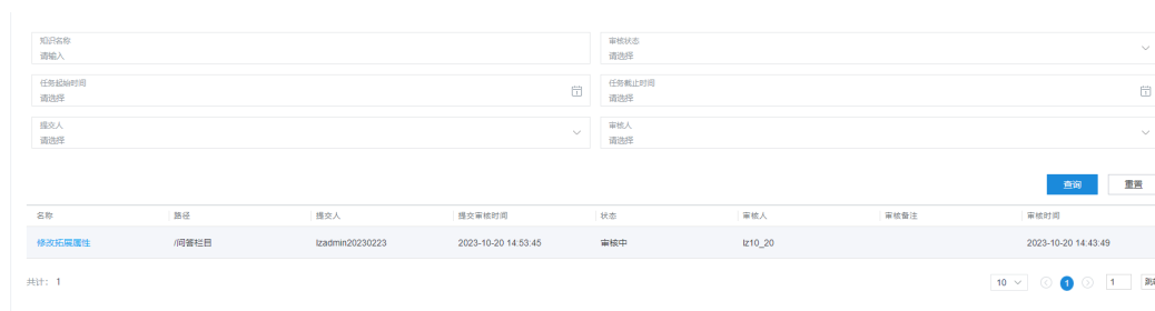
图 2-651 审核记录
