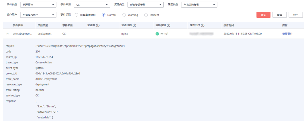
图 12-1 展开记录
