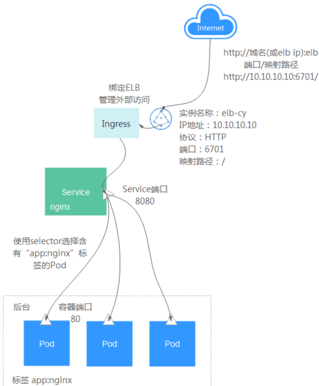
图 5-5 公网访问
