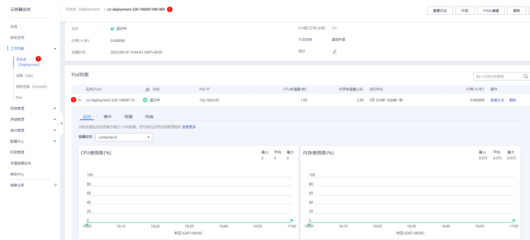
图 10-1 Pod 列表
