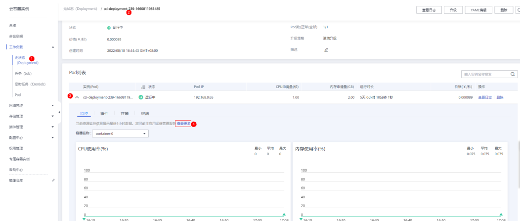
图 10-2 Pod 监控
