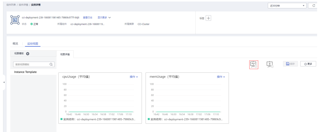
图 10-3 视图模板
