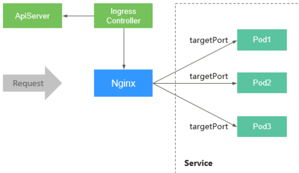
图 4-81 Nginx Ingress 工作原理
