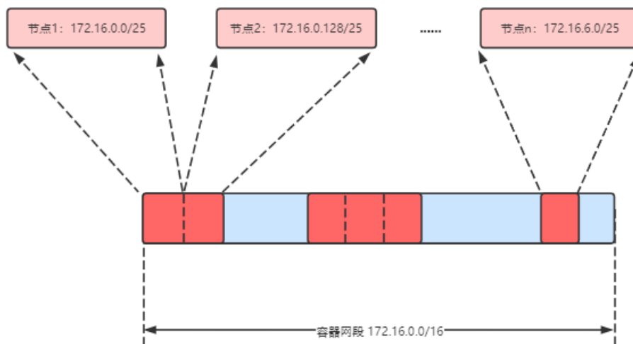
图 3-137 VPC 网络 IP 地址管理
