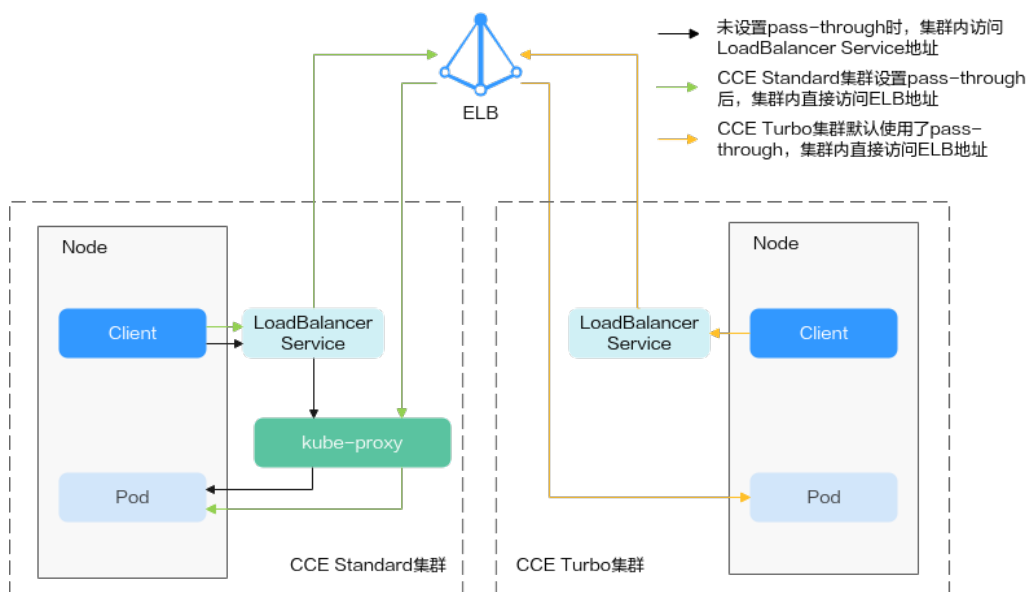
图 3-163 pass-through 访问示例
