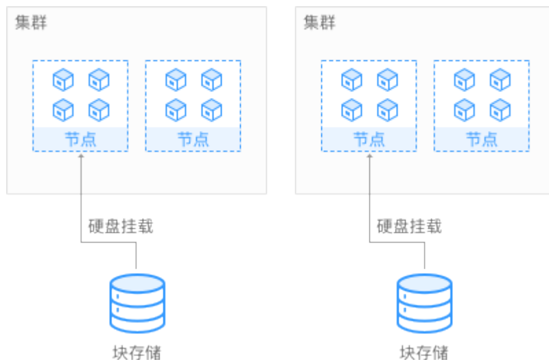
图 3-424 CCE 挂载云硬盘存储卷
