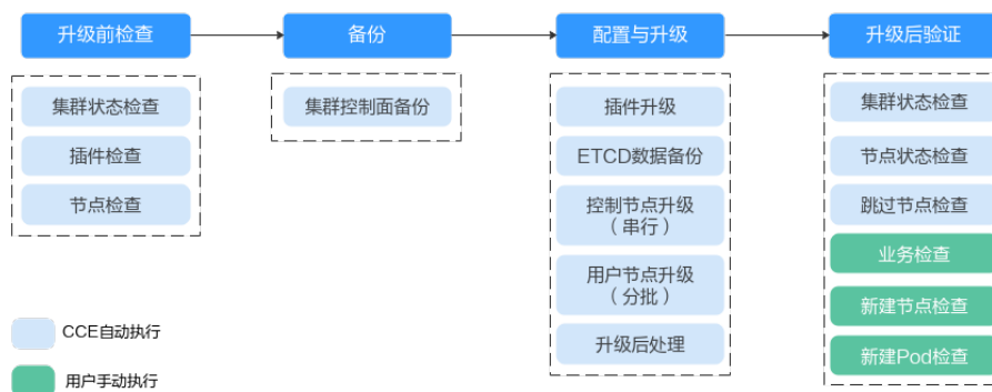
图 3-11 集群升级流程
