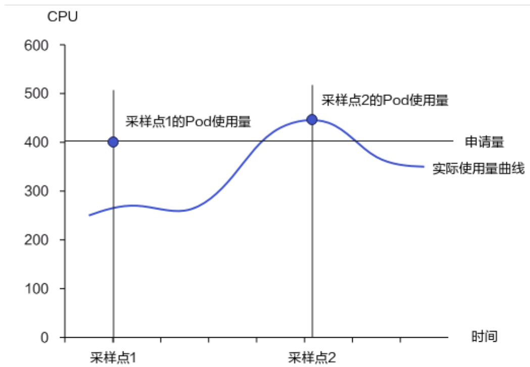
图 3-351 工作负载成本计算原理
