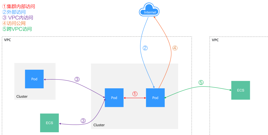
图 3-132 网络访问示意图
