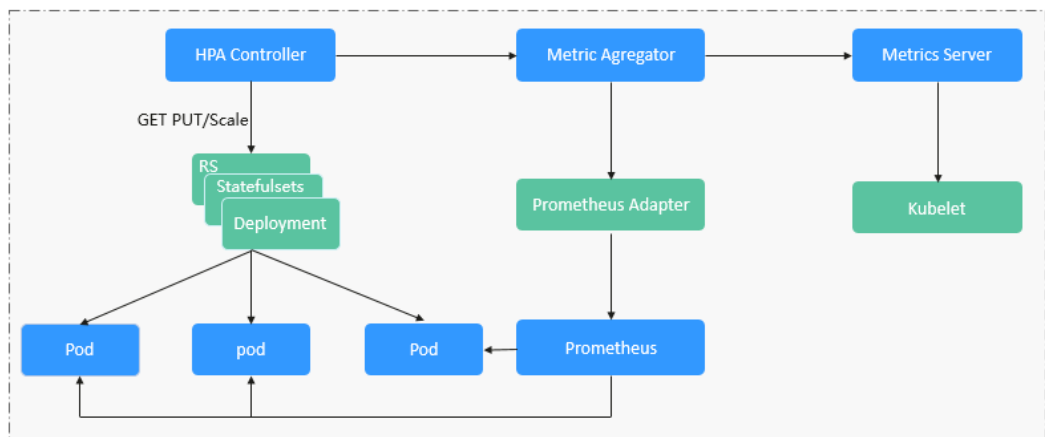
图 4-73 HPA 流程图
