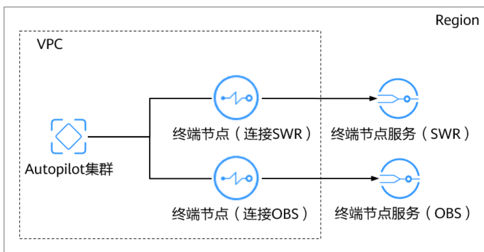
图 4-25 Autopilot 集群访问 SWR 和 OBS
