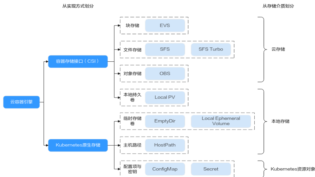
图 3-207 容器存储概览类型
