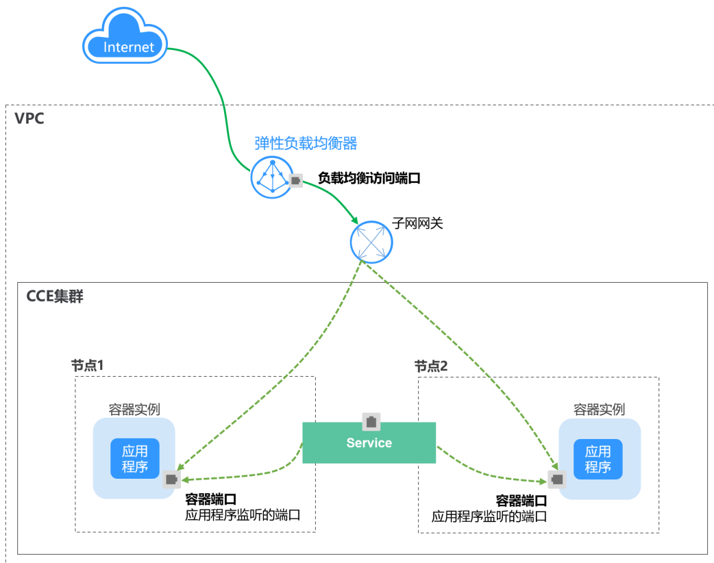
图 3-152 ELB 直通容器
