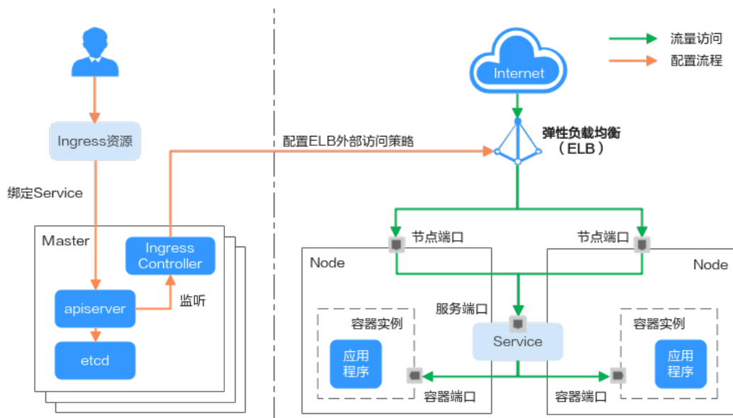
图 3-169 ELB Ingress 工作原理（CCE Standard 集群以及 CCE Turbo 集群使用共享型 ELB 场景）
