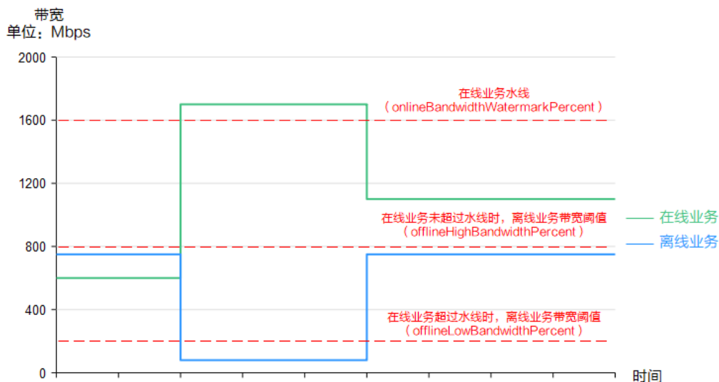
图 3-129 出口网络带宽保障示例图
