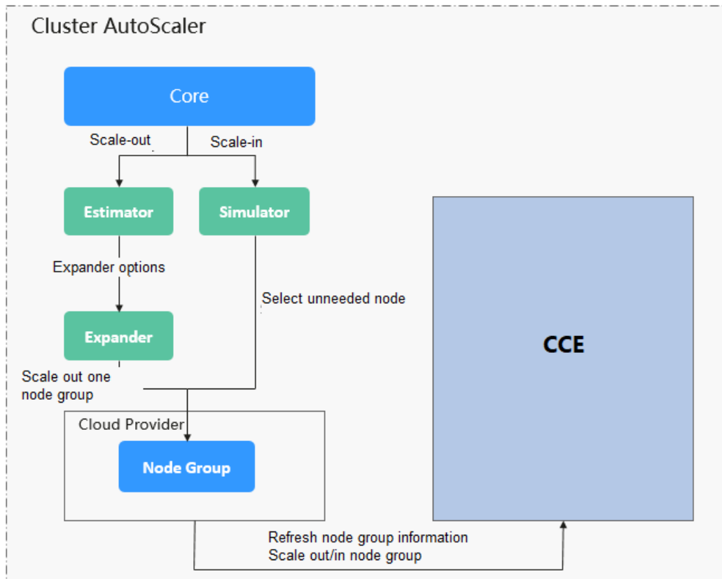
图 3-349 Cluster AutoScaler 架构图
