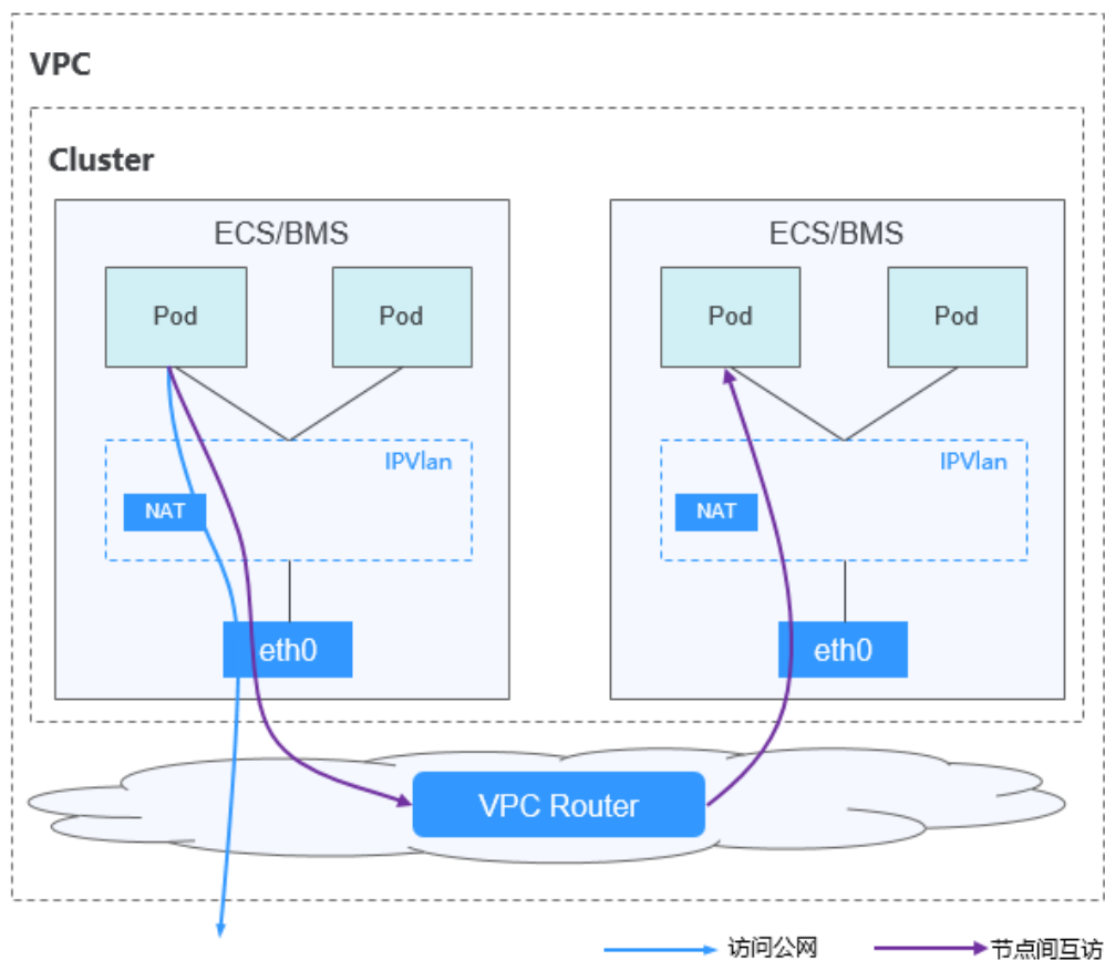
图 3-136 VPC 网络
