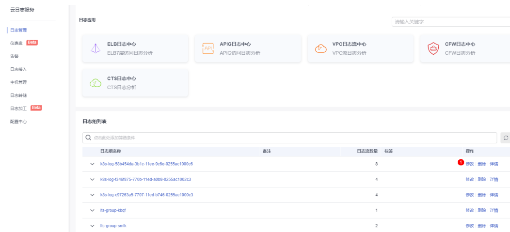
图 3-294 修改日志组
