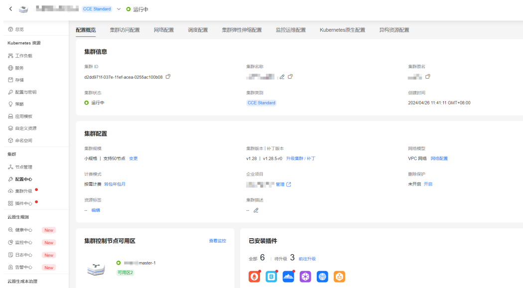
图 3-423 配置概览
