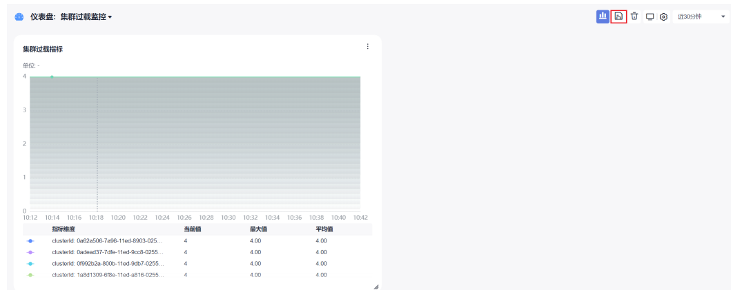
图 3-39 保存仪表盘
