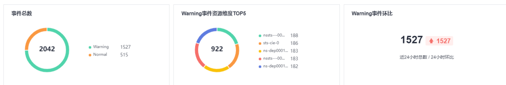
图 3-244 事件统计
