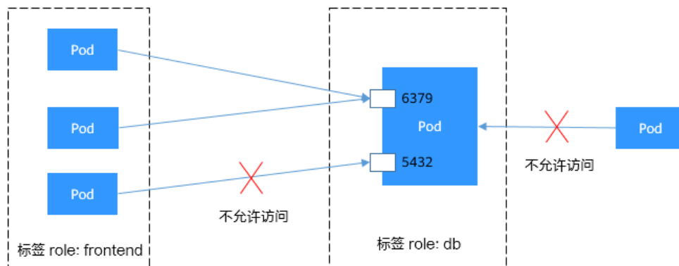
图 3-190 podSelector
