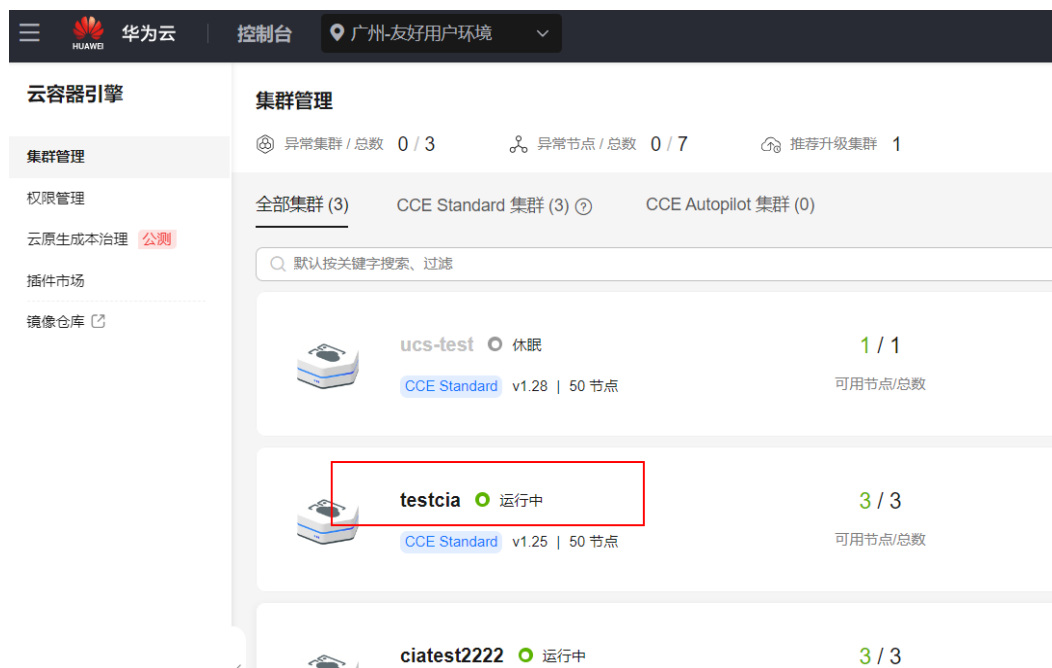
图 3-359 进入集群
