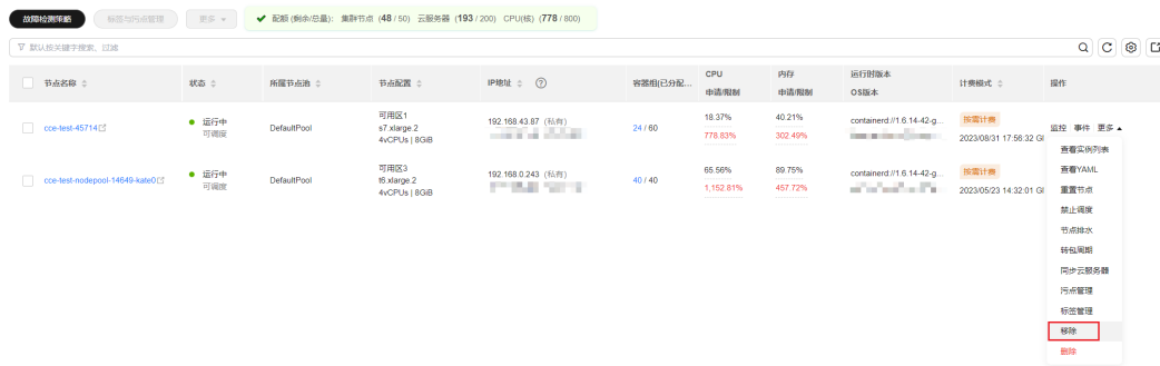
图 3-56 移除节点
