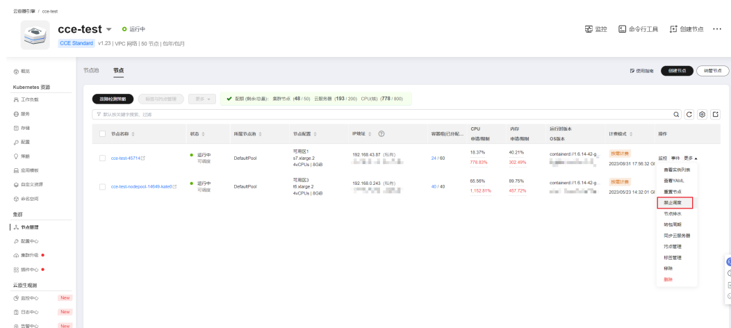
图 3-54 禁止调度
