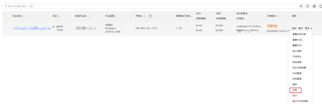
图 3-75 迁移节点
