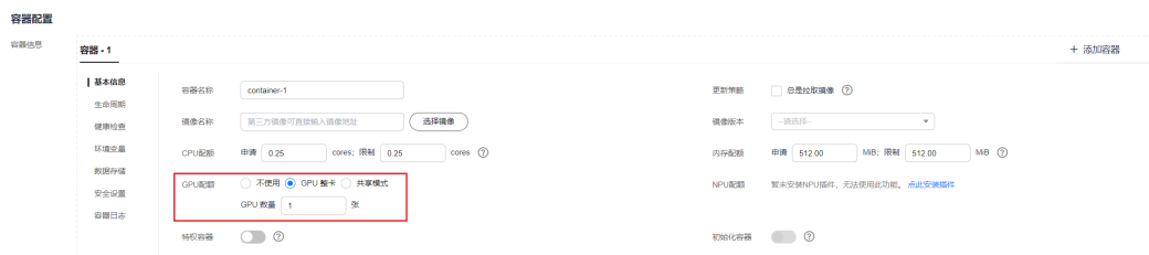
图 3-100 使用 GPU
