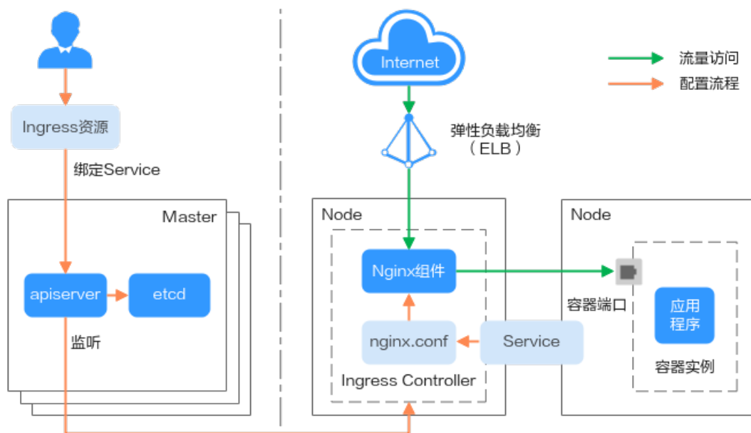
图 3-171 Nginx Ingress Controller 工作原理
