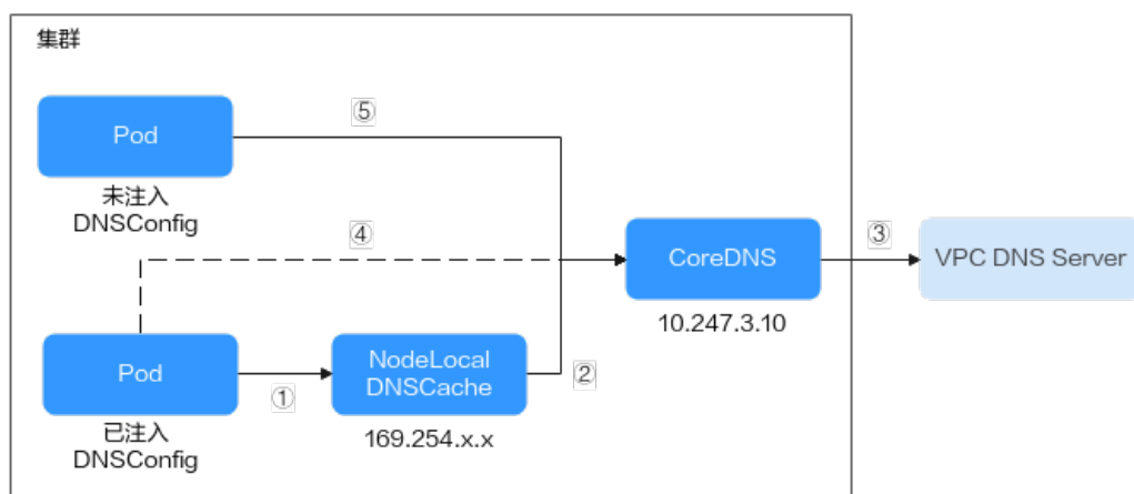
图 3-188 NodeLocal DNSCache 查询路径
