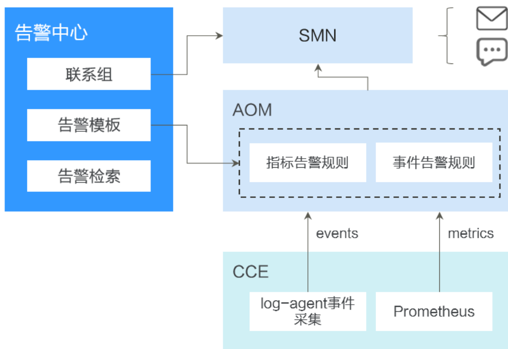
图 3-288 告警中心架构
