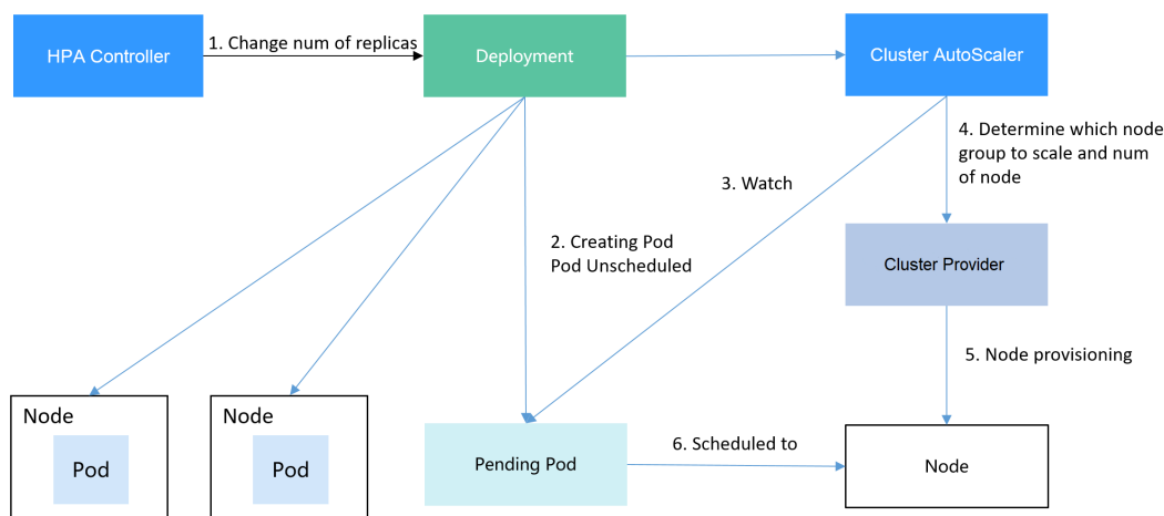
图 3-350 HPA + CA 工作流程
