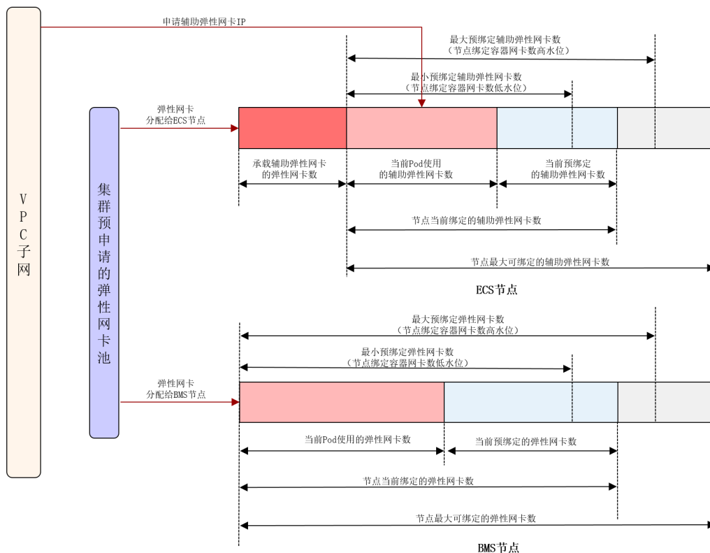
图 3-143 节点绑定容器网卡数总量高低水位策略
