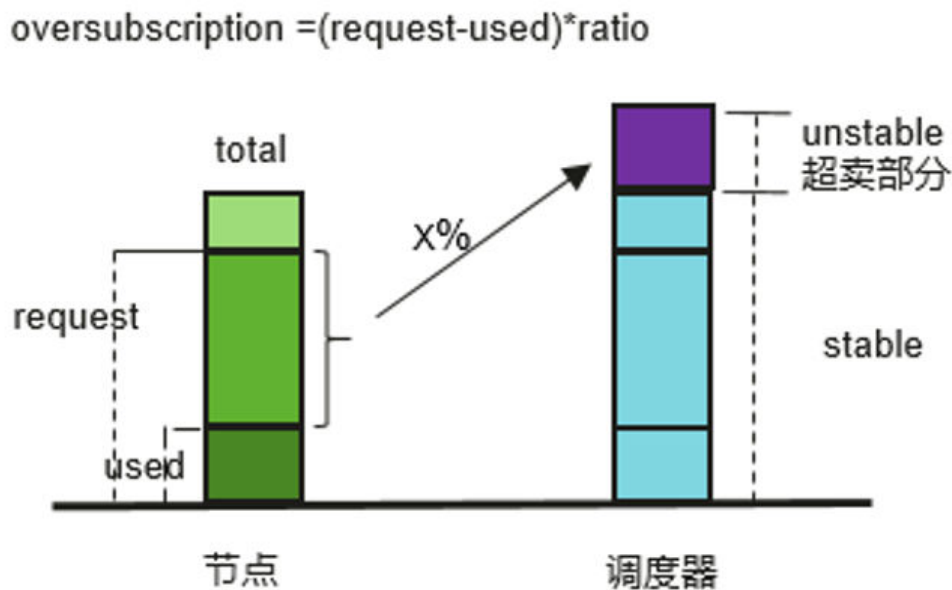
图 3-122 资源超卖示意图
