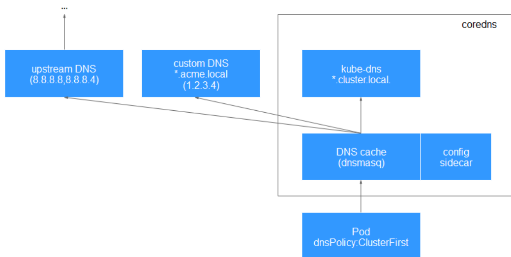
图 3-182 路由请求流程
