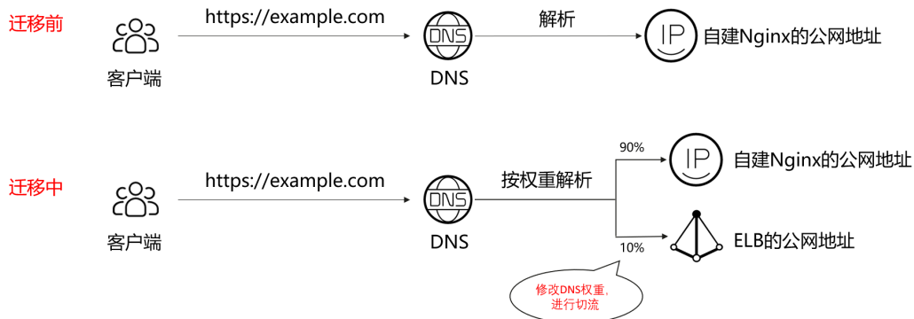
图 3-179 使用 DNS 切流
