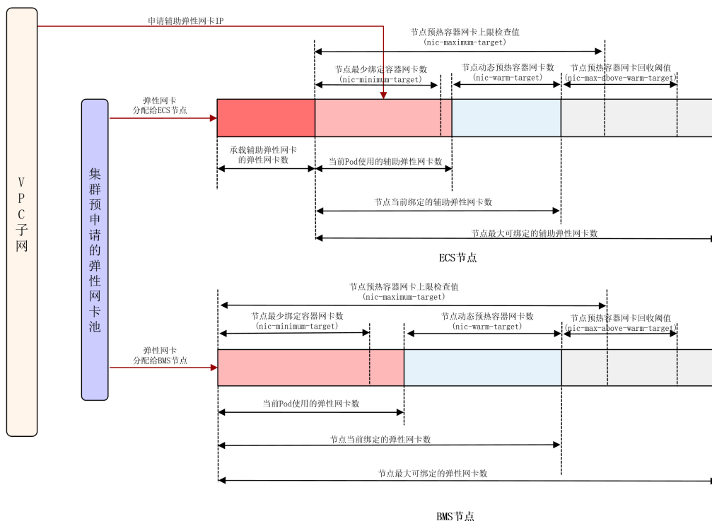
图 3-142 节点容器网卡动态预热策略
