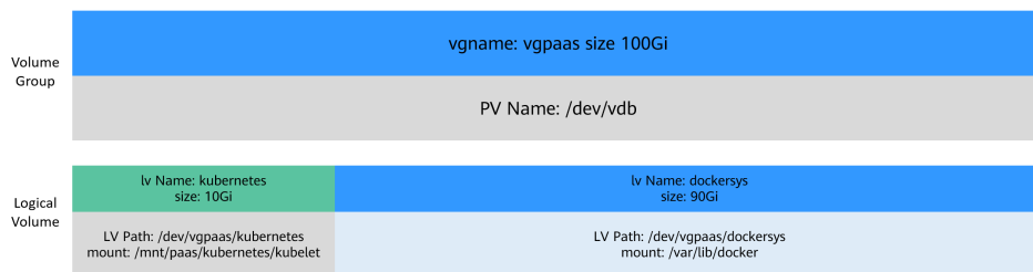
图 3-66 OverlayFS 类型容器引擎空间分配
