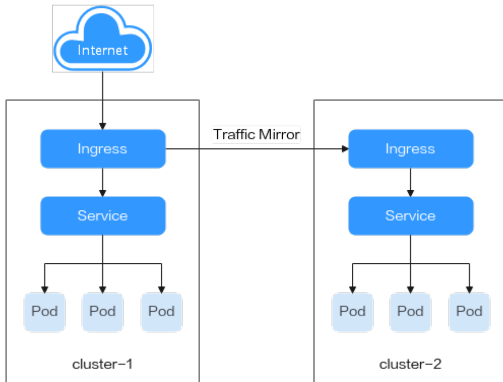
图 3-177 流量镜像
