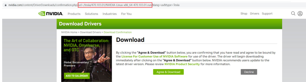
图 3-395 获取链接
