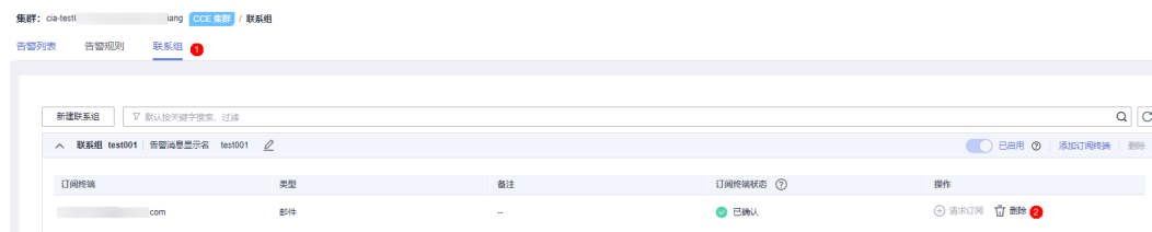
图 3-318 删除联系组
