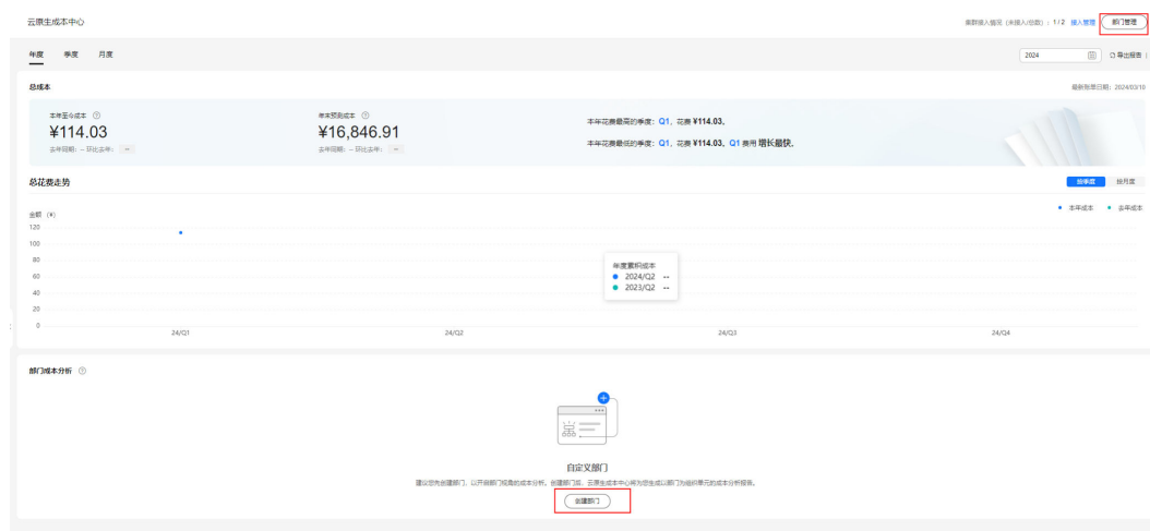
图 3-355 创建部门
