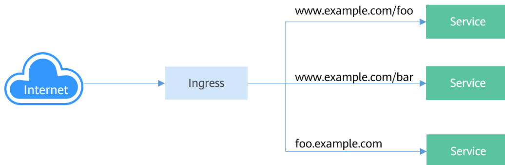
图 3-131 Ingress-Service
