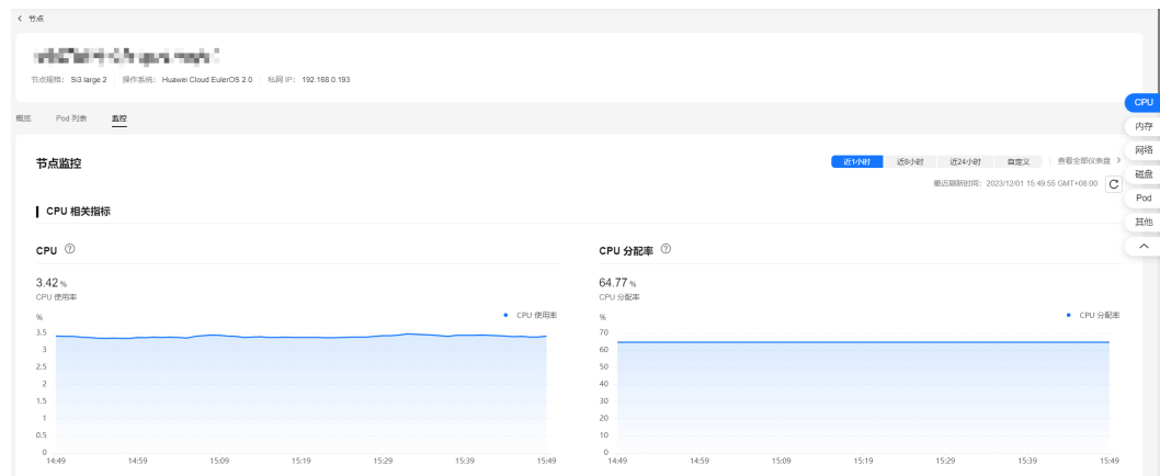
图 3-234 节点监控
