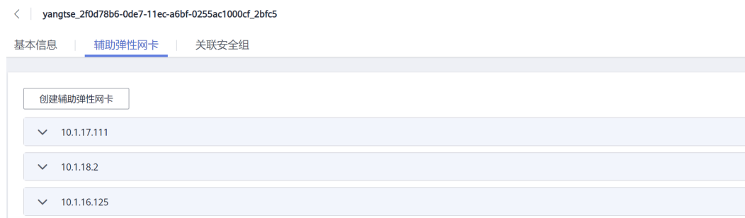
图 3-146 Pod 网卡
