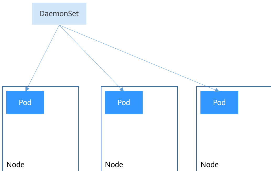
图 3-78 DaemonSet
