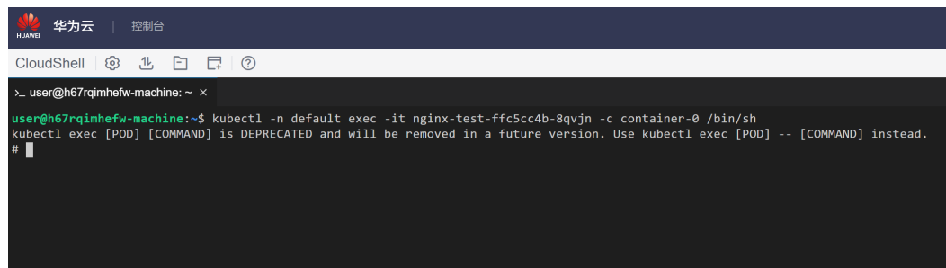
图 3-93 CloudShell 页面
