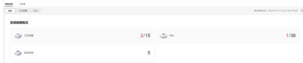
图 4-42 资源概况
