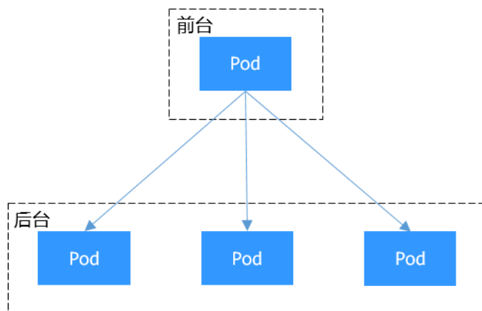
图 3-147 Pod 间访问
