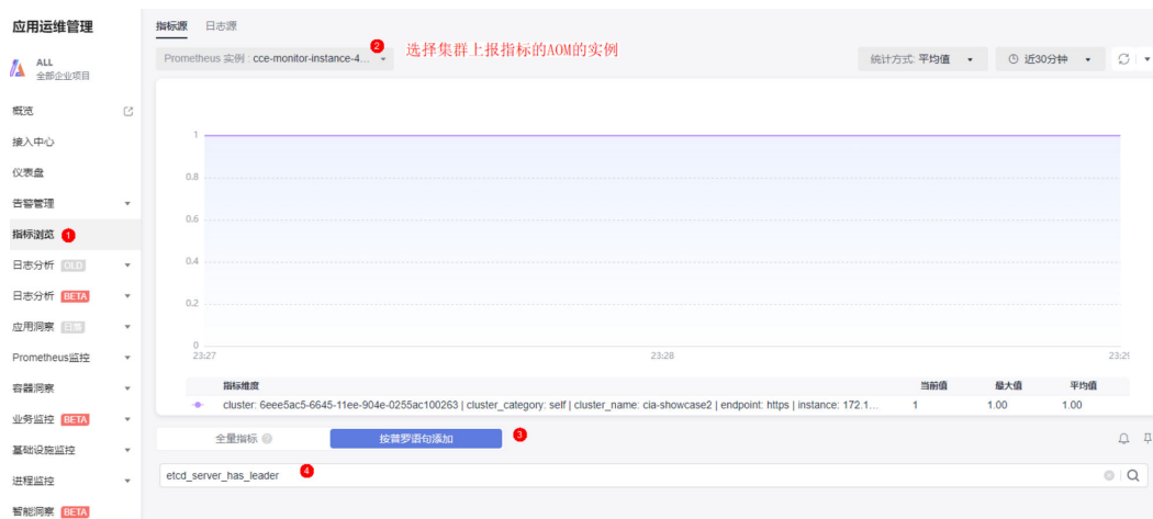
图 3-327 查看指标
