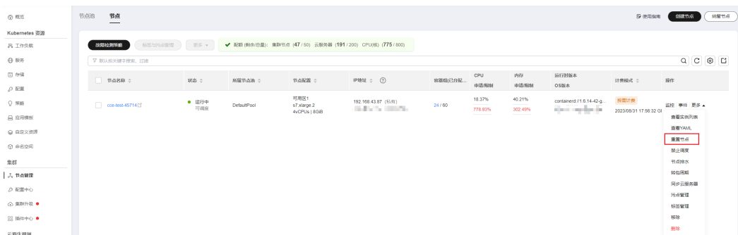
图 3-22 重置节点
