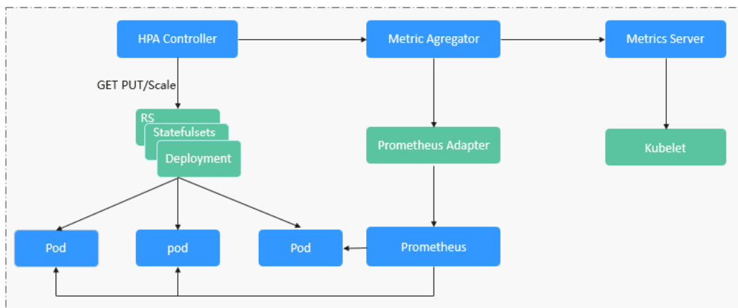
图 3-338 HPA 流程图
