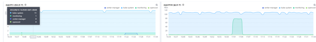
图 4-55 磁盘图表
