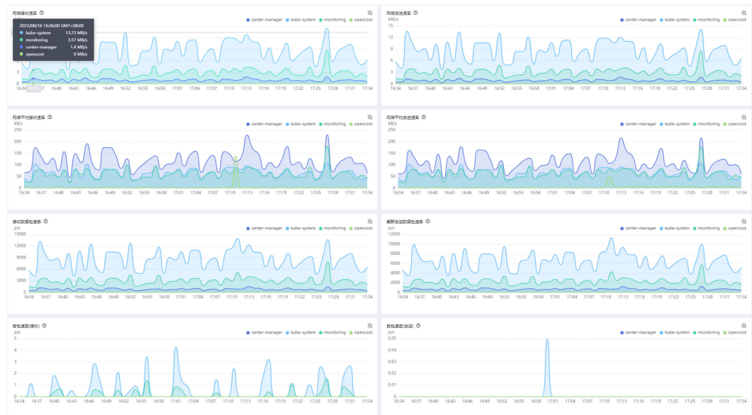
图 4-54 网络图表
