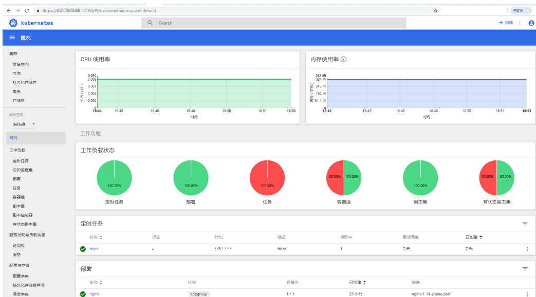
图 3-387 Dashboard 概览页
