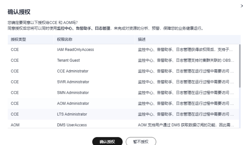
图 3-267 添加授权
