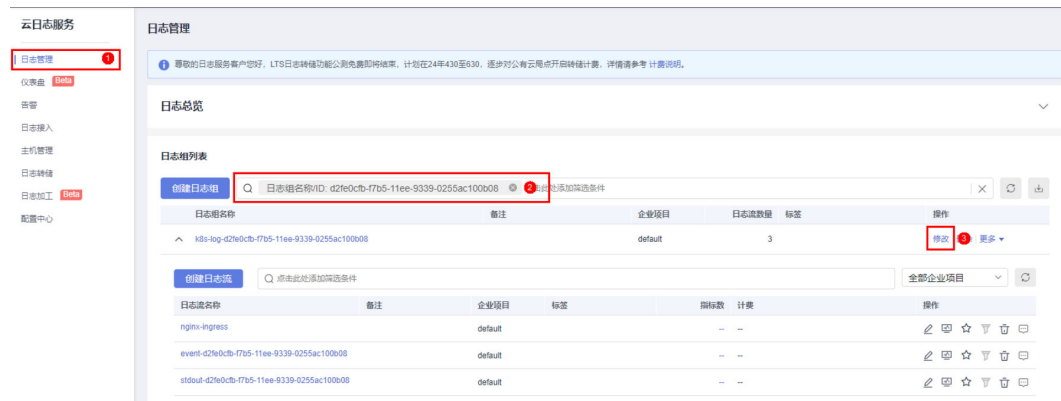
图 3-316 查询日志组
