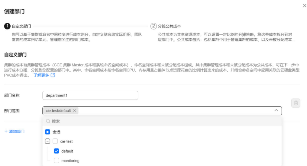
图 3-356 自定义部门
