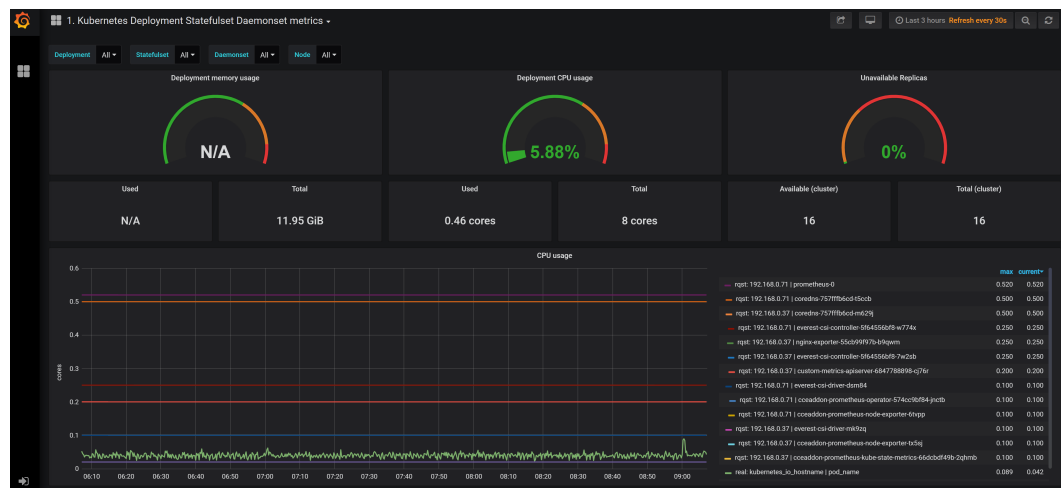
图 3-403 Grafana 面板
