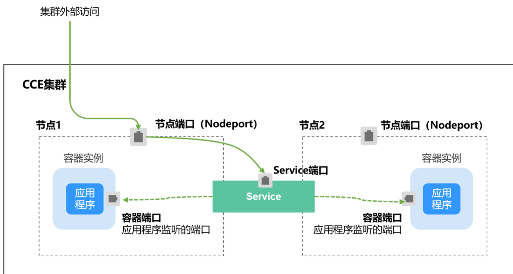
图 3-150 NodePort 访问
