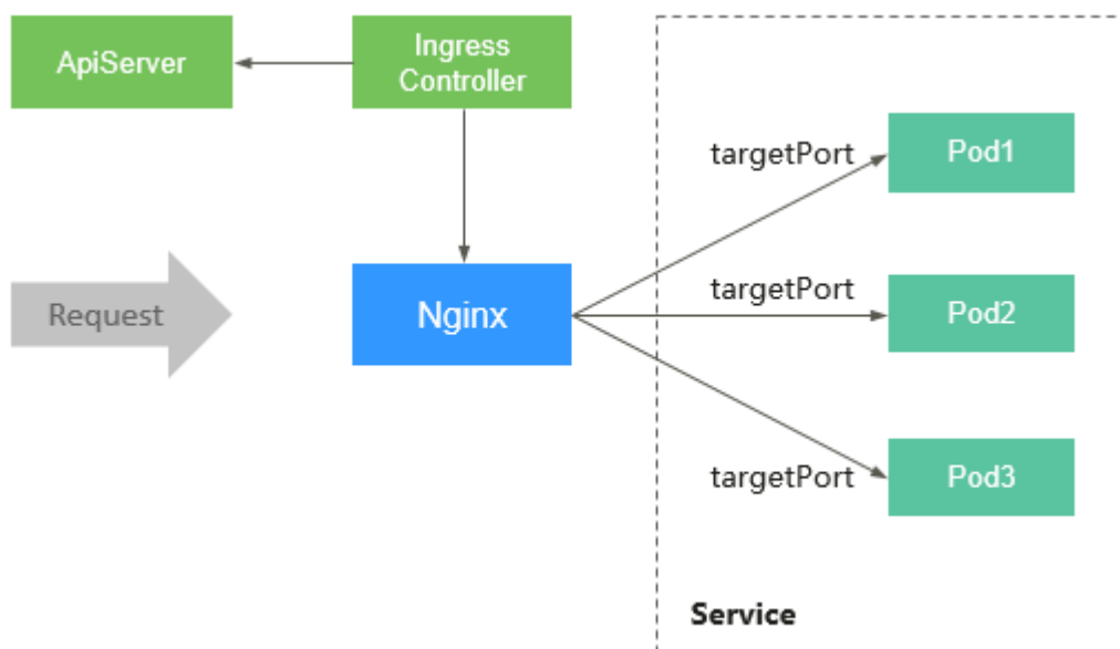
图 3-389 Nginx Ingress 工作原理
