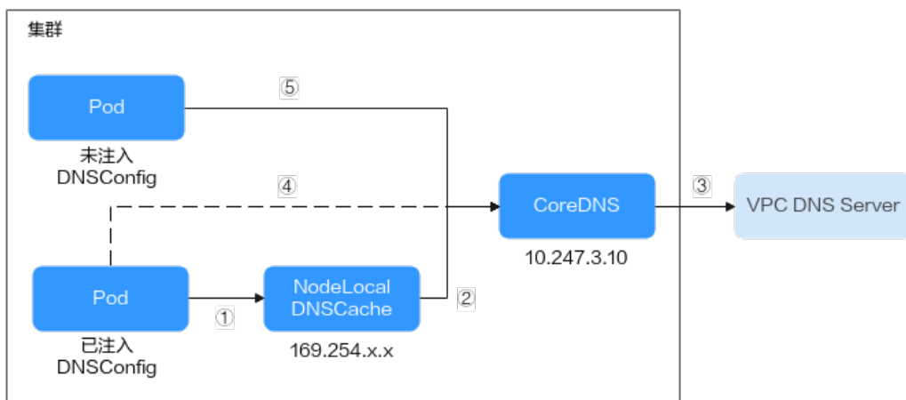
图 3-397 NodeLocal DNSCache 查询路径
