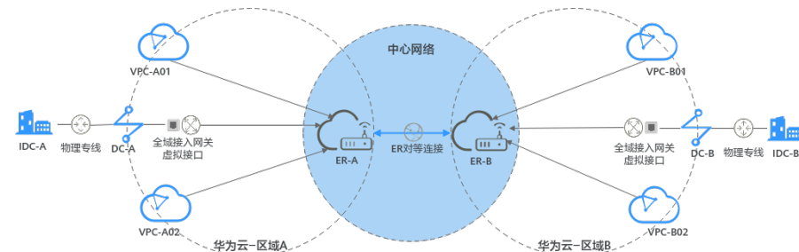
图 2-3 企业路由器与云下数据中心互通
