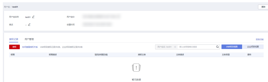
图 1-5 用户组授权
