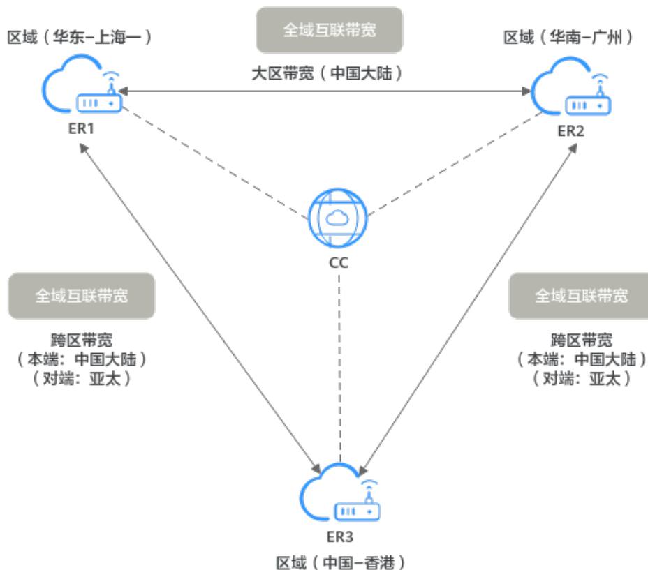
图 3-4 大区/跨区带宽使用场景（中心网络）
