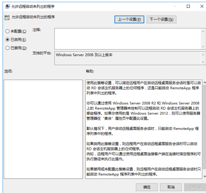
图 12-91 允许远程启动未列出的程序
