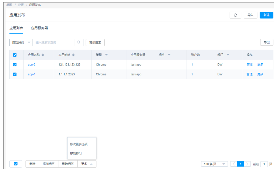
图 6-39 批量修改应用配置
