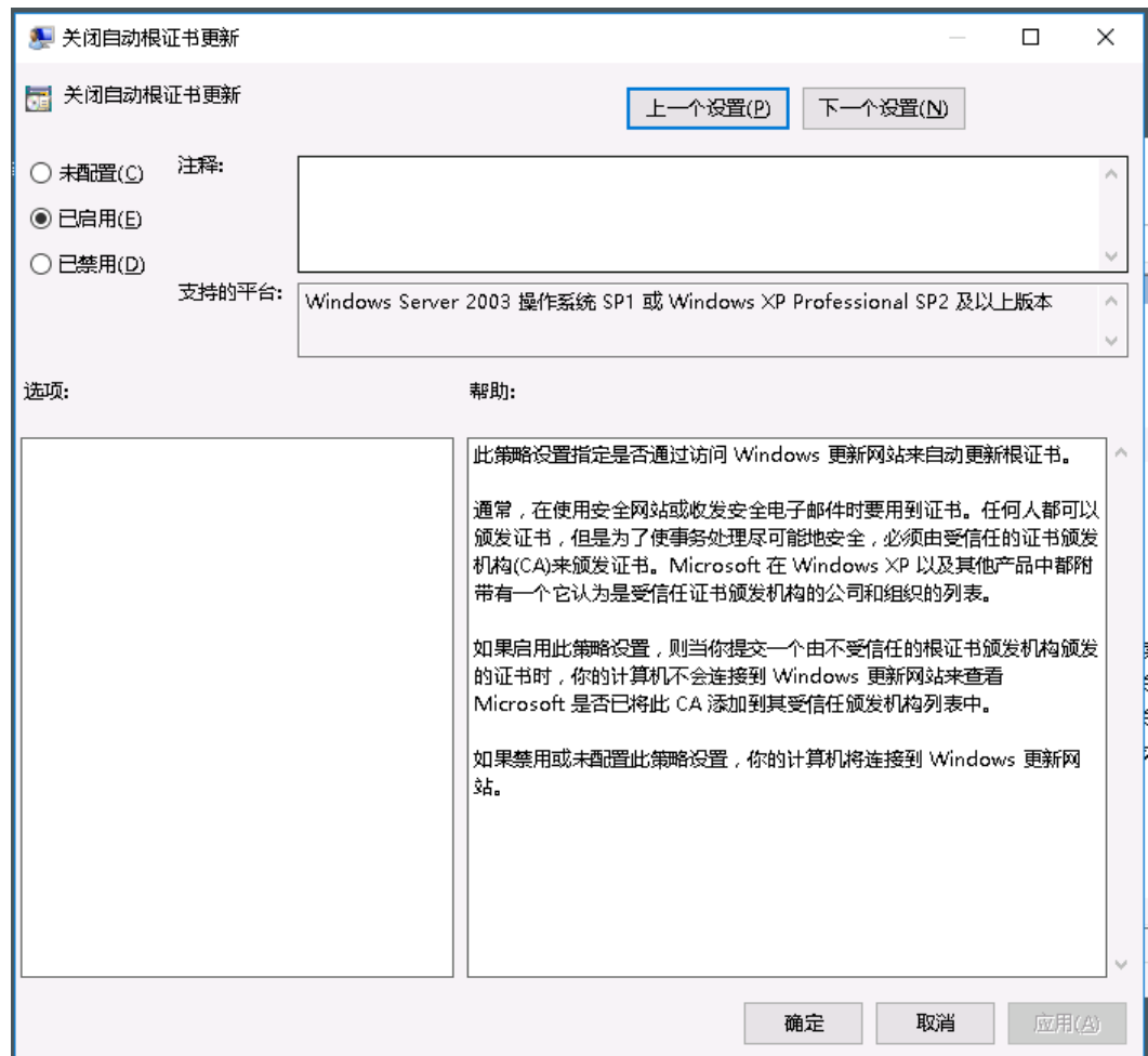
图 12-30 关闭自动根证书更新
