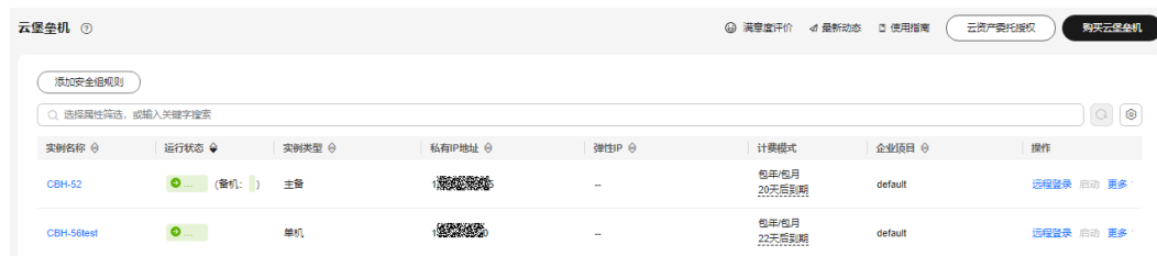
图 4-7 实例列表
