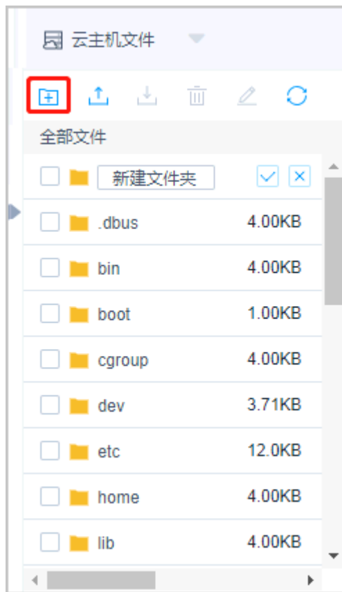
图 9-5 新建文件夹
