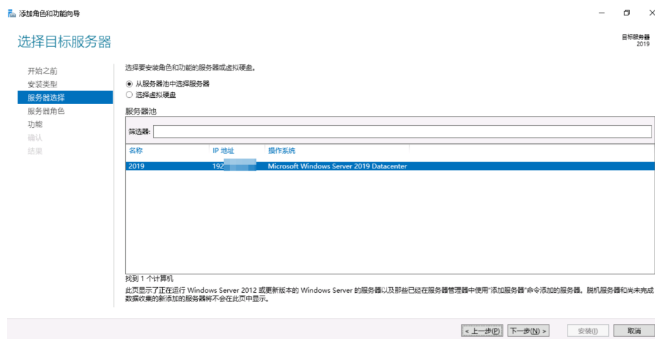
图 18-68 选择服务器
