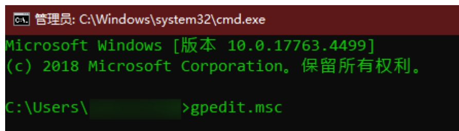
图 18-54 打开组策略
