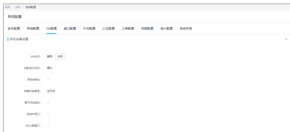
图 14-3 HA 配置
