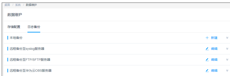
图 17-7 日志备份
