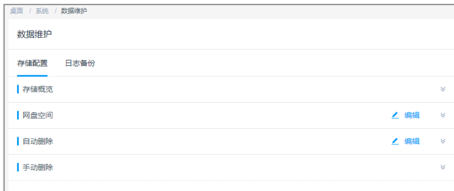
图 17-3 存储配置
