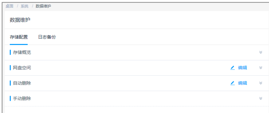
图 17-2 存储配置
