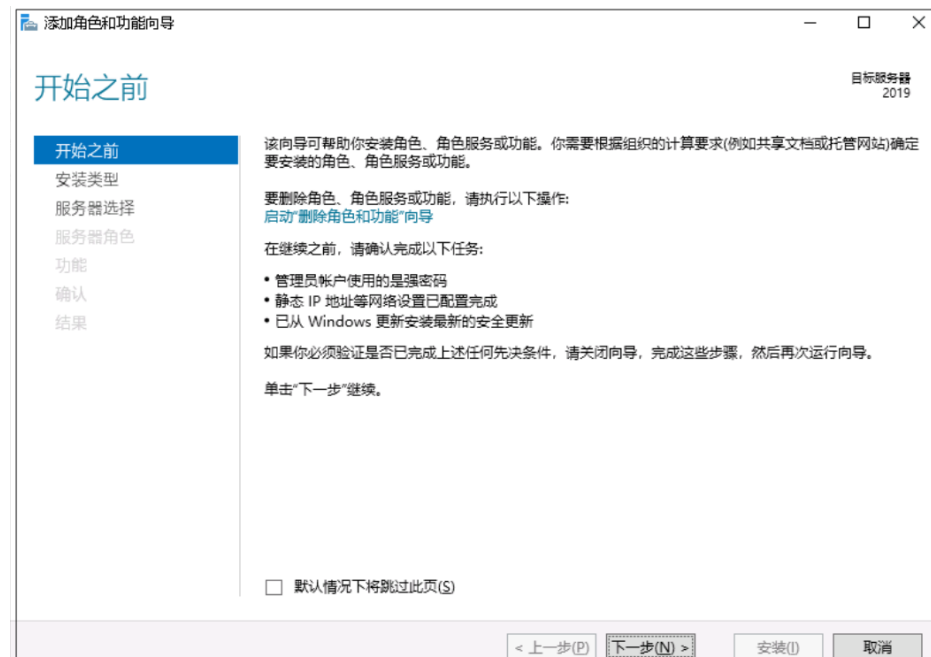
图 18-2 开始之前
