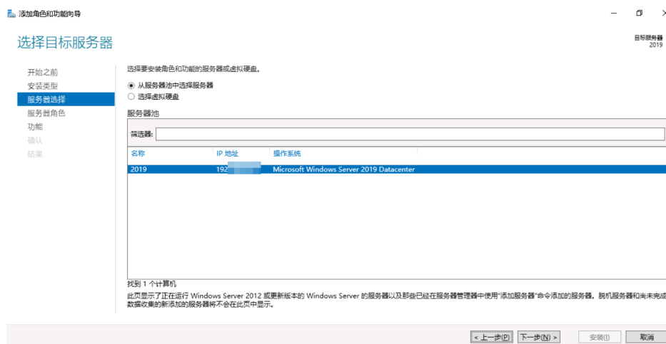
图 18-4 选择服务器
