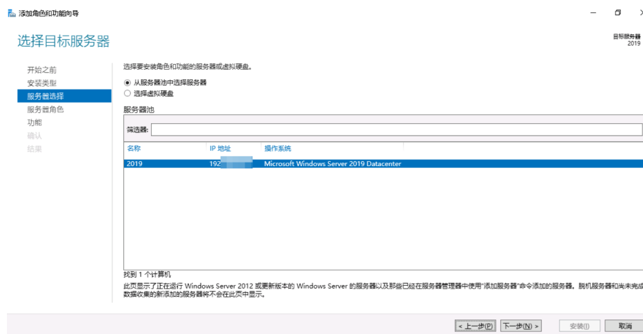
图 18-36 选择服务器
