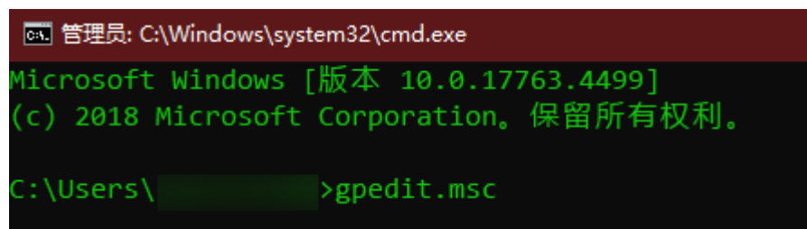
图 18-86 打开组策略
