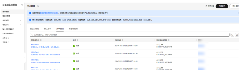
图 21-2 共享密钥
