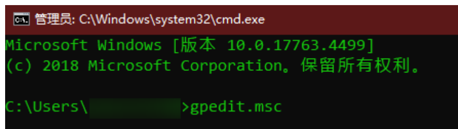
图 18-22 打开组策略
