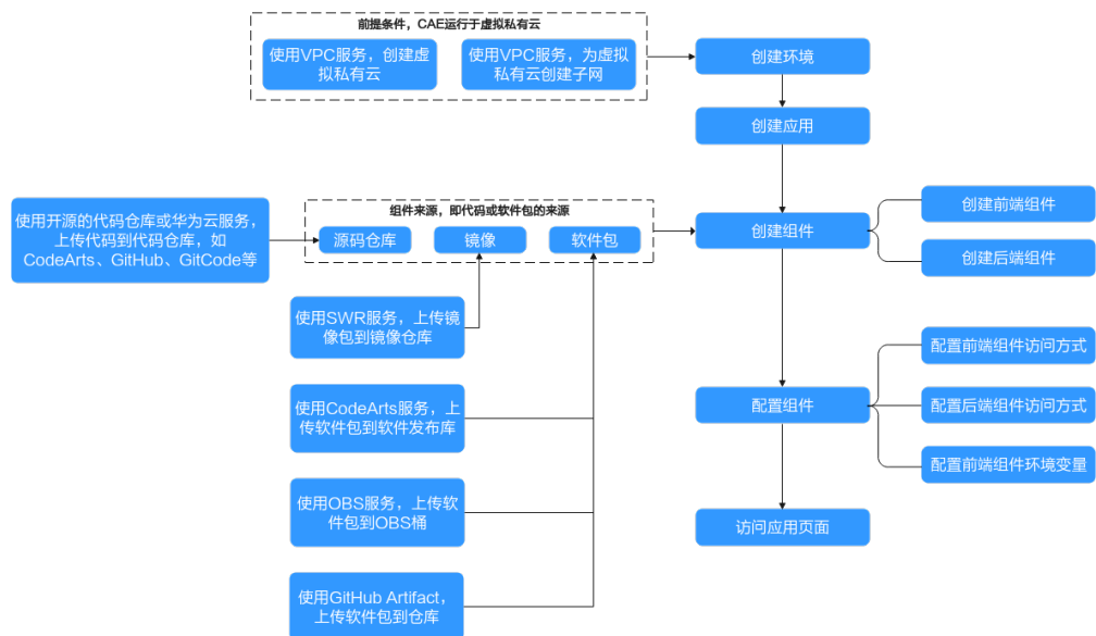
图 1-1 云应用引擎使用流程
