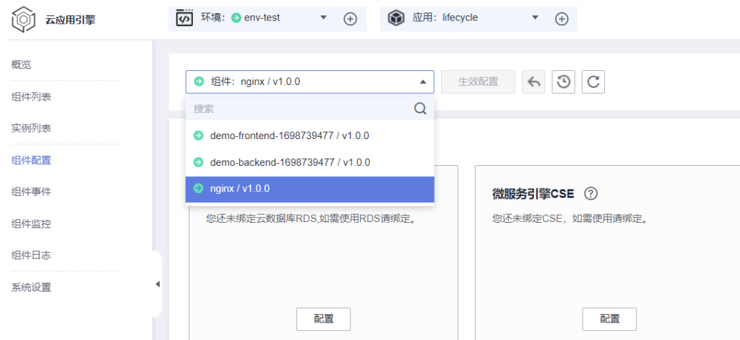
图 7-57 选择组件
