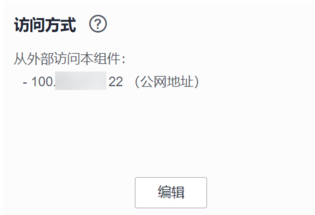
图 7-18 外网访问
