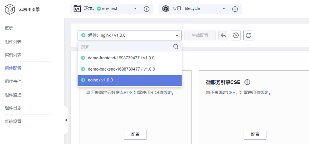
图 7-43 选择组件
