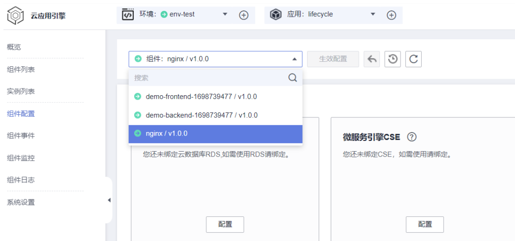
图 7-54 选择组件
