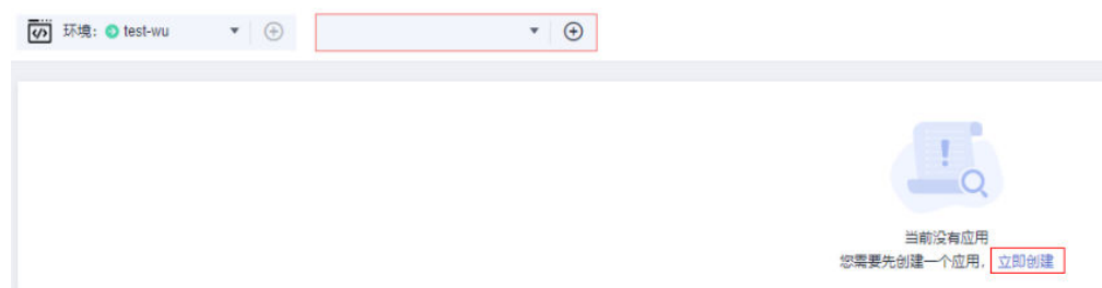
图 4-1 创建应用
