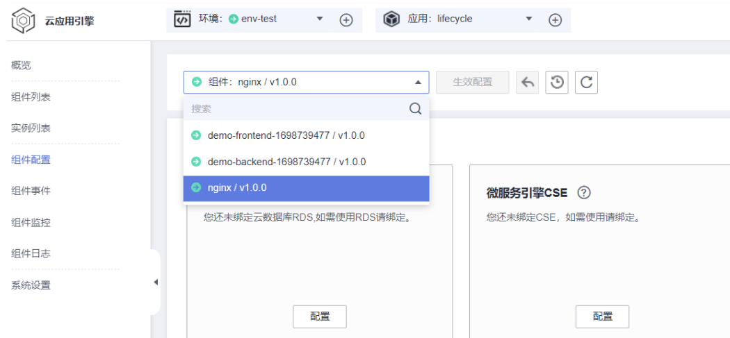
图 7-14 选择组件
