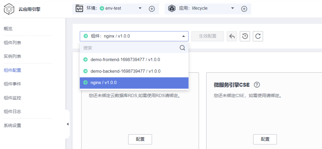
图 7-61 选择组件
