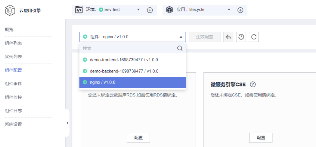
图 7-6 选择组件
