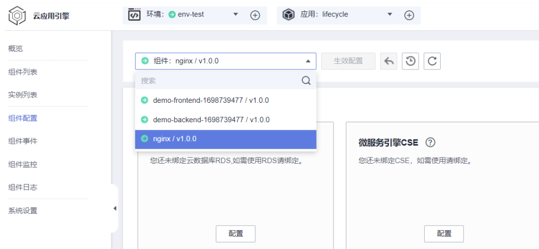
图 7-59 选择组件
