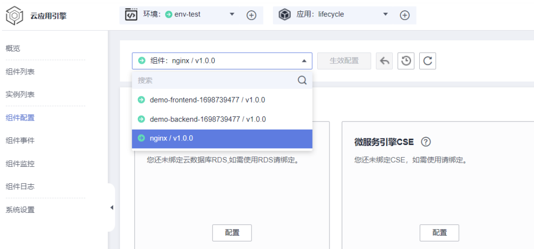
图 7-38 选择组件
