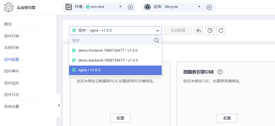
图 7-76 选择组件
