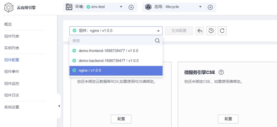
图 7-8 选择组件
