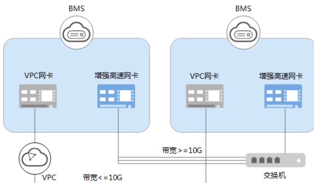
图 6-7 增强高速网络架构
