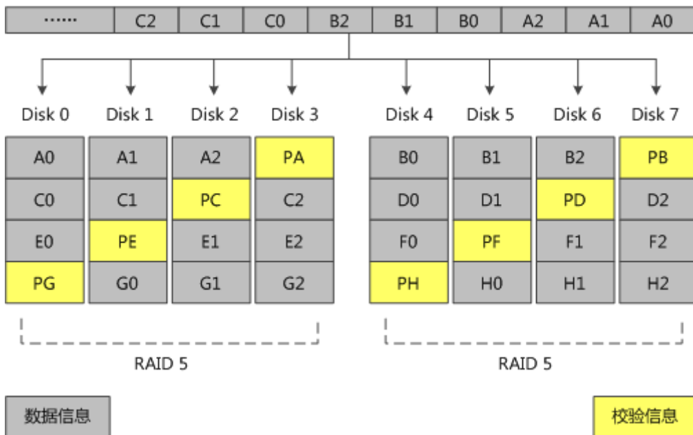
图 4-39 RAID 50 数据存储原理
