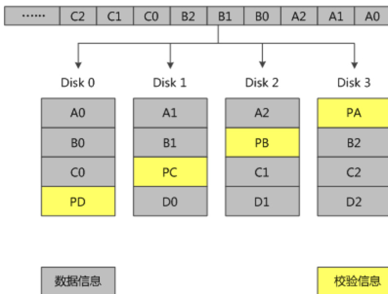
图 4-36 RAID 5 数据存储原理
