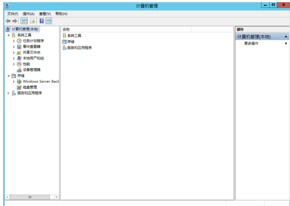
图 4-22 计算机管理
