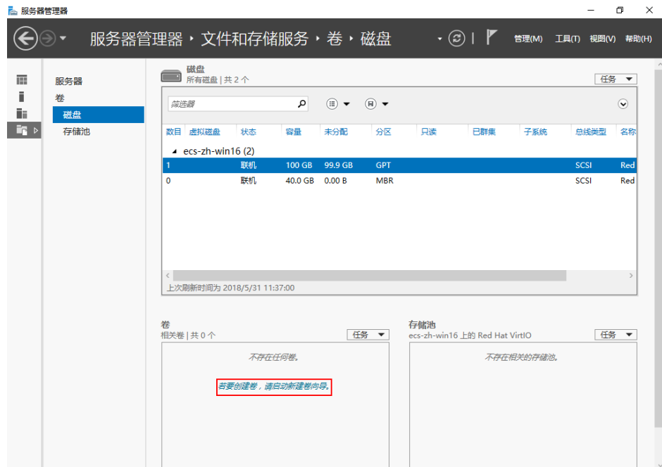
图 4-9 初始化完成
