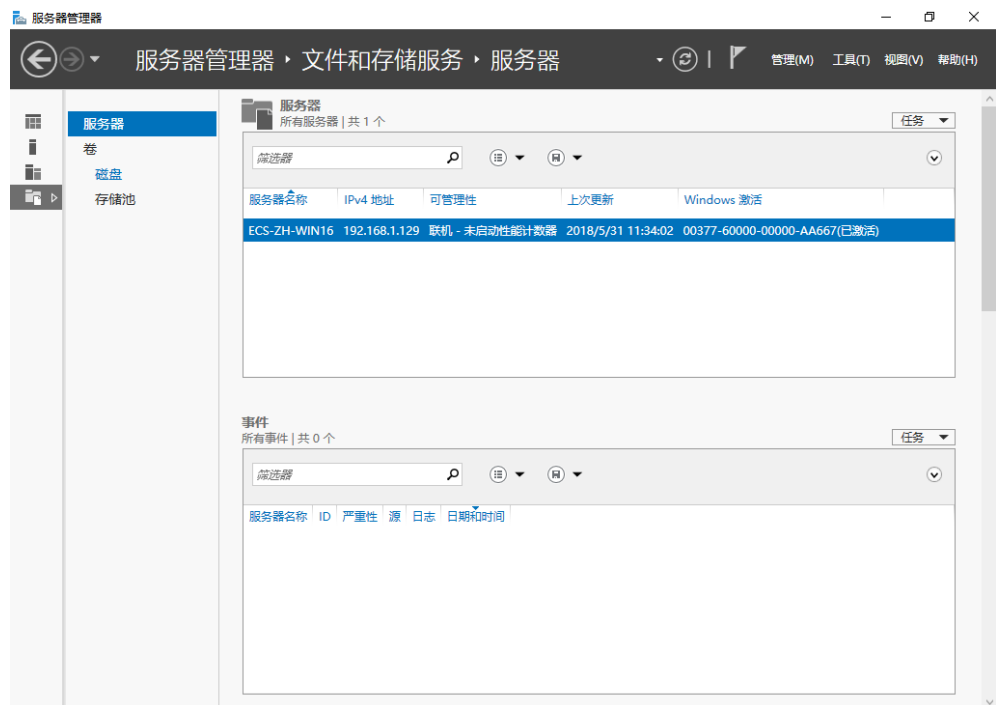
图 4-4 服务器
