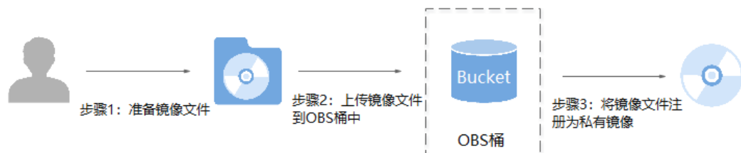
图 3-3 创建过程
