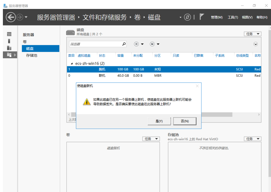
图 4-6 使磁盘联机
