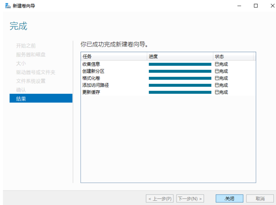
图 4-16 新建卷完成
