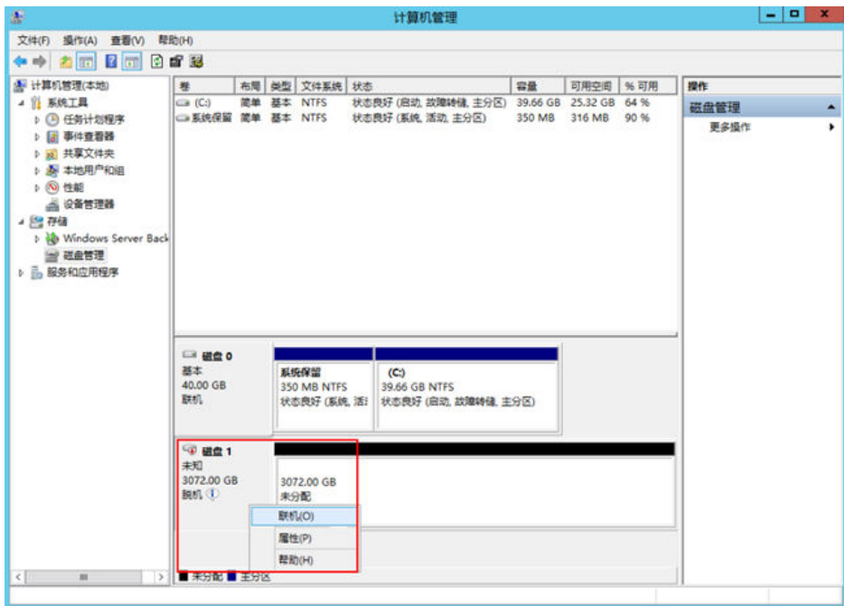
图 4-23 磁盘列表
