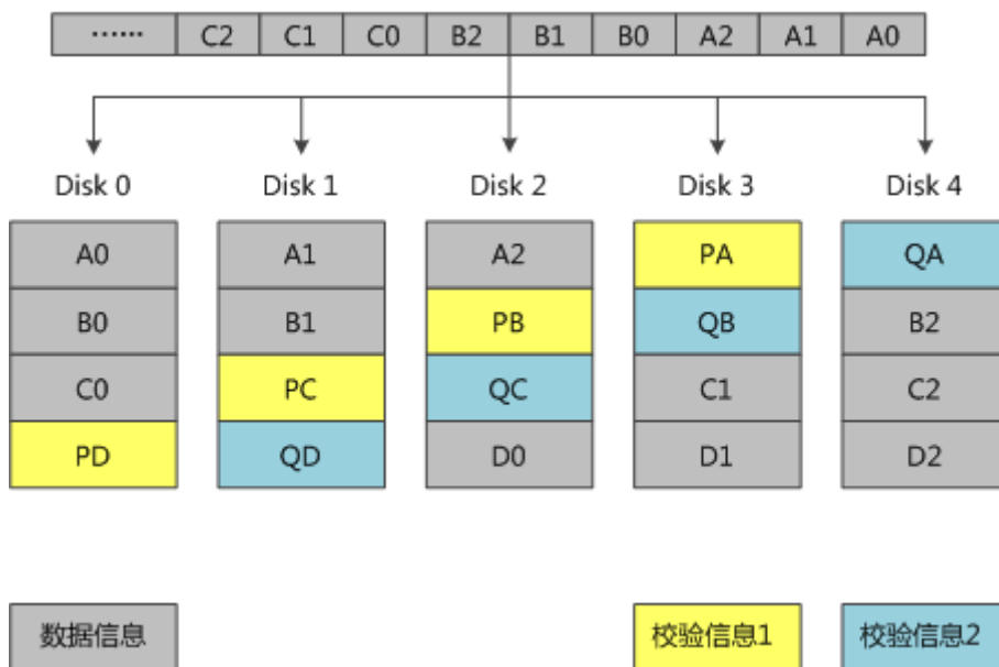
图 4-37 RAID 6 数据存储原理
