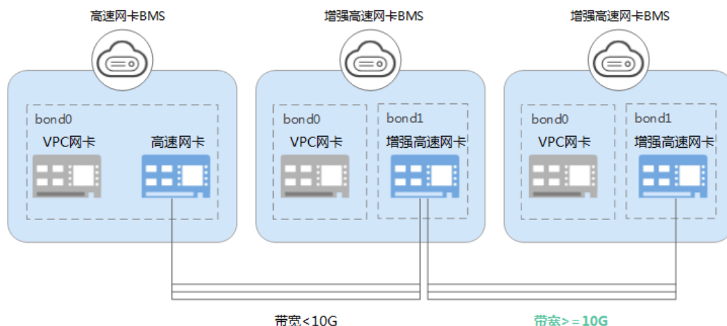
图 6-9 两代高速网络对比
