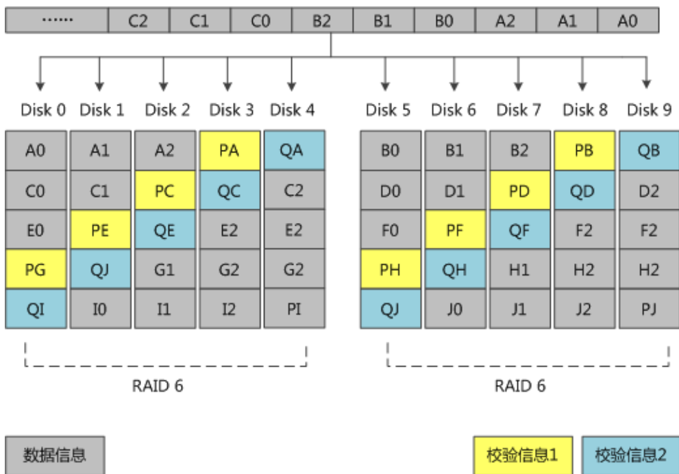
图 4-40 RAID 60 数据存储原理
