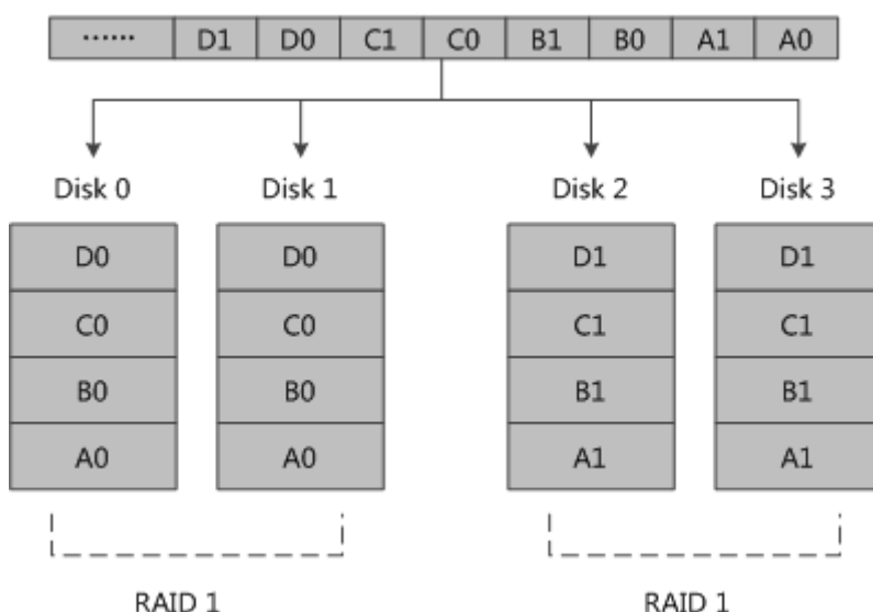
图 4-38 RAID 10 数据存储原理
