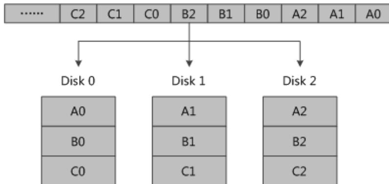
图 4-34 RAID 0 数据存储原理
