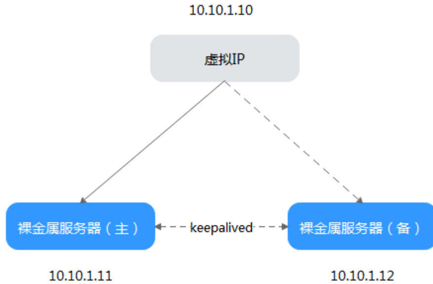
图 6-5 高可用性模式组网图
