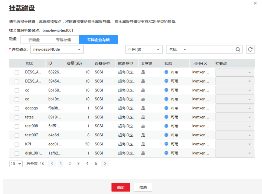
图 4-1 挂载磁盘
