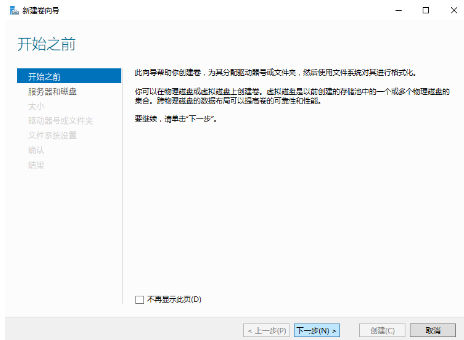
图 4-10 新建卷向导
