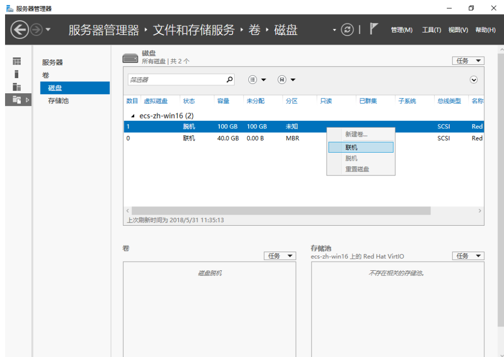
图 4-5 磁盘
