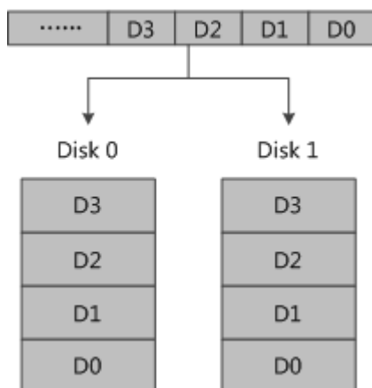
图 4-35 RAID 1 数据存储原理
