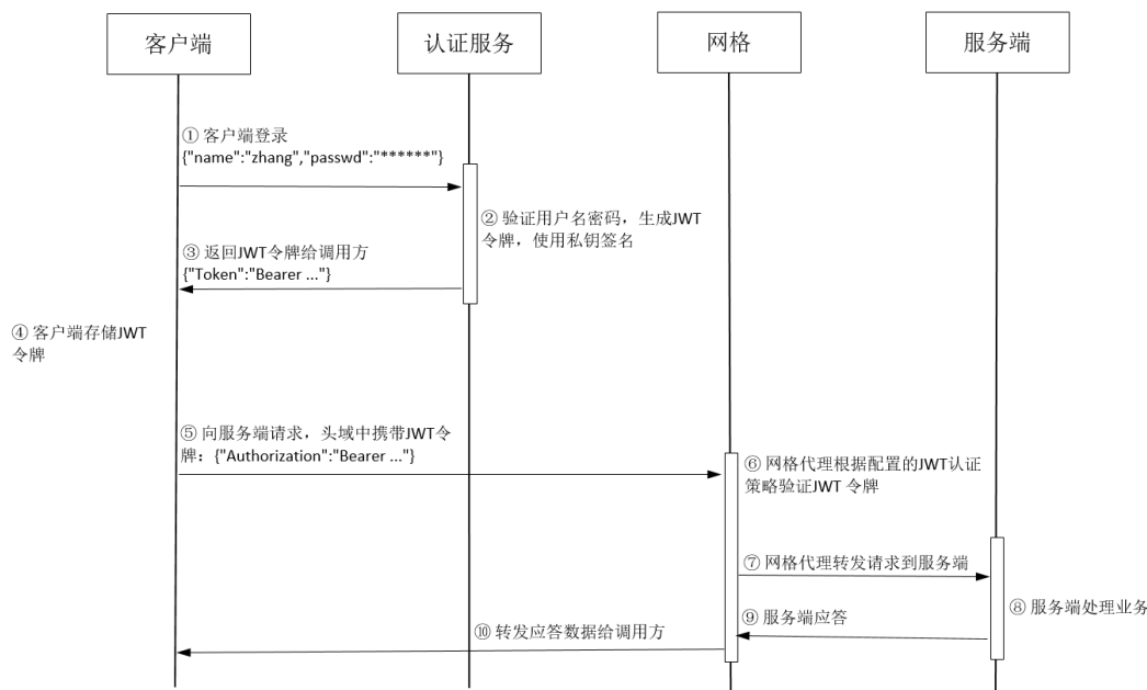
图 1-47 Istio JWT 认证流程
