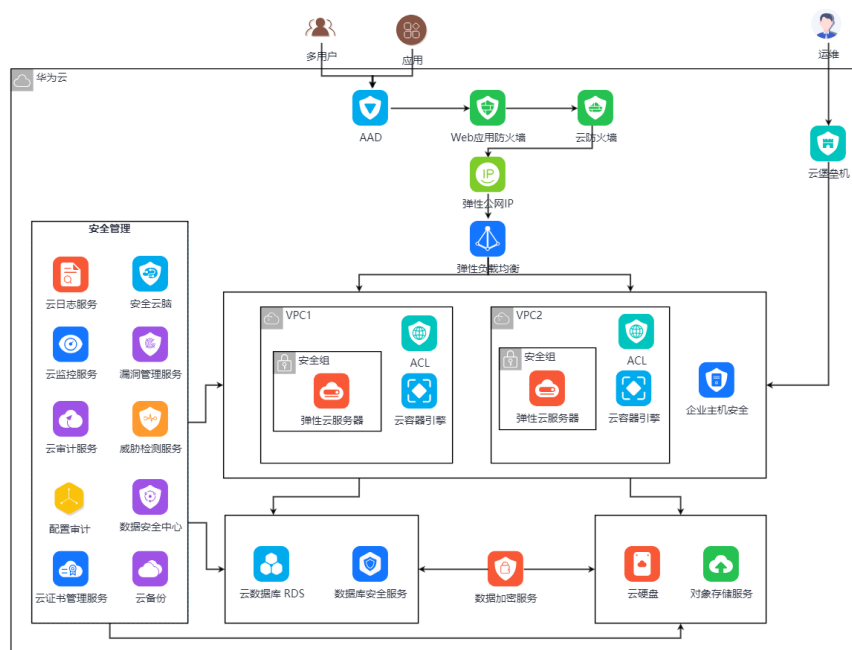
图 3-6 单账号的工作负载级的安全参考架构
