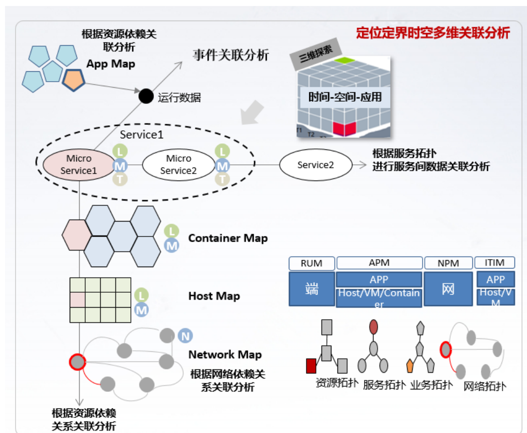
图 4-4 根因定位定界
