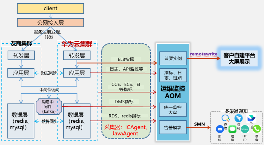
图 6-2 解决方案结构图
