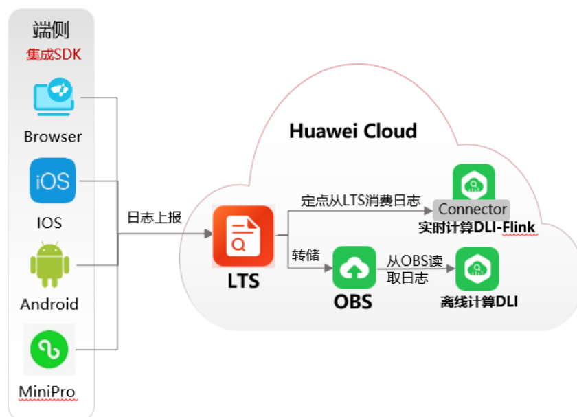
图 6-3 解决方案结构图
