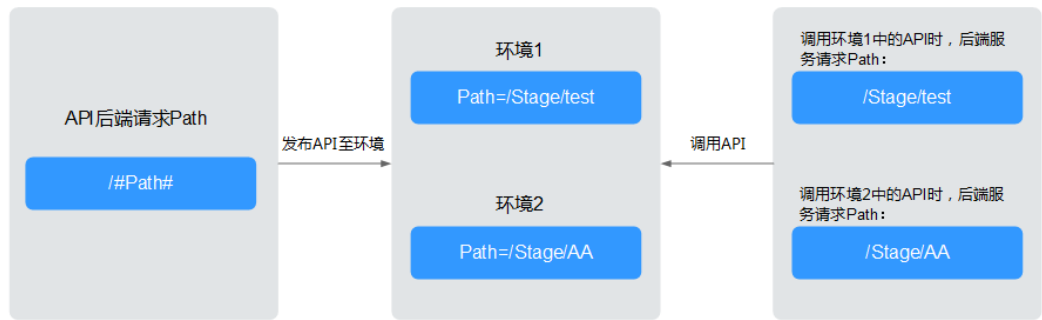
图 13-29 环境变量
