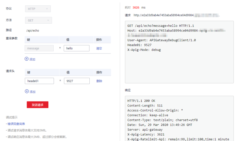
图 13-17 调试界面
