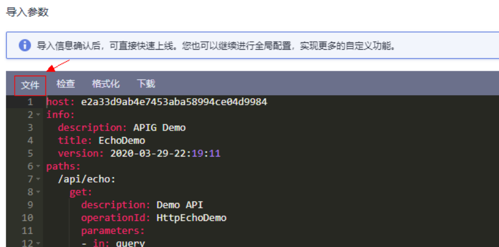
图 13-21 导入参数
