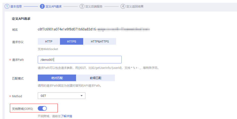
图 13-13 支持跨域
