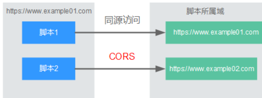
图 6-1 跨域访问
