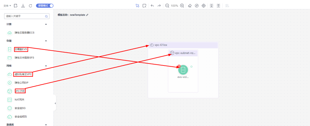
图 2-14 添加元素
