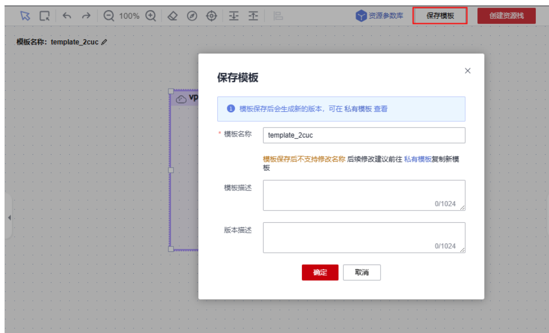
图 2-17 保存模板
