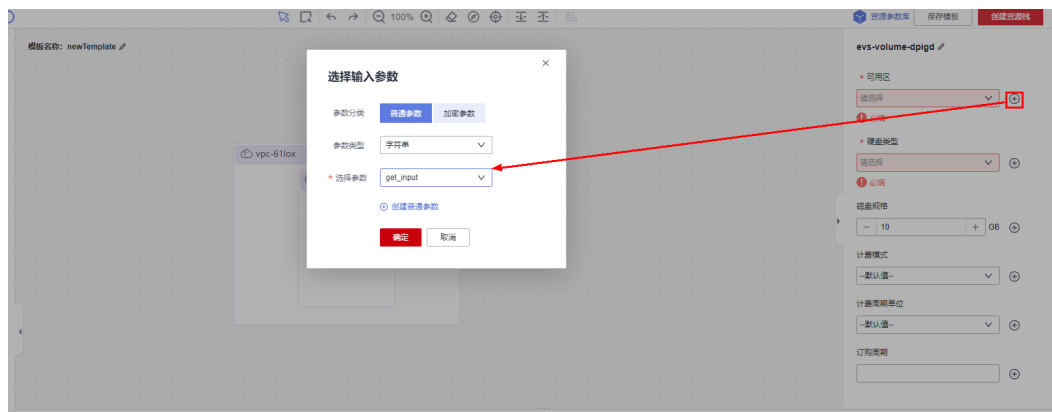
图 2-16 生成 input
