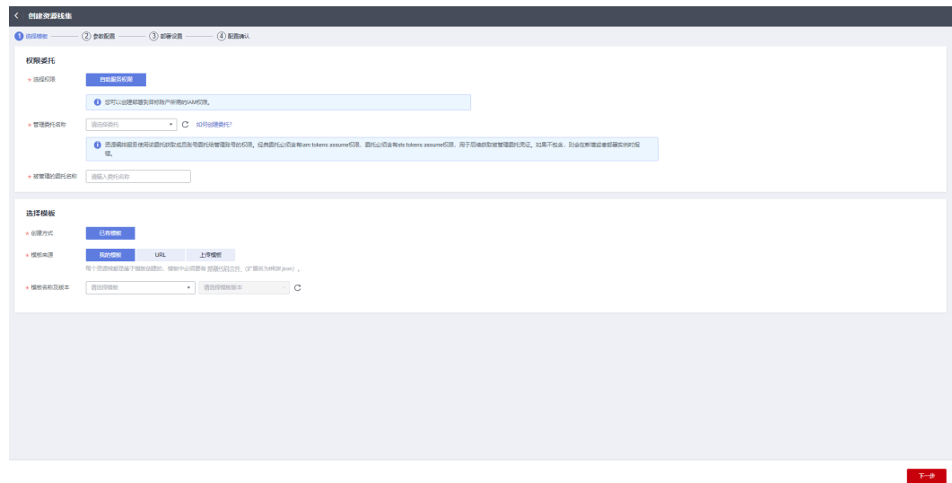
图 4-2 选择模板
