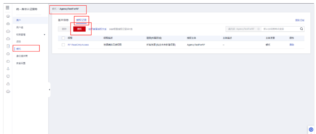
图 6-3 委托授权
