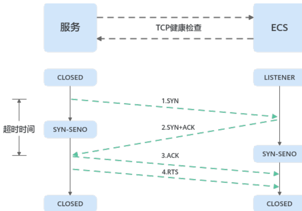
图 5-1 TCP 健康检查
