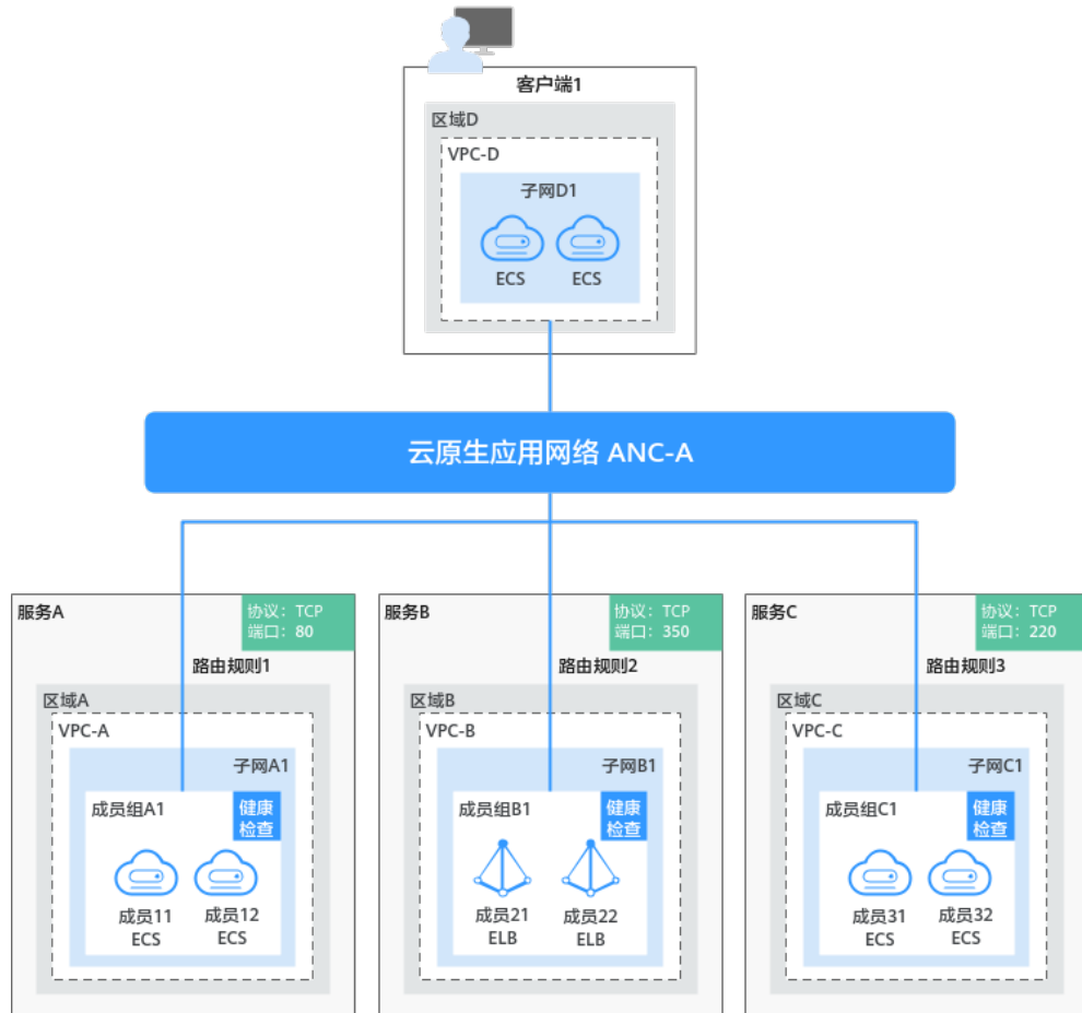
图 6-2 共享 ANC 组网示例-关联不同账号下的服务
