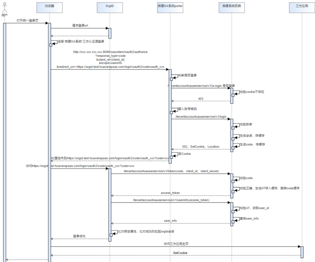
自建OA账号登录流程图：
