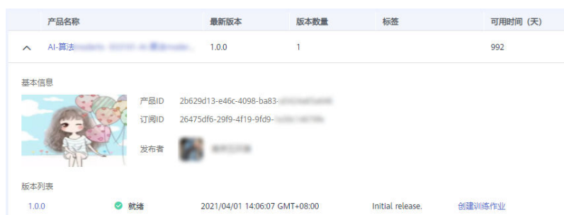
图 5-3 同步算法
