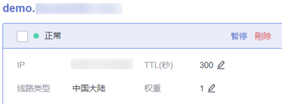
图 10-5 调度策略
