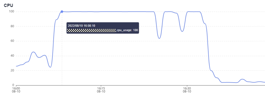
图 5-1 CPU 使用率
