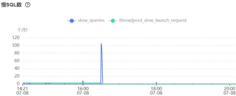
图 5-7 慢 SQL 数
