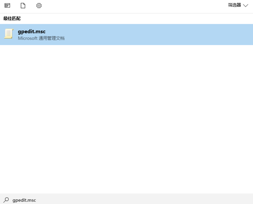
图 12-1 输入 gpedit.msc
