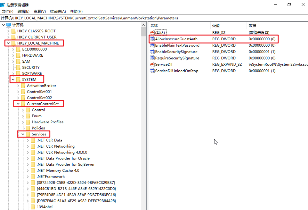
图 12-5 进入注册表
