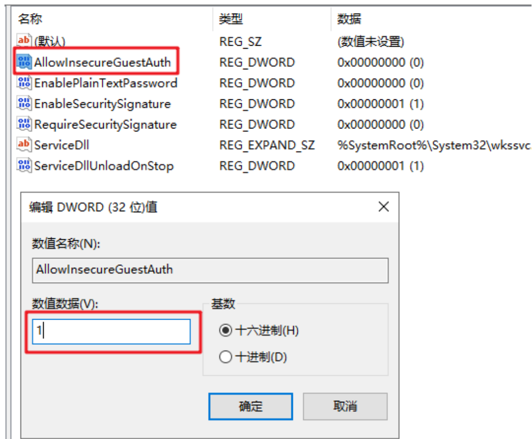
图 12-6 修改值
