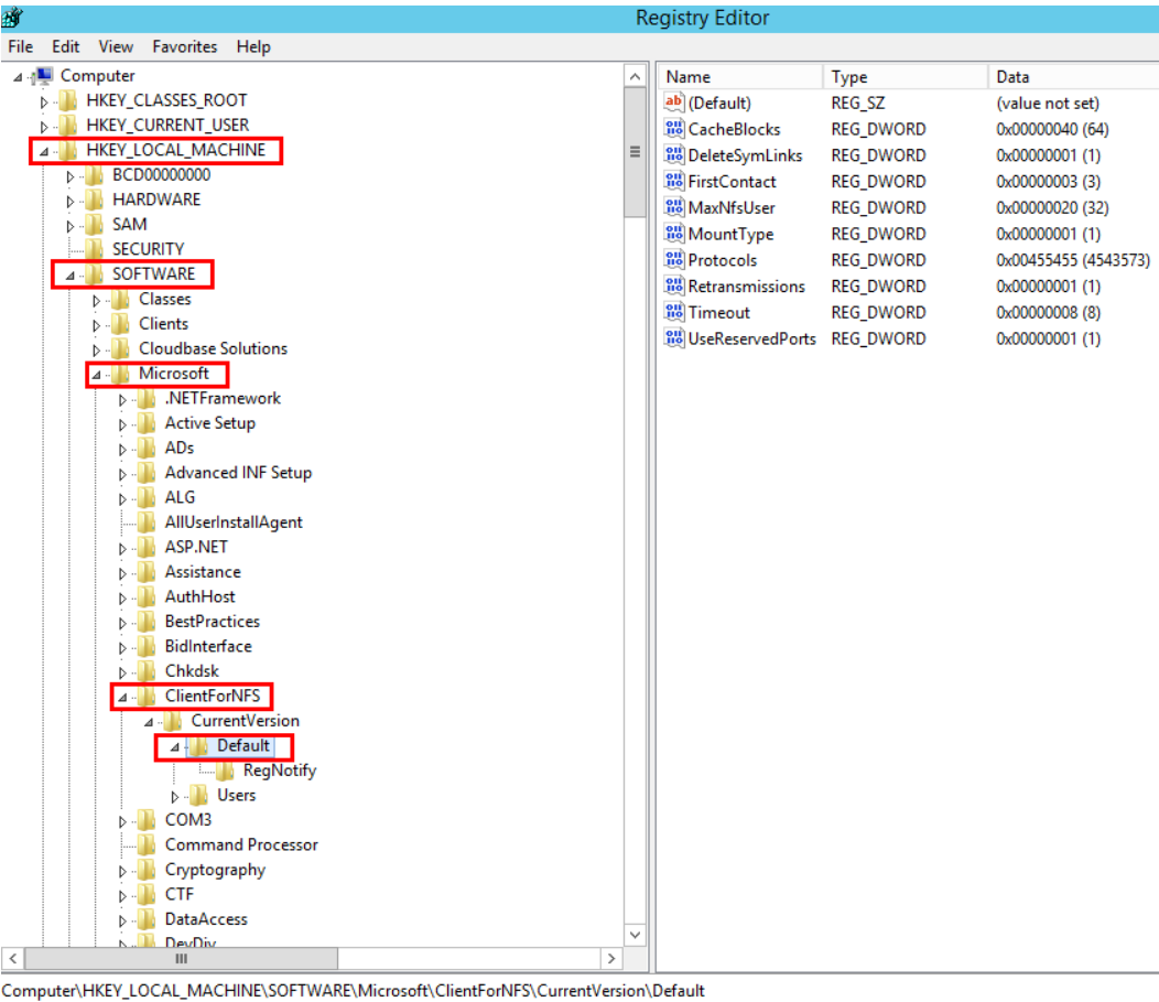
图 8-1 进入目录
