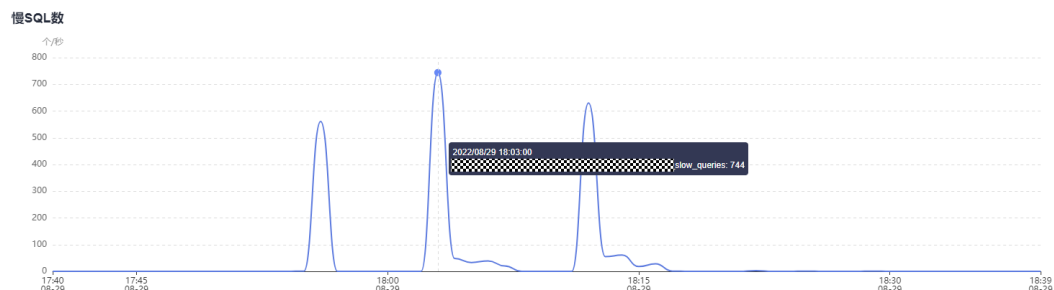
图 1-14 慢 SQL 数
