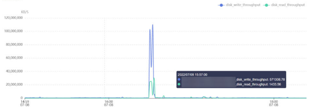
图 1-12 磁盘吞吐
