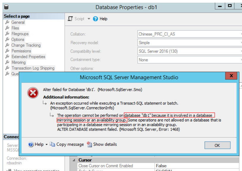
图 3-8 报错信息
