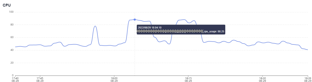
图 1-15 CPU 使用率
