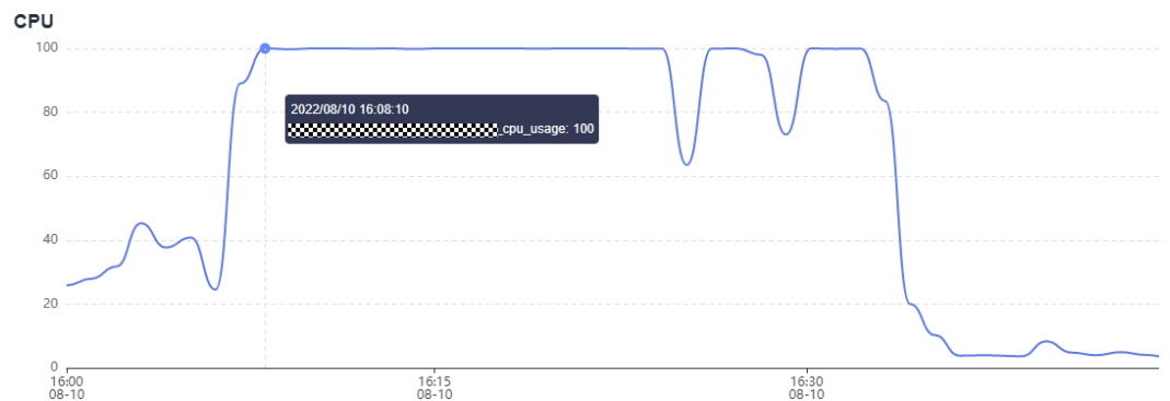
图 1-5 CPU 使用率
