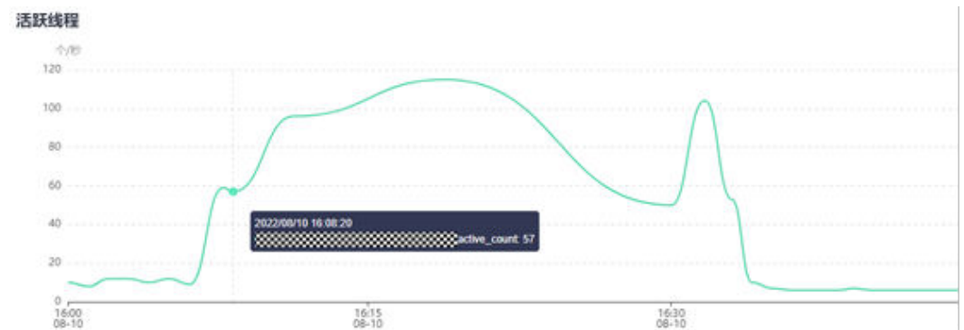
图 1-7 活跃连接数
