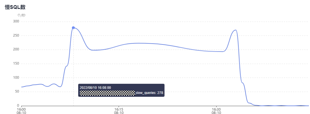
图 1-8 慢 SQL 数
