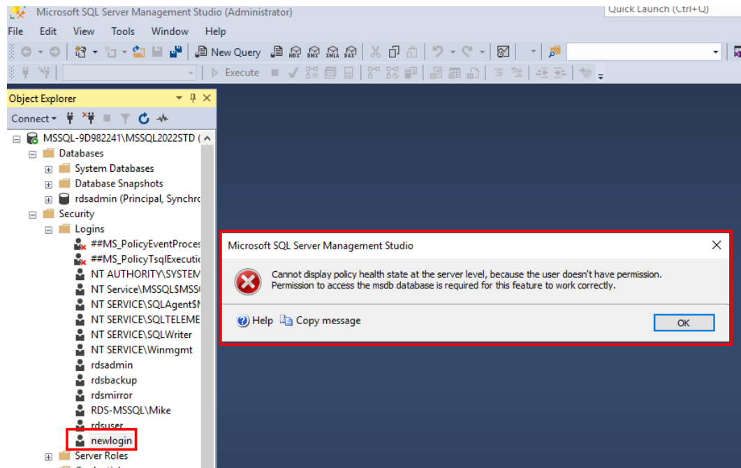
图 3-1 报错信息
