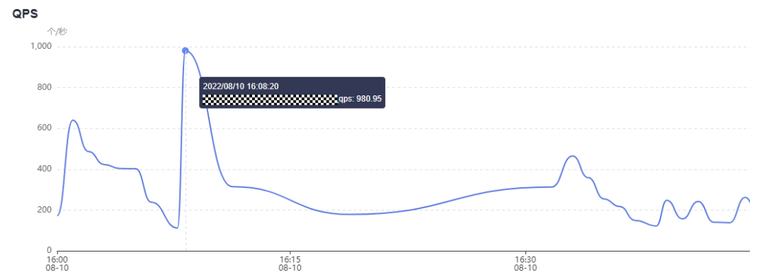
图 1-6 QPS
