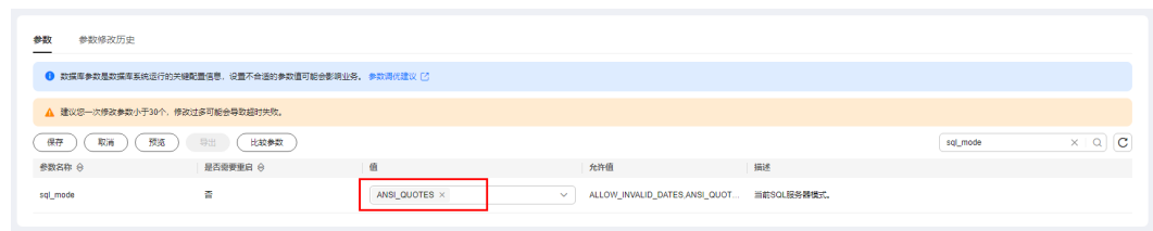
图 1-25 查看参数值
