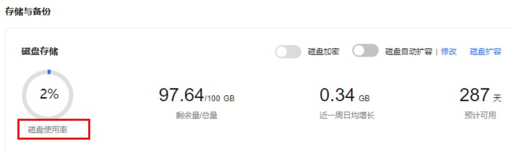
图 1-31 存储空间
