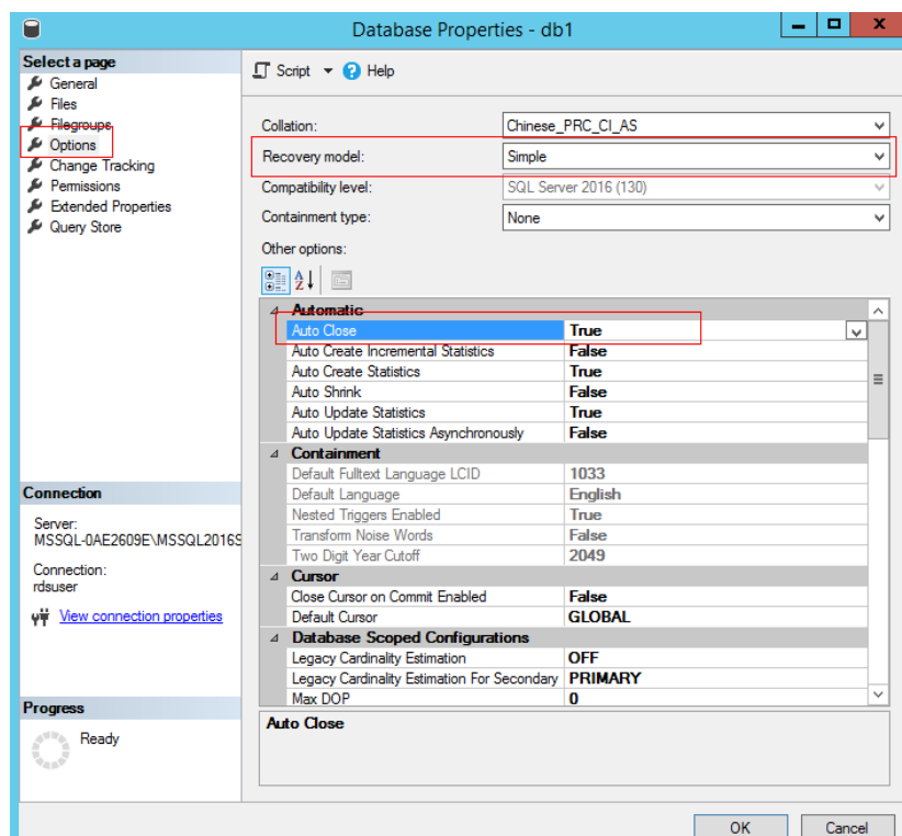
图 3-7 查看属性
