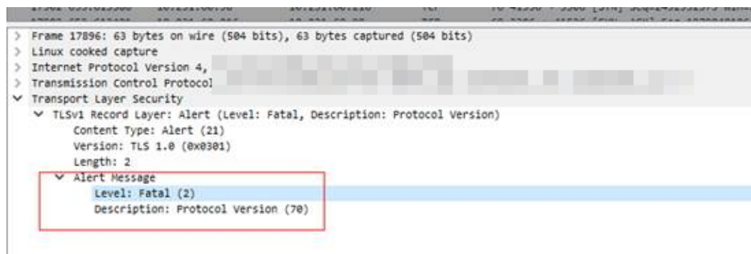
图 1-28 MySQL-server 的回复
