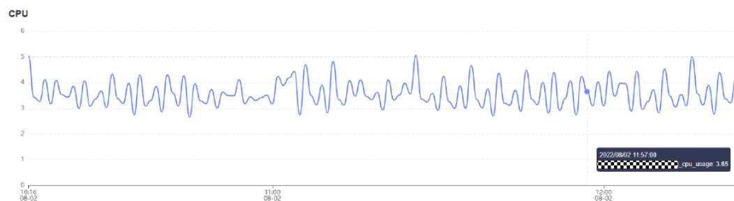
图 1-18 CPU 使用率
