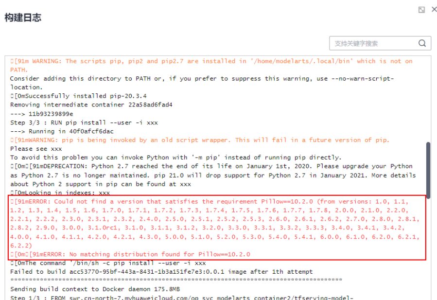
图 5-3 pip 版本不匹配
