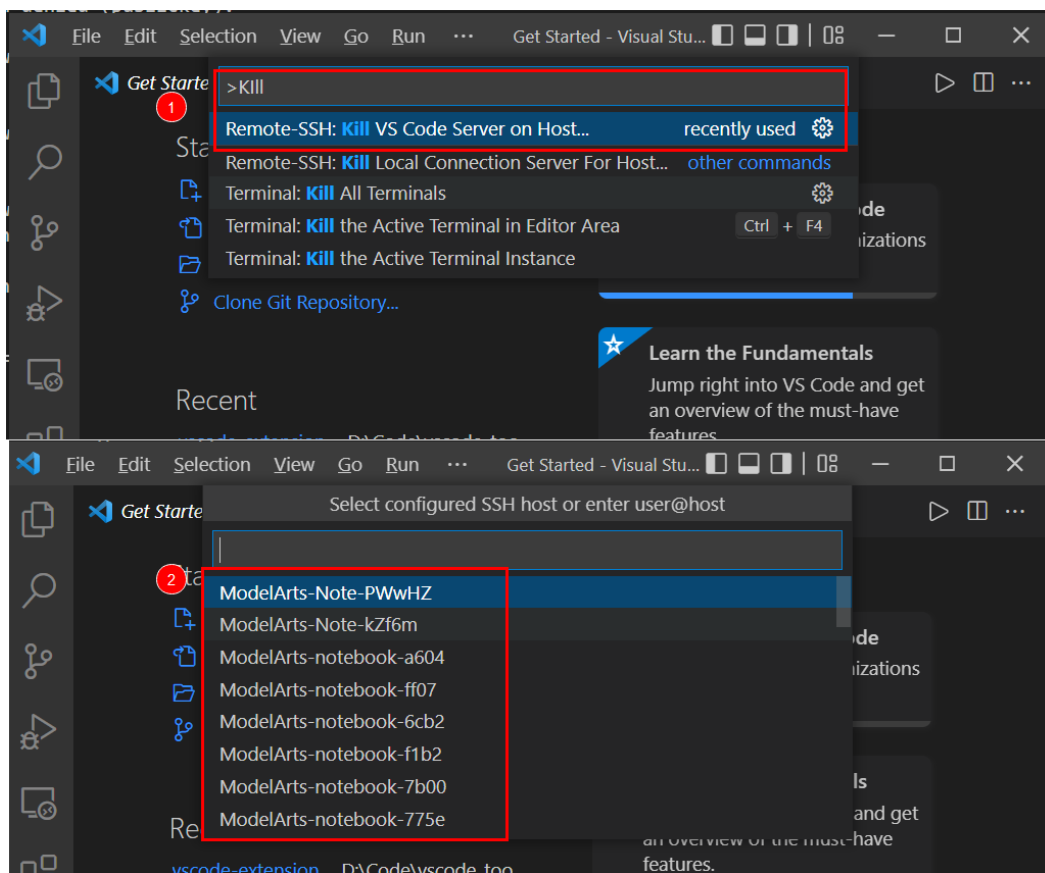
图 3-7 清除异常的实例
