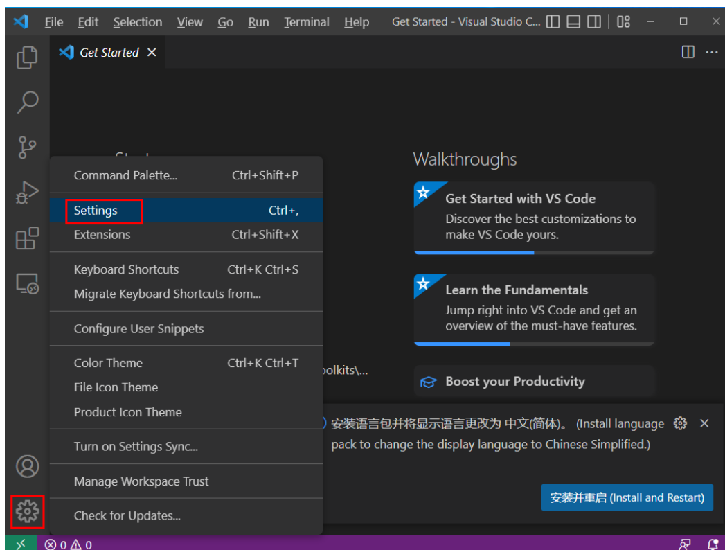
图 3-14 打开 Settings
