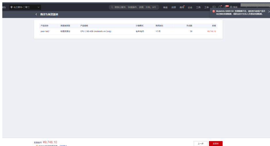
图 10-3 报错信息（1）
