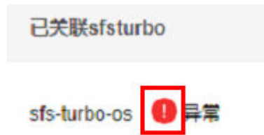
图 8-2 关联异常
