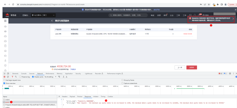
图 10-8 报错信息
