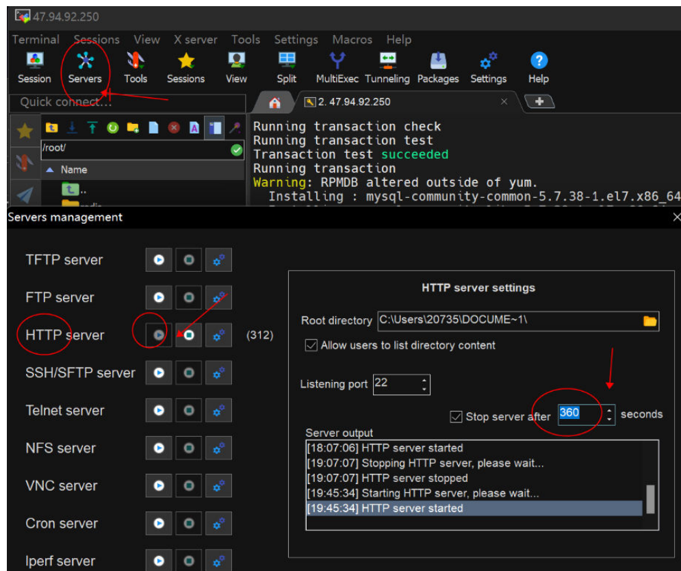
图 3-18 设置 “Stop server after”
