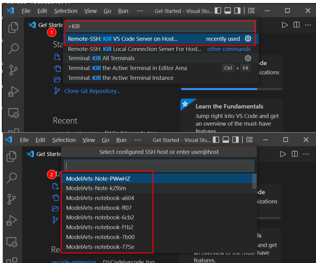
图 3-10 清除异常的实例
