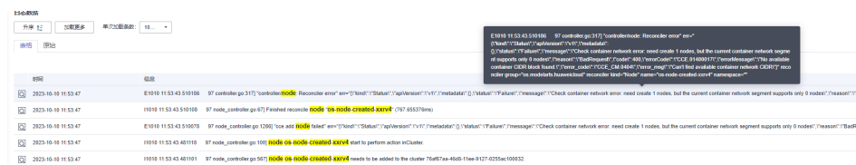
图 10-6 报错信息
