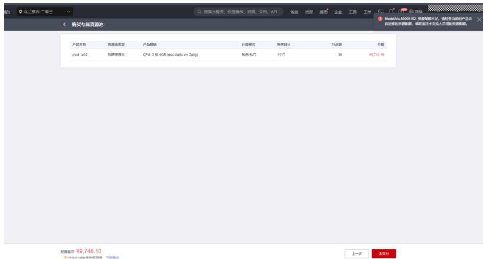
图 10-4 报错信息 (2)
