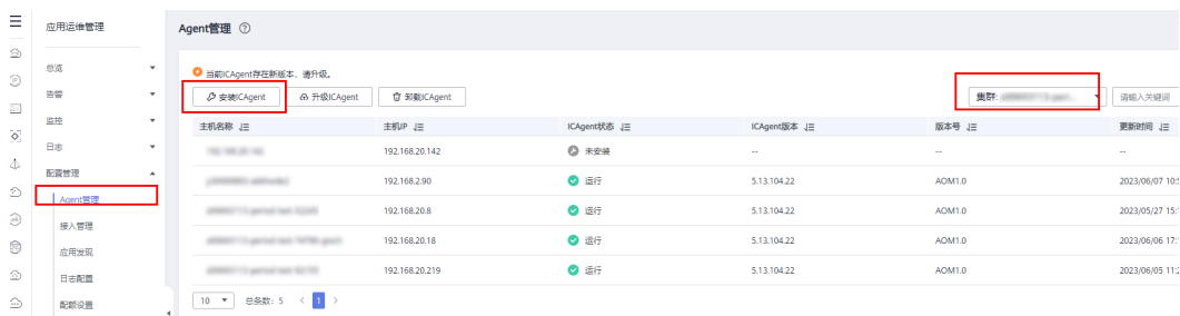
图 10-11 安装 ICAgent
