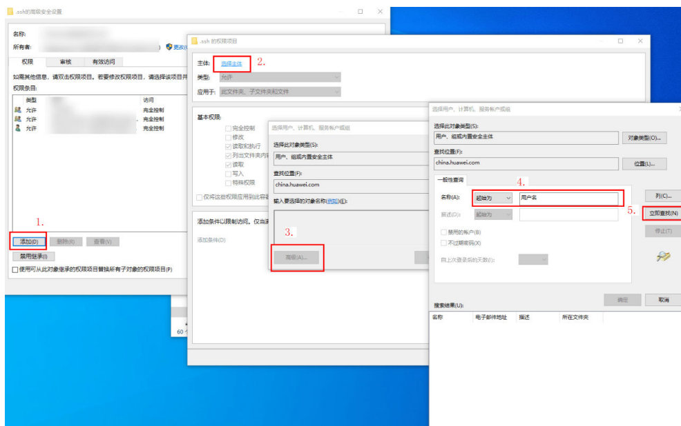
图 3-11 添加所有者
