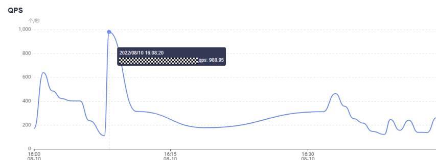
图 5-2 QPS
