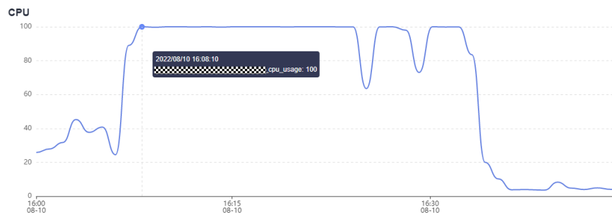
图 5-1 CPU 使用率
