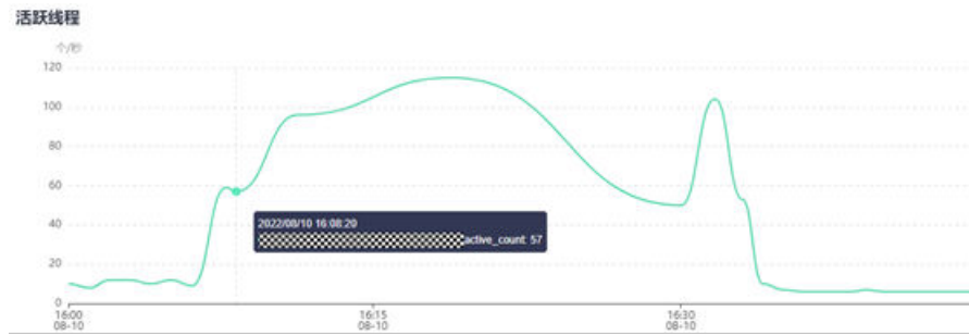
图 5-3 活跃连接数
