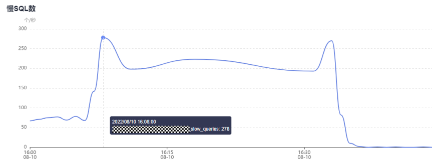
图 5-4 慢 SQL 数
