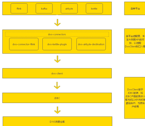
图 8-1 dws-client 交互场景
