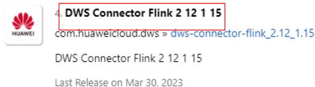
图 8-2 Flink 包
