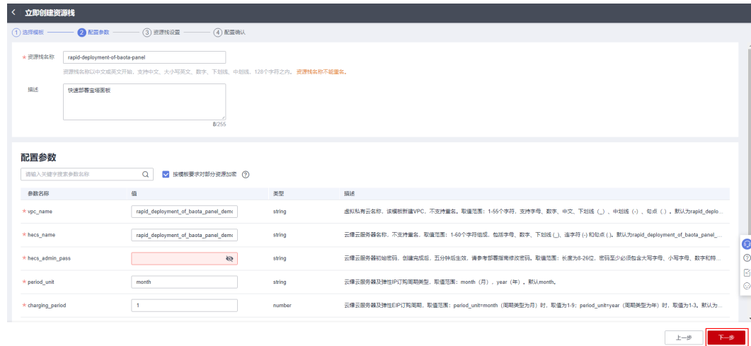
图 3-19 配置参数
