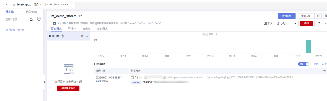
图 3-29 查看日志
