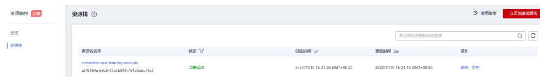
图 3-33 一键卸载
