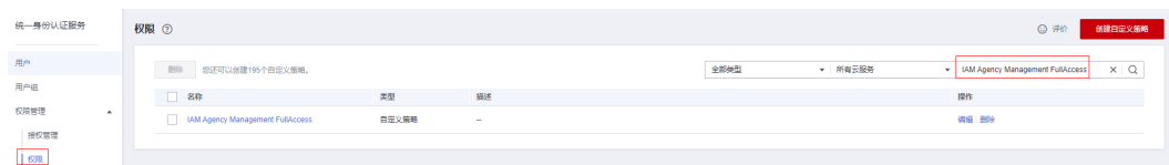
图 3-9 权限列表
