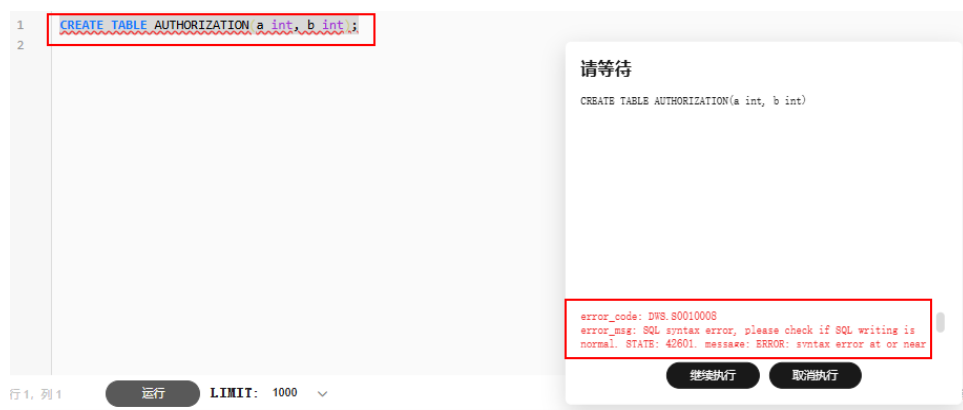
图 4-1 使用关键字作为表名
