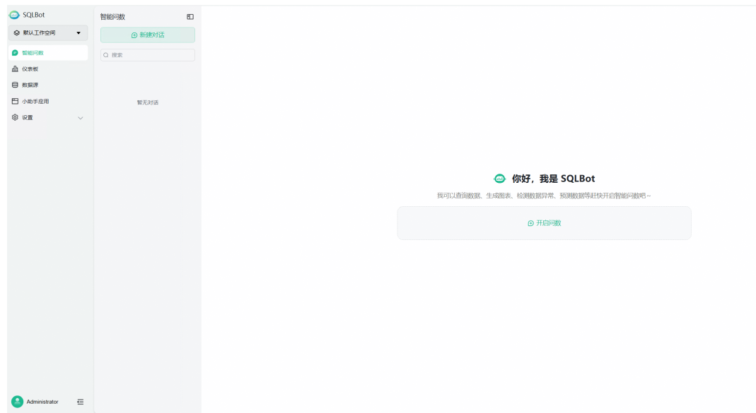
图 3-30 开启问数
