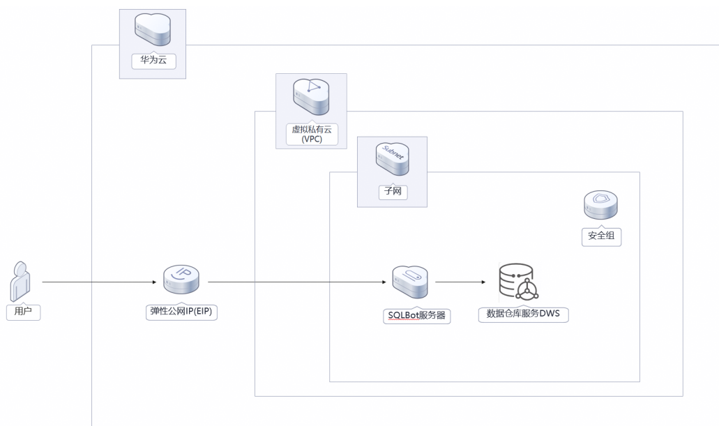
图 1-1 方案架构图
