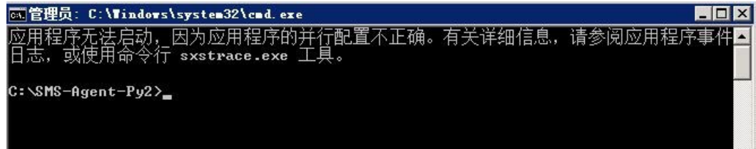
图 6-5 启动报错
