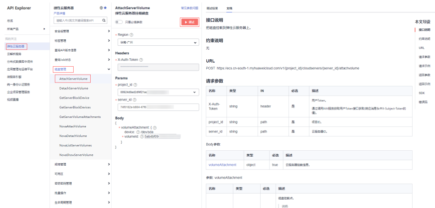
图 14-1 挂载磁盘
