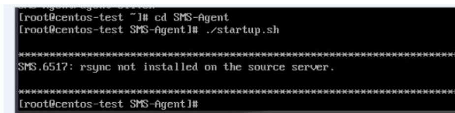
图 16-6 错误信息
