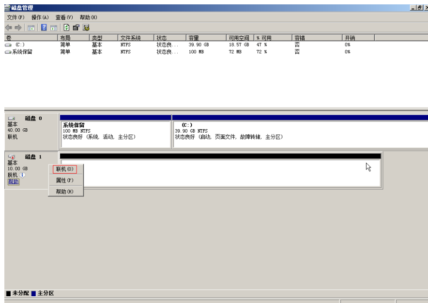
图 7-7 联机
