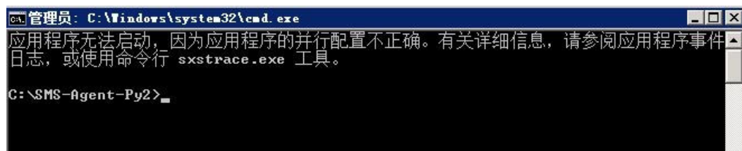
图 6-6 启动报错
