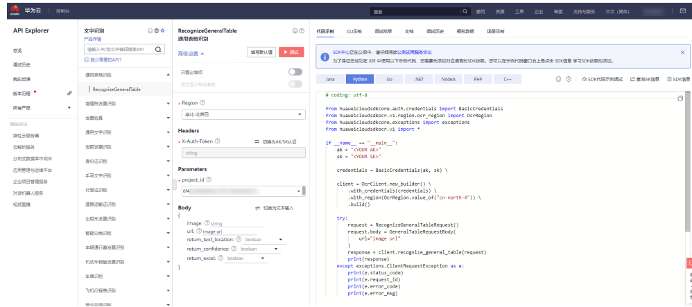
图 3-3 API Explorer
