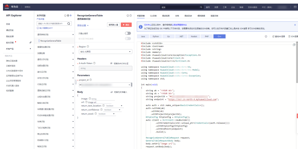
图 6-3 API Explorer
