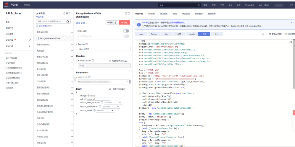
图 5-3 API Explorer
