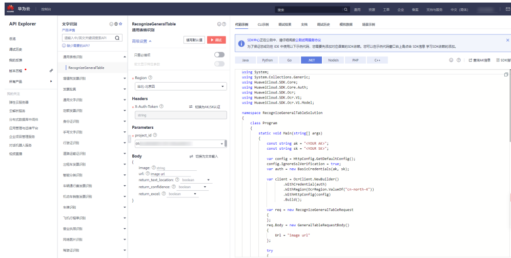
图 8-3 API Explorer
