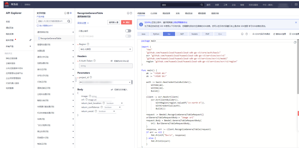
图 7-3 API Explorer
