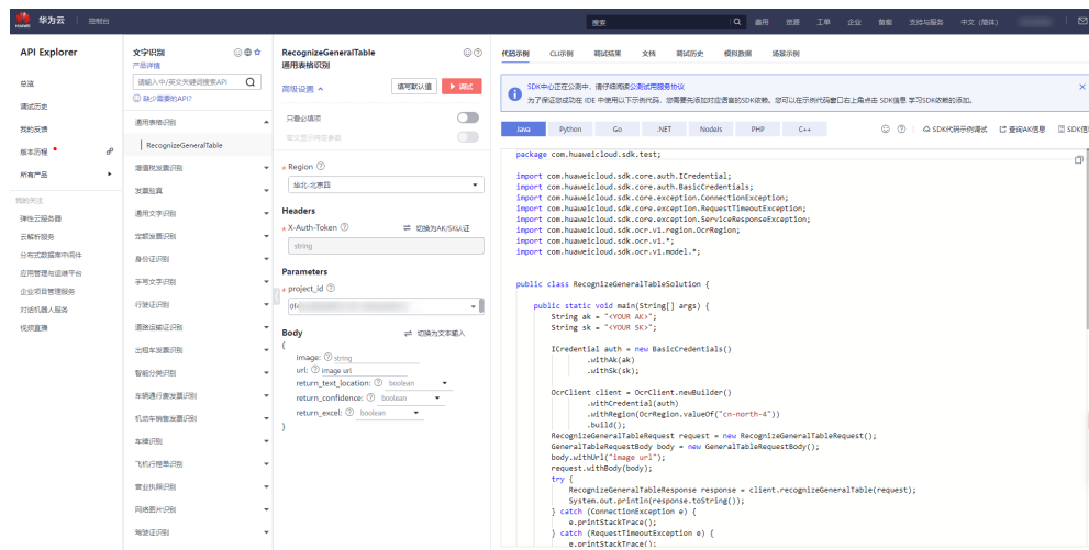
图 2-3 API Explorer
