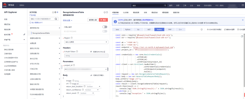
图 4-3 API Explorer
