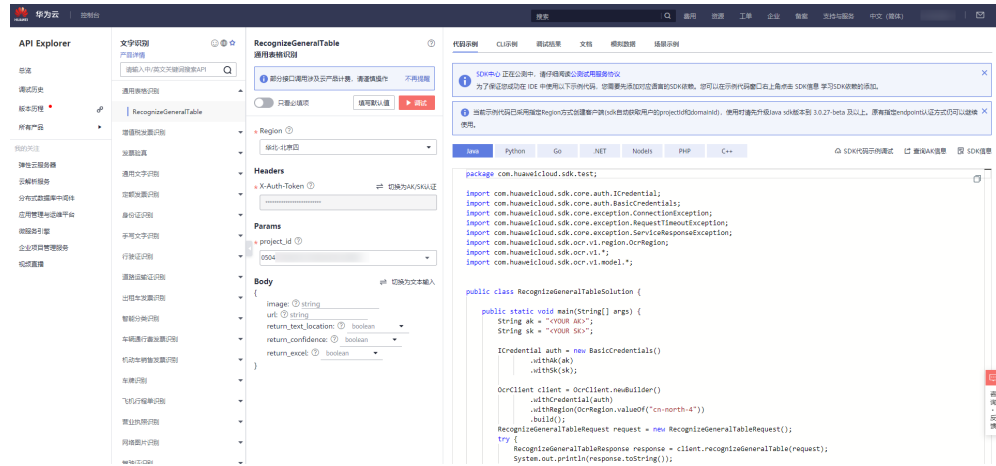
图 1-1 API Explorer
