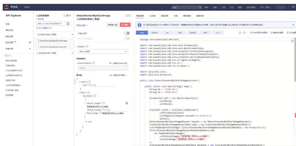
图 2-4 API Explorer
