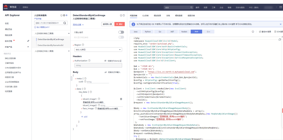
图 7-4 API Explorer
