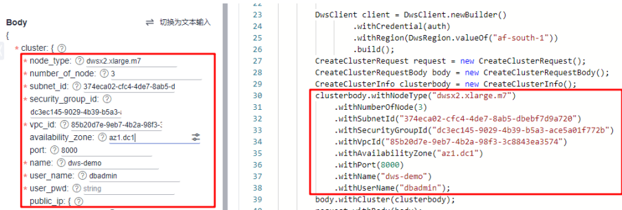
图 1-2 设置输入参数
