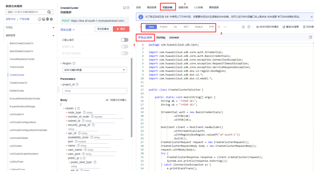
图 1-1 获取 SDK 代码示例
