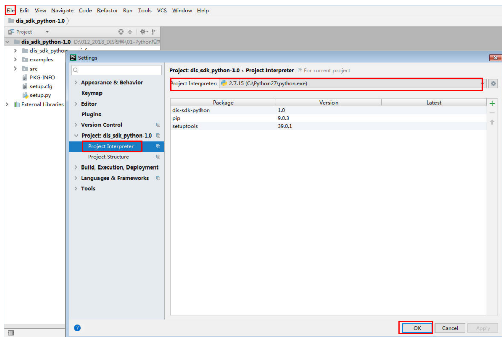
图 6-4 添加 python
