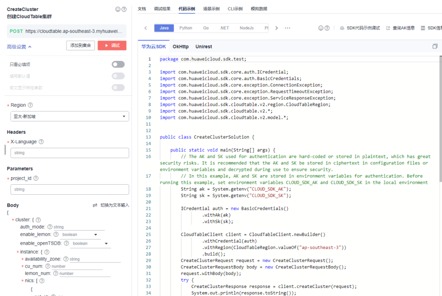
图 1-1 获取 SDK 代码示例
