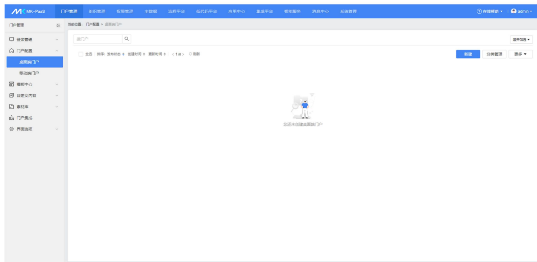
图 3-34 门户管理
