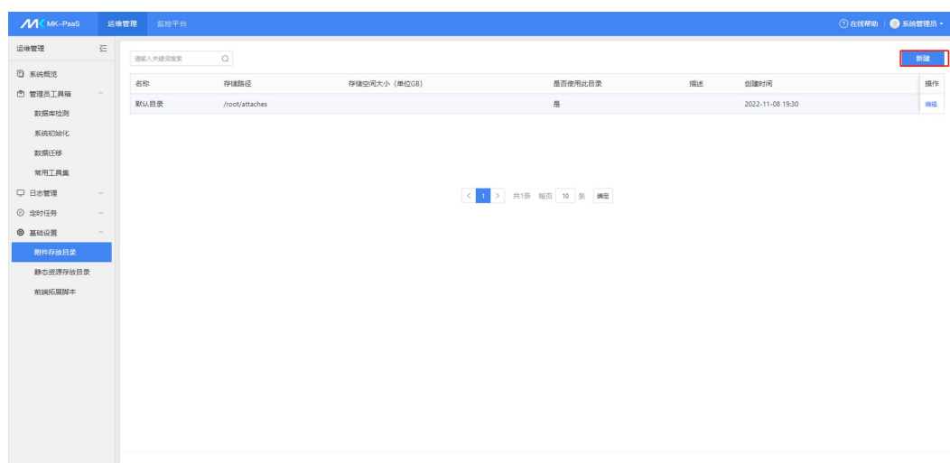
图 3-25 新建目录
