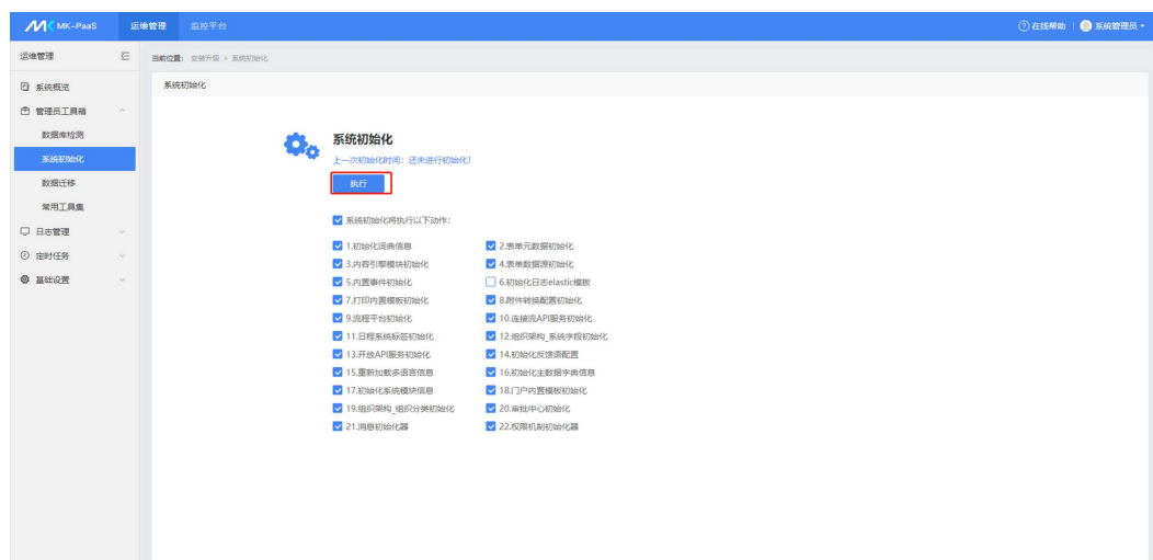
图 3-24 系统初始化
