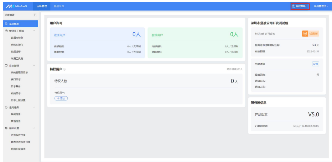
图 3-28 在线帮助
