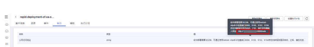
图 3-17 输出
