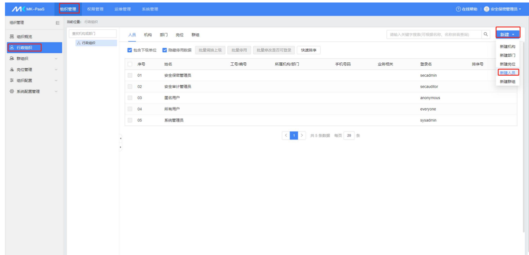
图 3-30 新建人员
