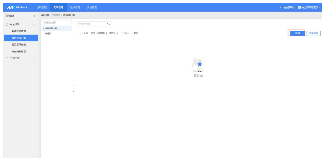
图 3-32 新建角色
