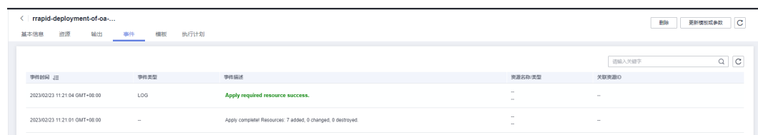
图 3-16 部署成功
