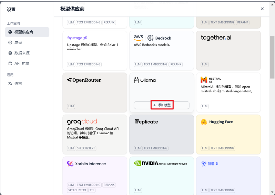
图 3-19 添加模型
