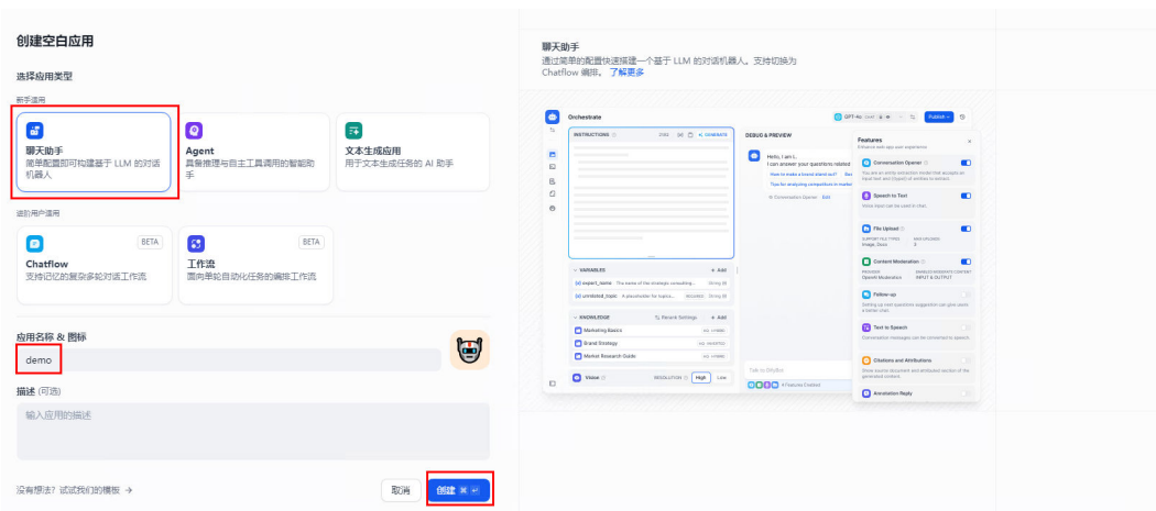
图 3-22 创建应用
