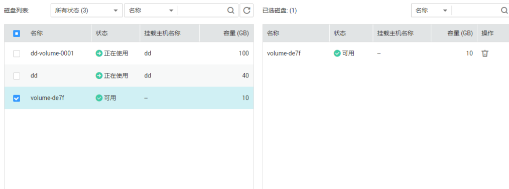
图 2-3 选择磁盘
