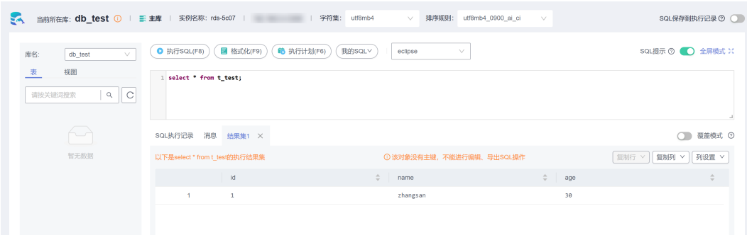
图 1-13 查询数据
