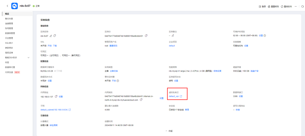
图 2-6 MySQL 概览
