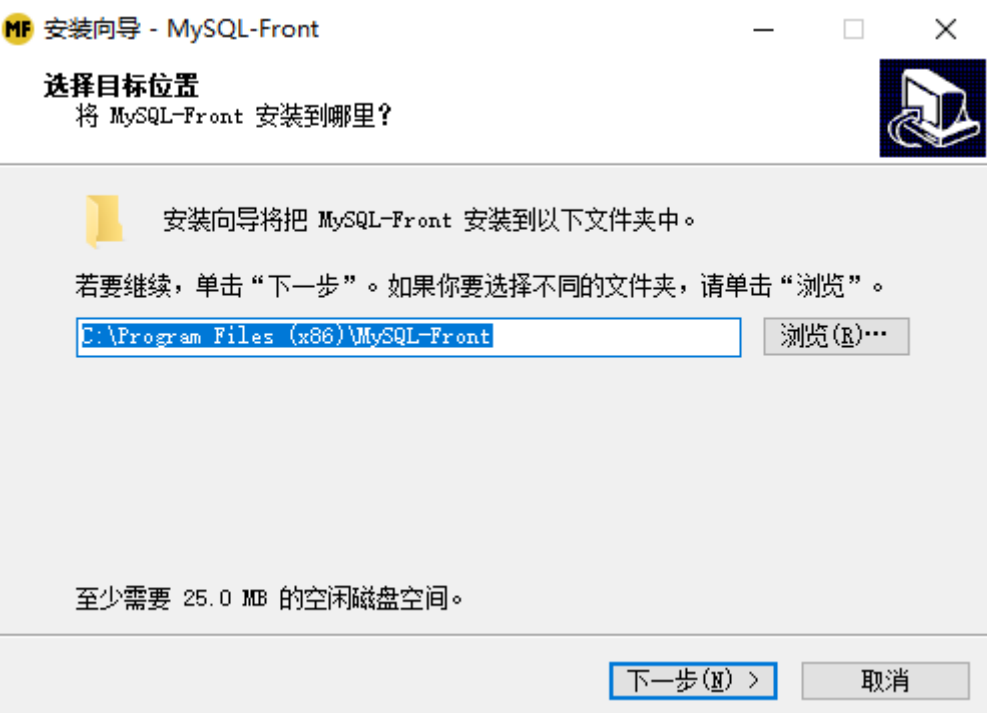
图 3-9 选择位置
