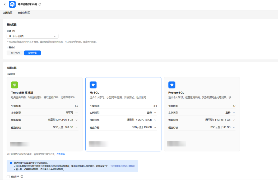
图 1-1 基础配置
