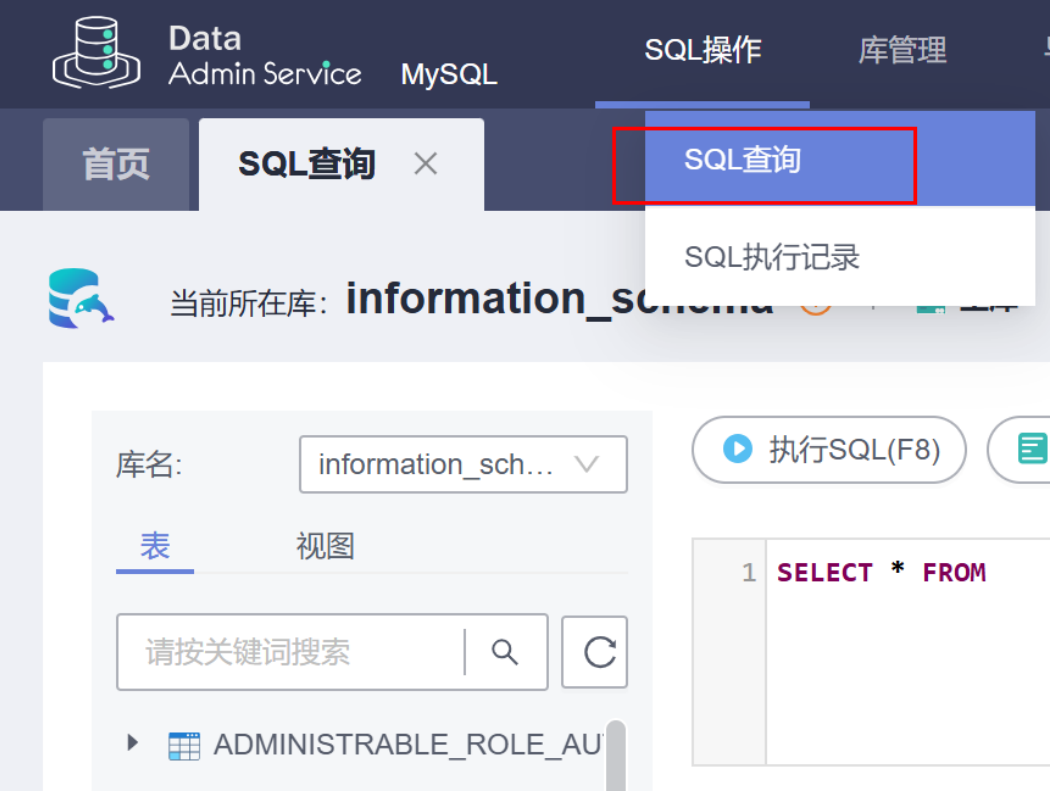
图 1-8 SQL 查询
