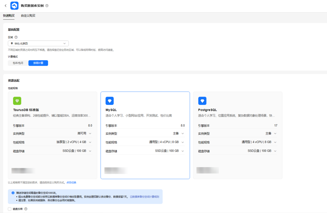
图 2-1 基础配置
