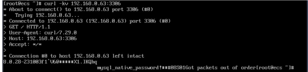
图 2-8 网络正常
