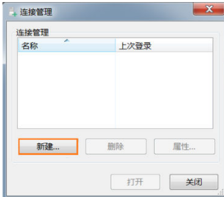
图 3-13 连接管理
