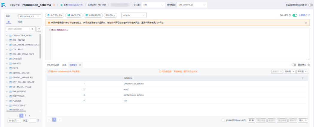
图 1-9 查询数据库
