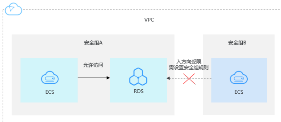
图 4-1 连接示意图
