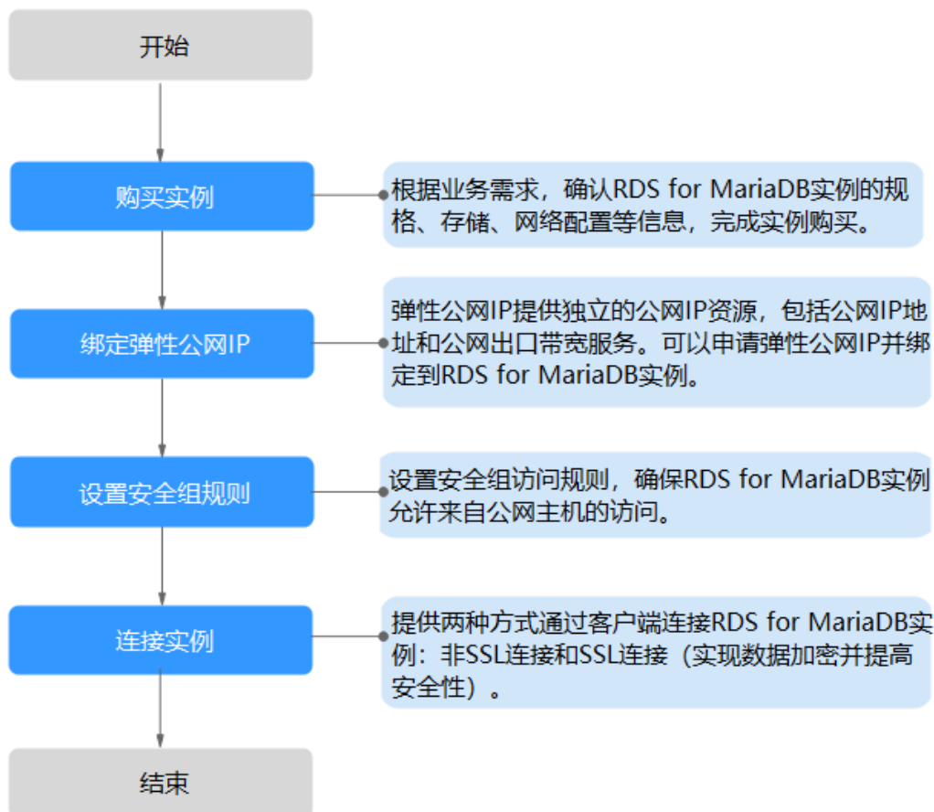
图 3-6 通过公网连接实例
