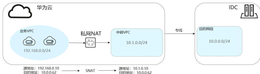
图 3-1 组网图
