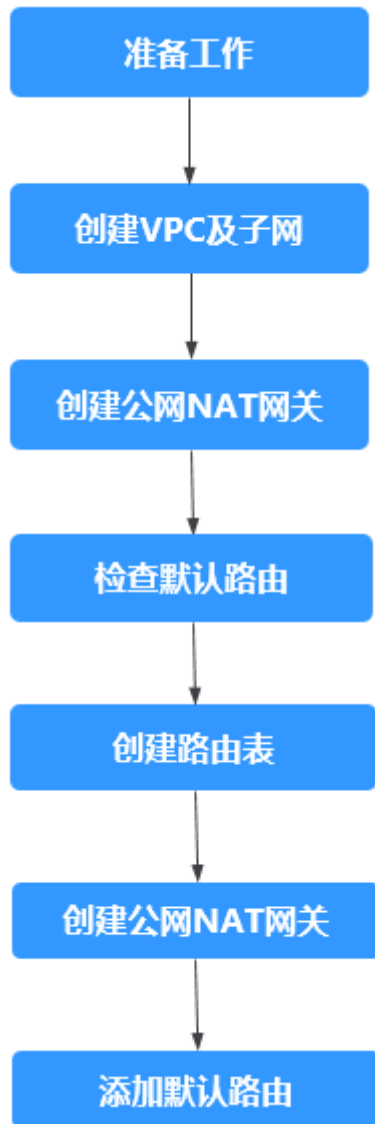
图 4-1 入门流程
